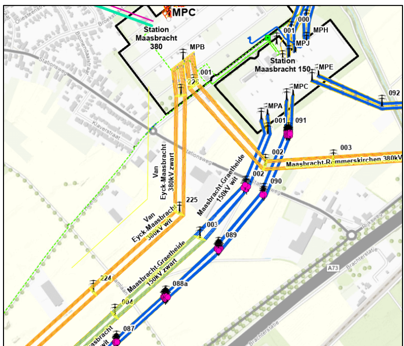
Figuur 1: huidige situatie aanlanding van de 380 kV-verbindingen (gele lijnen) en de 150 kV-verbindingen (blauwe lijnen) op station Maasbracht
