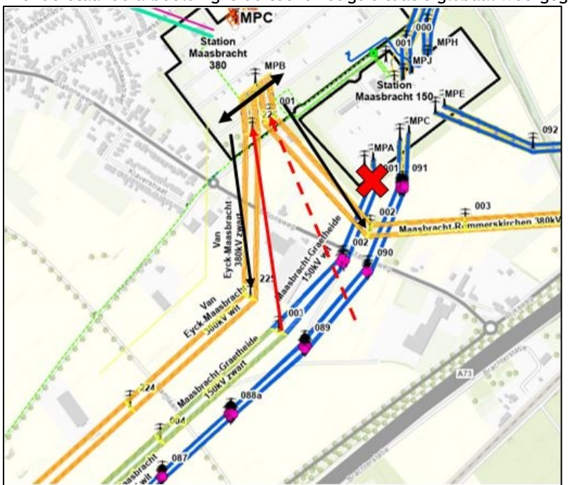
Figuur 2: globale weergave toekomstige situatie met de aangepaste situatie van de bestaande 380 kV-verbindingen (zwarte pijlen), en de aansluiting van de opgewaardeerde (rode pijl) en toekomstige 380 kV-verbindingen (rode pijl stippellijn).
