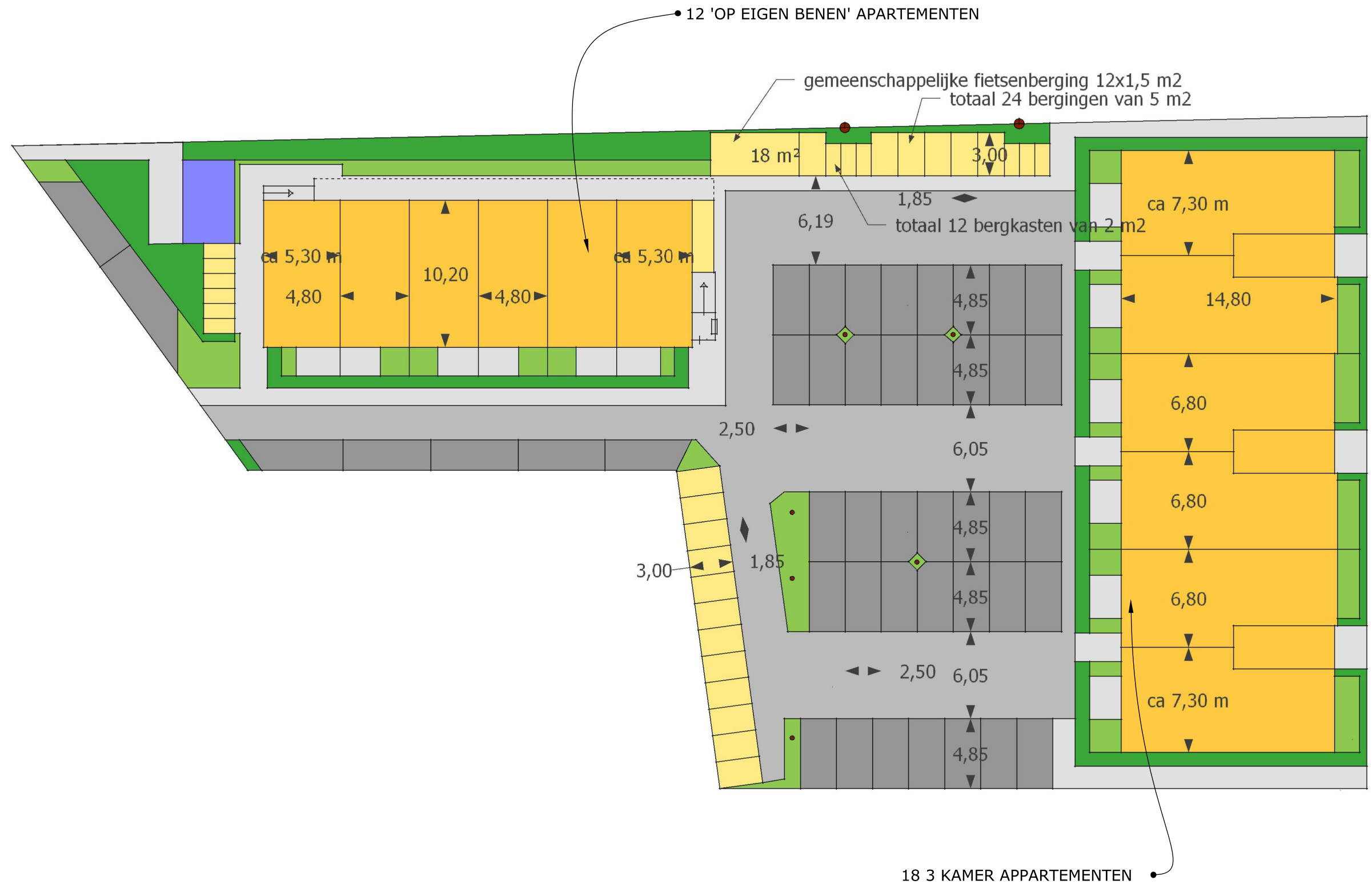
MATENPLAN. SCHAAAL 1:300
