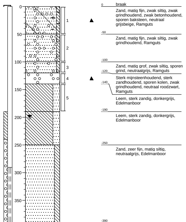
Boring: 004 Datum: 17-08-2016
