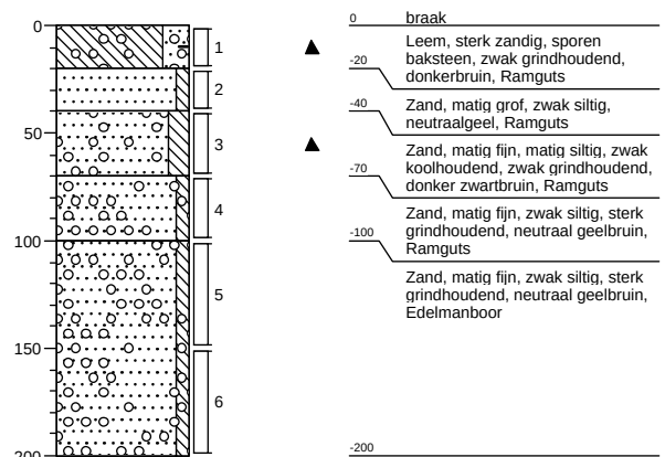
Boring: 102 Datum: 23-09-2016
