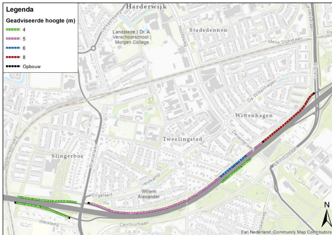
Overzichtstekening Geluidsscherm Meerjarenprogramma Geluidsanering en Vervanging en Renovatie
