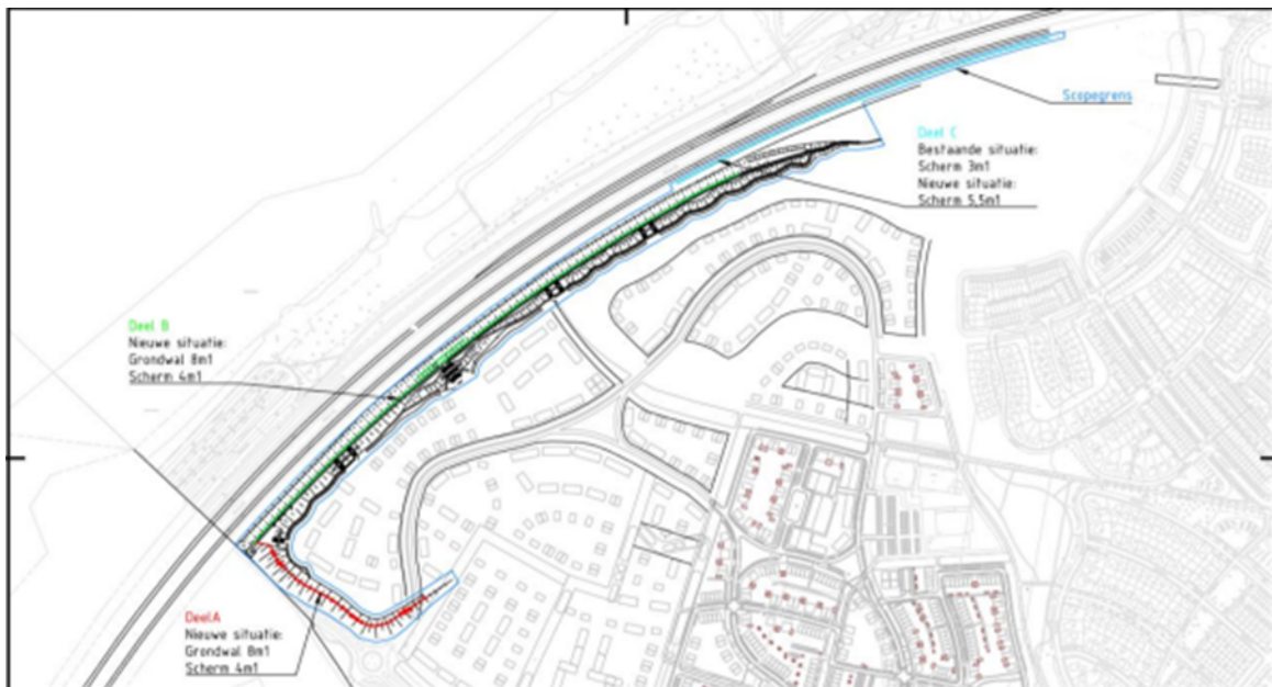
Overzichtstekening Geluidsscherm Harderweide
