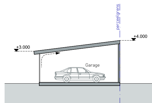
T2 - principesnede garage
