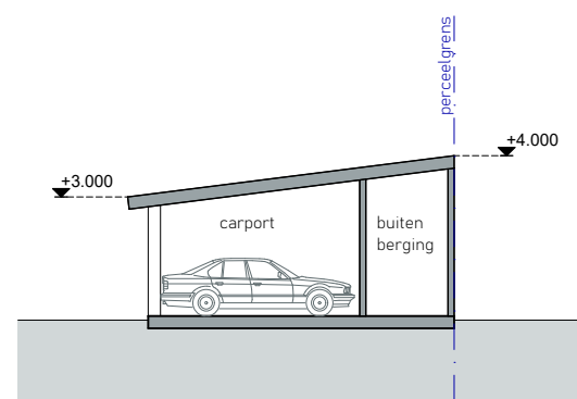
T1 - principesnede carport
