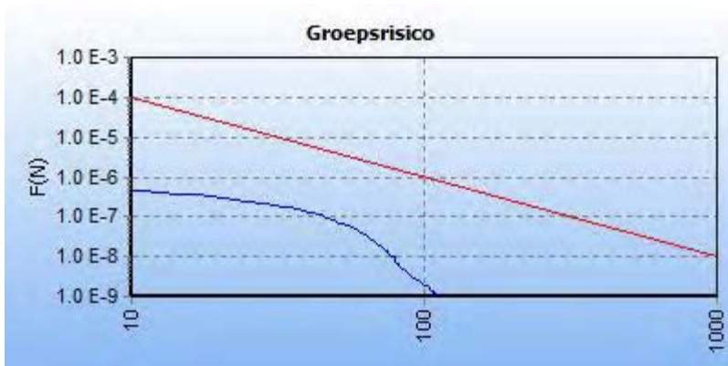
5.2 Figuur 5.2 FN curve voor 7924_leiding-N-570-20-deel-1 van N.V. Nederlandse Gasunie voor de kilometer tussen stationing 2190.00 en stationing 3190.00
