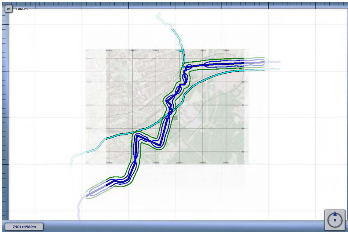
3.2 Figuur 3.2 Plaatsgebonden risico voor 7924_leiding-N-570-20-deel-1 van N.V. Nederlandse Gasunie
