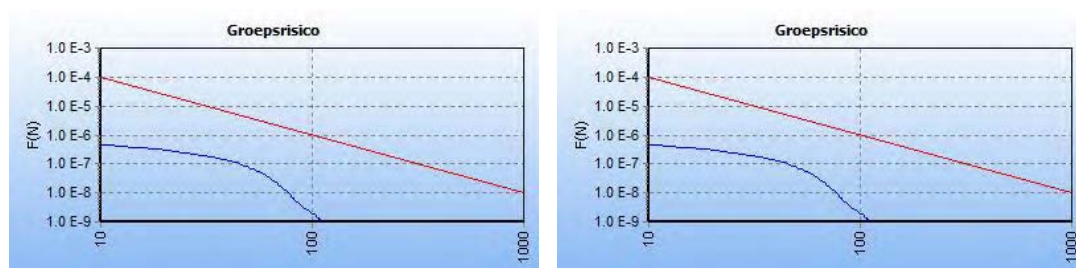
Figuur 7. Groepsrisico N-570-20, huidig (links) en toekomstig (rechts)
