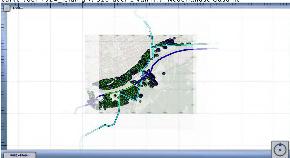
Figuur 4.2 Kilometer leiding behorende bij de maximale overschrijding van de FN-curve voor 7924 leiding-A-510-deel-1 van N.V. Nederlandse Gasunie
