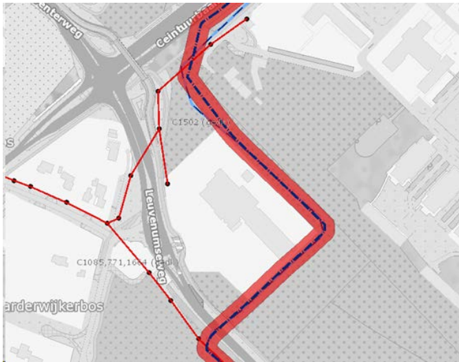
Afbeelding 4.2 perstransportleiding
