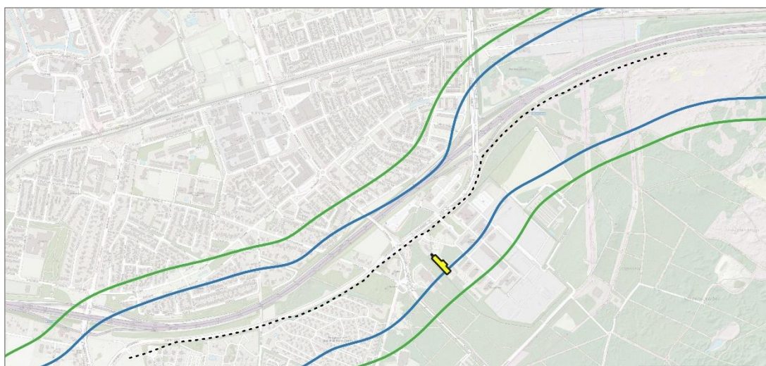
Figuur 4. Plaatsgebonden risicocontouren aardgasbuisleiding A-510
