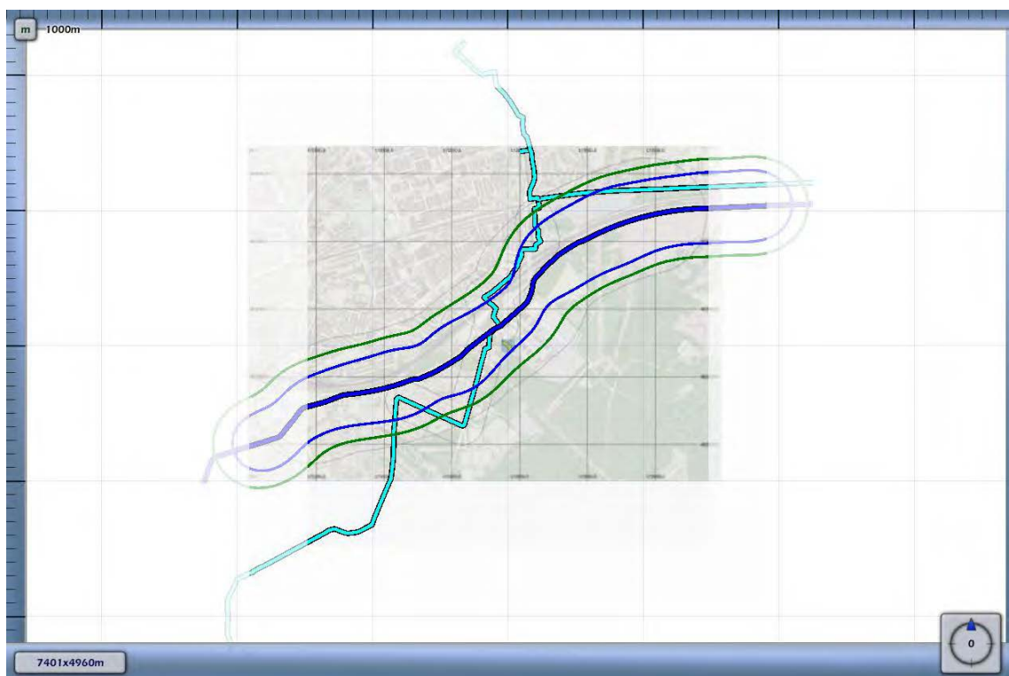
3.1 Figuur 3.1 Plaatsgebonden risico voor 7924_leiding-A-510-deel-1 van N.V. Nederlandse Gasunie
