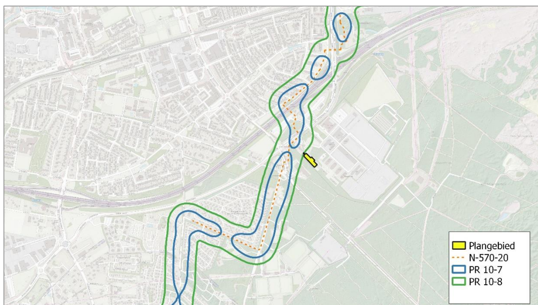
Figuur 5. Plaatsgebonden risicocontouren aardgasbuisleiding N-570-20
