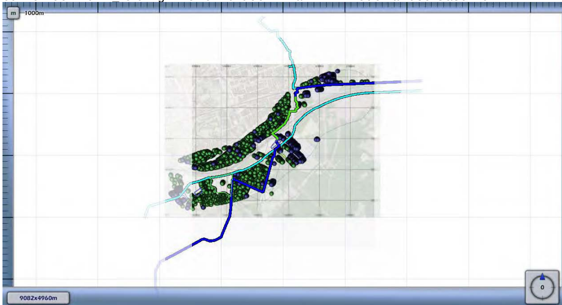
Figuur 4.4 Kilometer leiding behorende bij de maximale overschrijding van de FN-curve voor 7924 leiding-N-570-20-deel-1 van N.V. Nederlandse Gasunie
