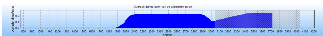
4.1 Figuur 4.1 Groepsrisico screening voor 7924_leiding-A-510-deel-1 van N.V. Nederlandse Gasunie
