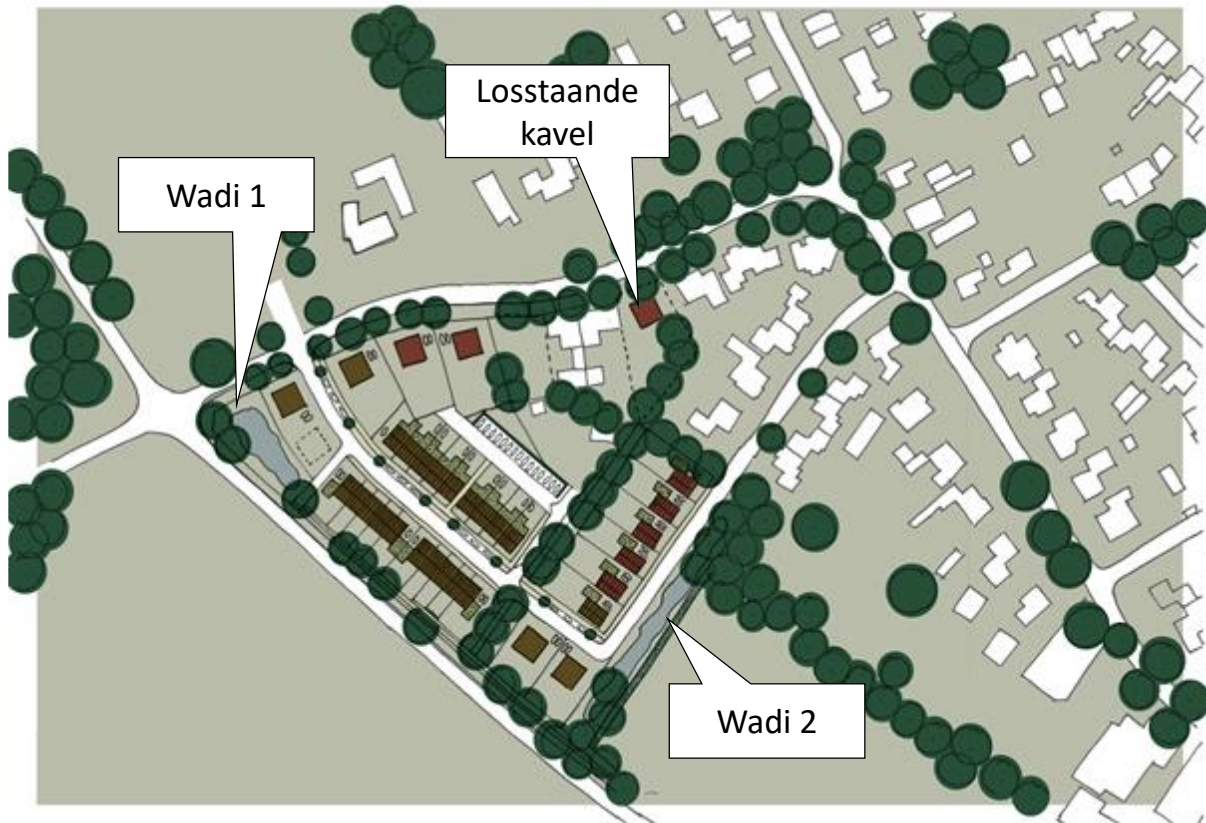
figuur 3 Stedenbouwkundig plan met wadi's
