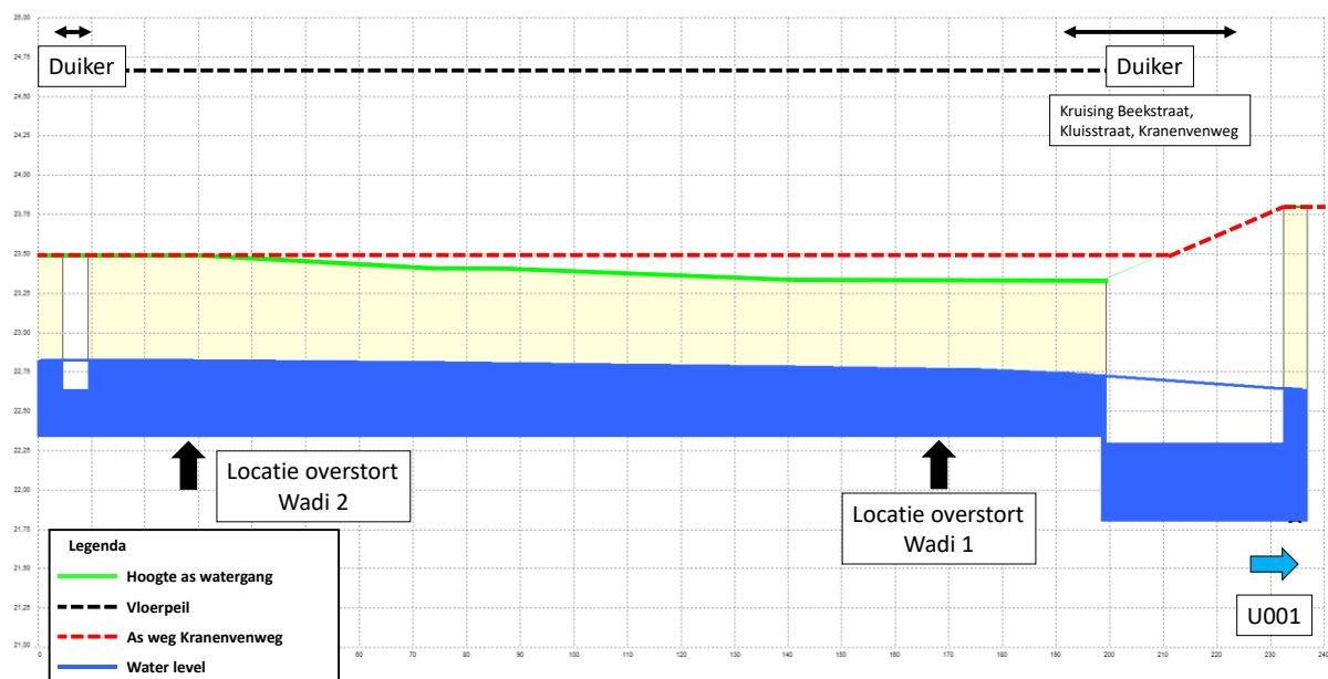
figuur 10 Verloop maximale spiegelverhanglijn tijdens stresstestbui 03
