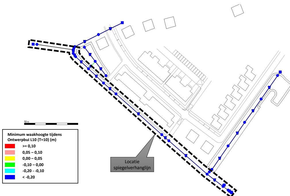
figuur 6 Minimum waakhoogte in HWA stelsel tijdens ontwerpui L10 (T=10)
