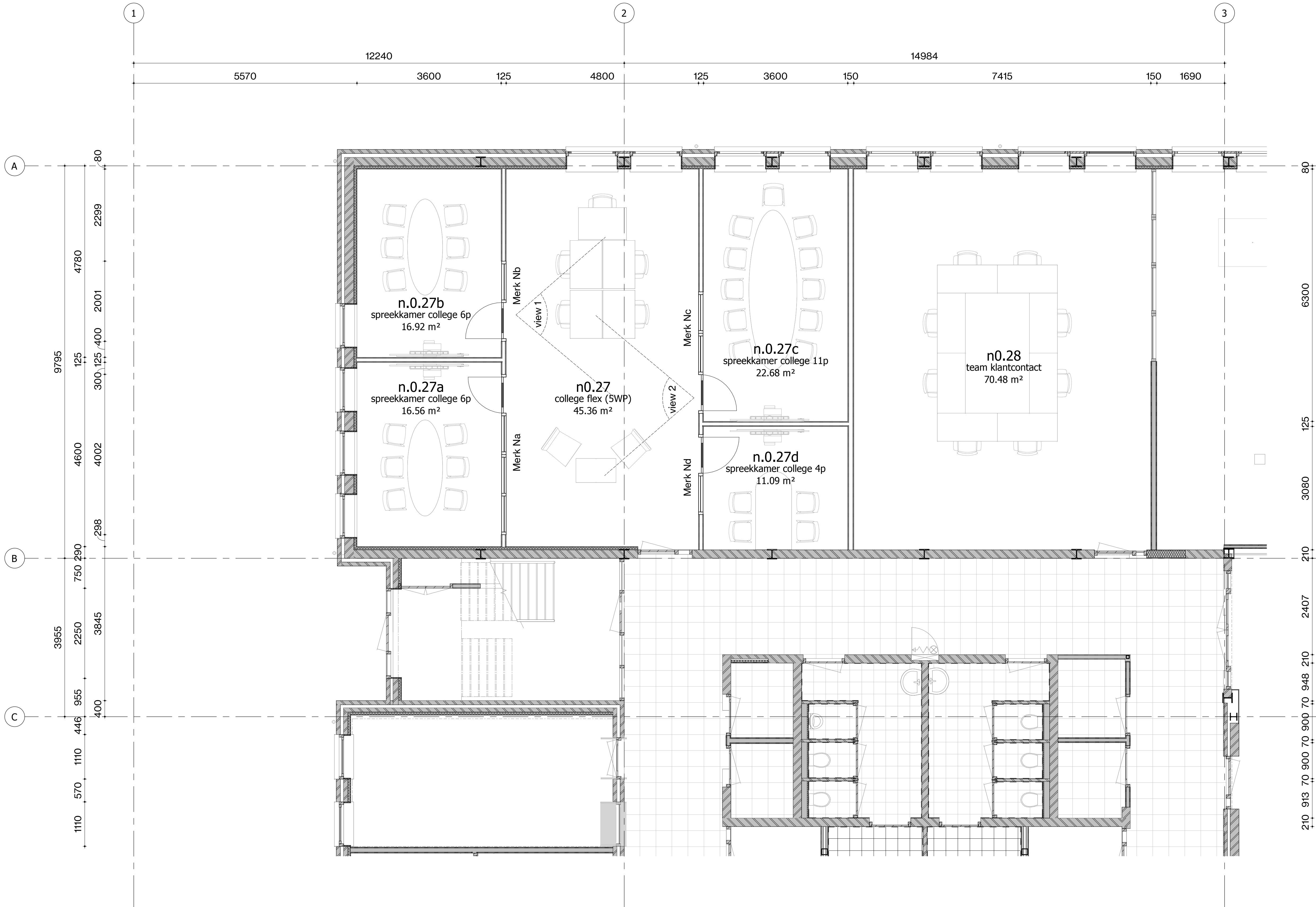
Begane grond
