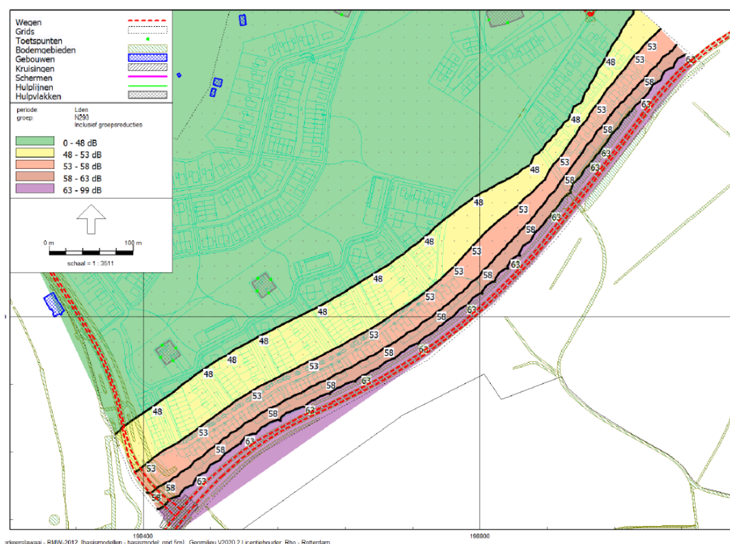
Afbeelding 4.13: vrije veldcontouren N293 - op 3 en 5 meter hoogte
