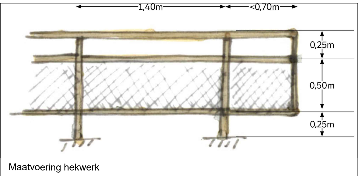
Maatvoering hekwerk
