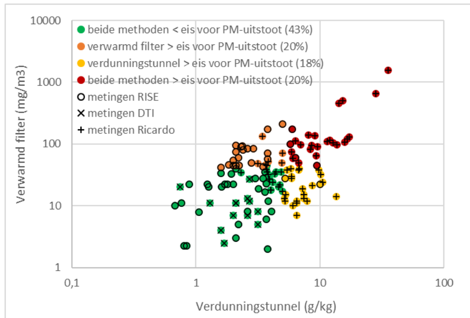
Figuur 4. Correlatie tussen de verwarmd filter methode en de verduunningstunnel methode op basis van 2 datasets: RISE (EN-PME methode met verwarmd filter bij 180 °C, zwart omcirkeld) en Ricardo (DINplus methode met verwarmd filter bij 70°C), waarbij de data is vergeleken met de eis voor PM-uitstoot (respectievelijk 40 mg/m 3 en 5 g/kg). De percentages geven het deel van de metingen aan dat binnen dit criterium valt.
