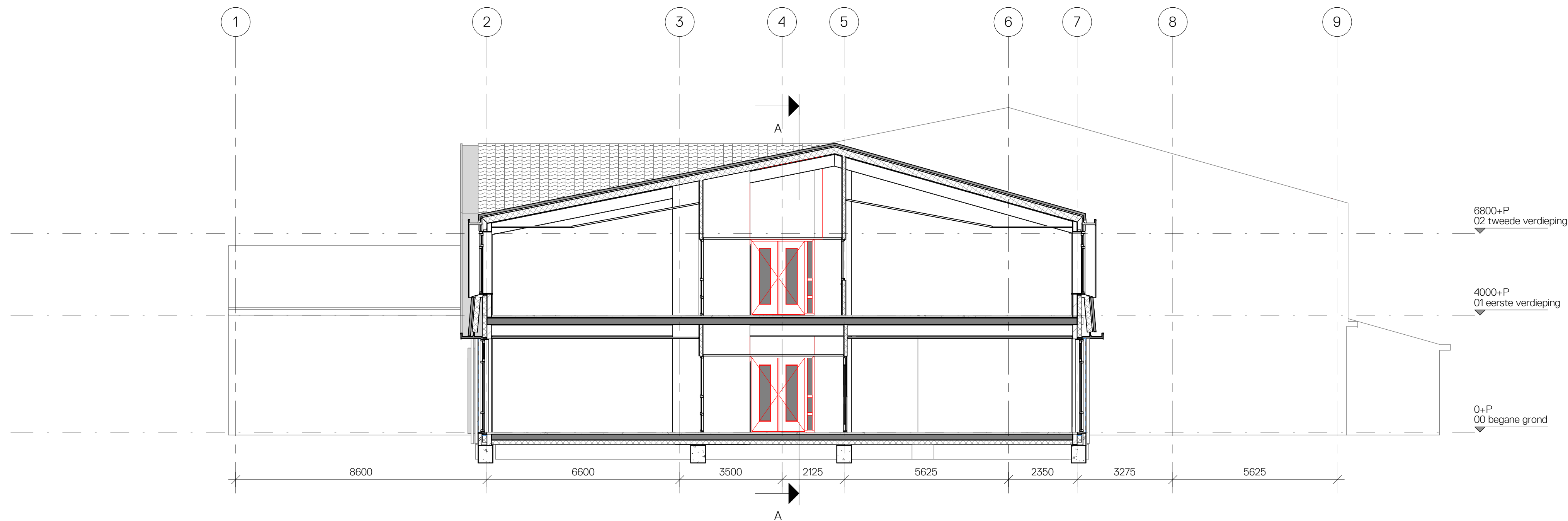
2 Doorsnede B 1:100
