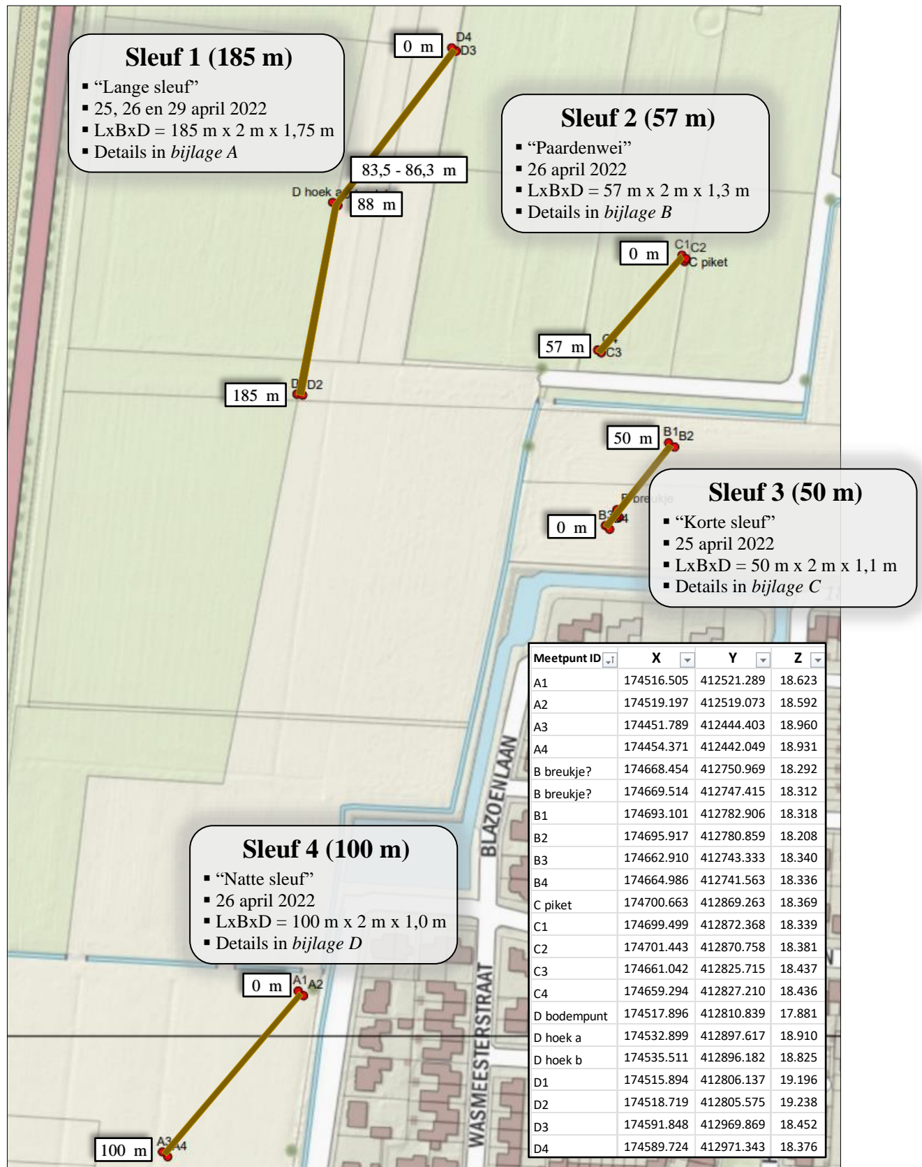
Figuur 3 Situering en karakteristieken van de 4 sleuven ter plaatse van ontwikkellocatie Repelakker III. In het kader staan de ingemeten coördinaten en NAP-hoogtes.
