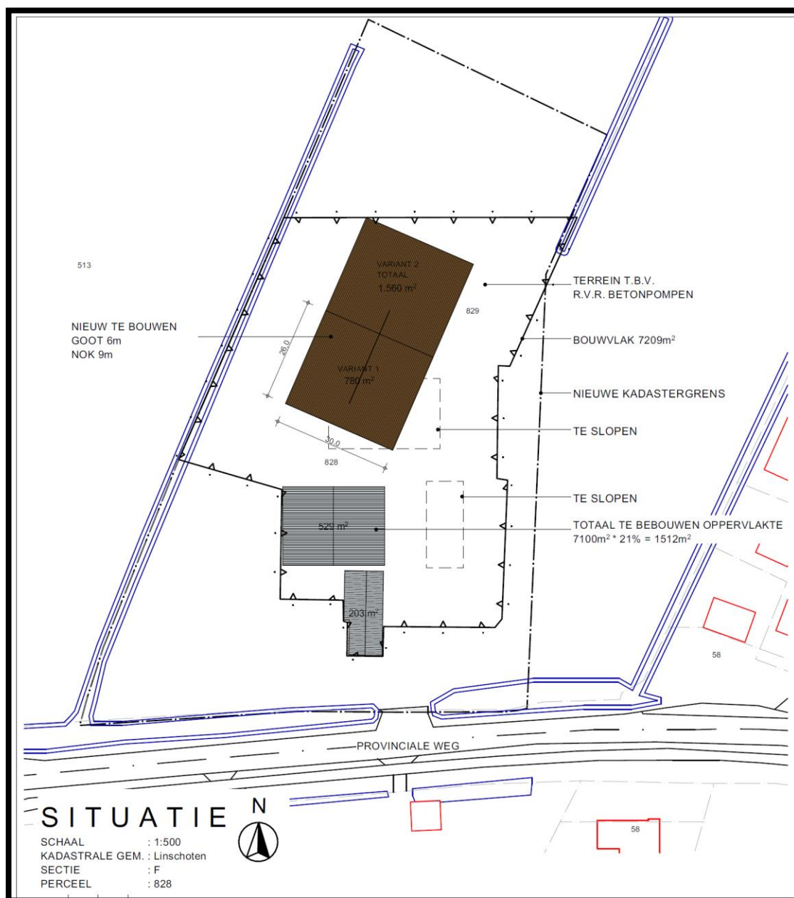
Figuur 1: Overzicht van de oude situatie en de nieuwe kadastrale grenzen van de inrichting.
