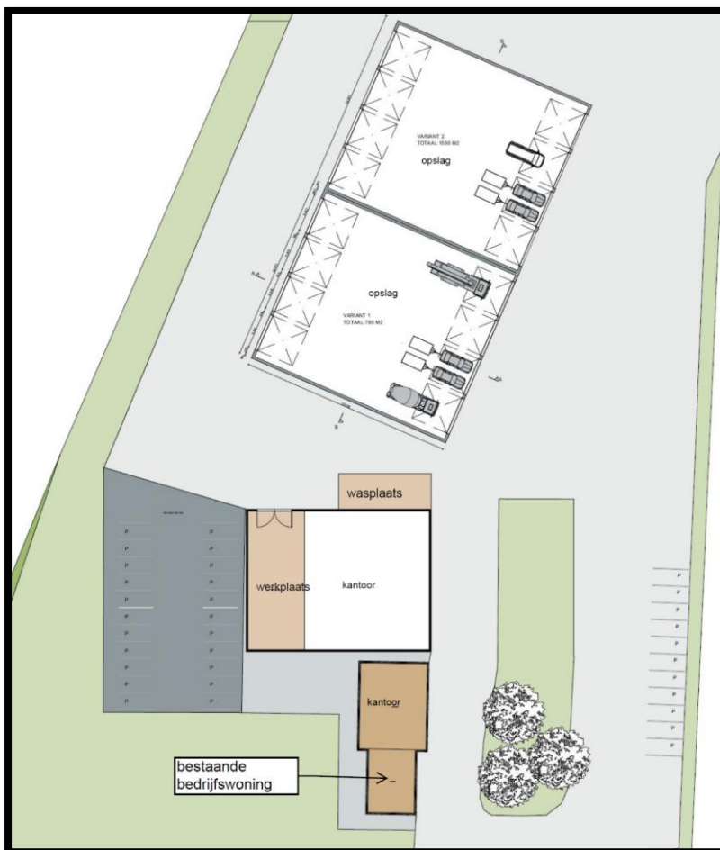
Figuur 2: Nieuwe indeling van het bedrijf.
