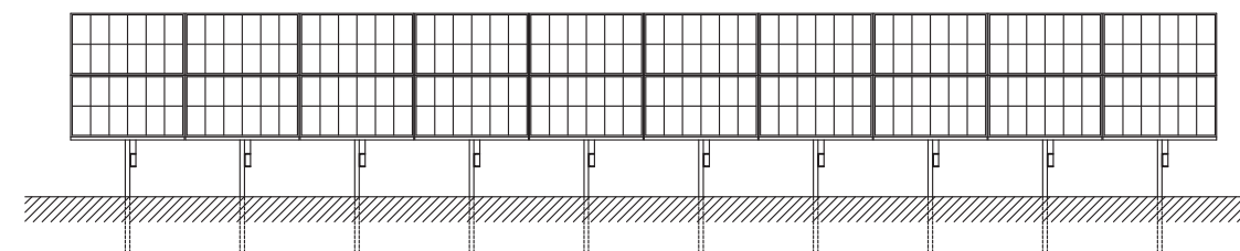
Vooraanzicht zonnepaneel (2 panelen)/ Front view solar panel (2 panels)
