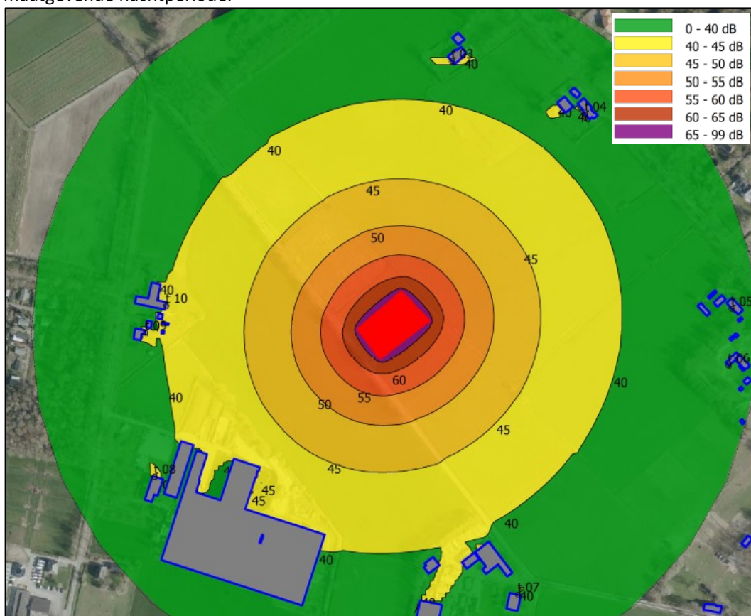
Figuur 2. Geluidcontouren nachtperiode 5,0 meter hoogte incl. 5 dB toeslag.
