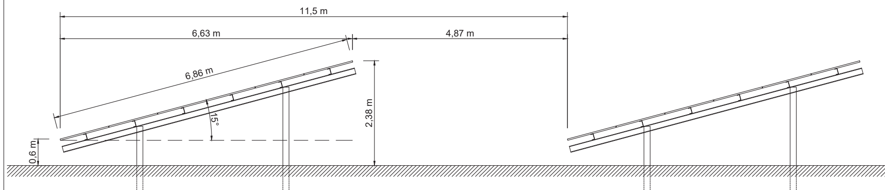
Zijaanzicht zonnepanelen (6 panelen)/ Side view solar panels (6 panels)
