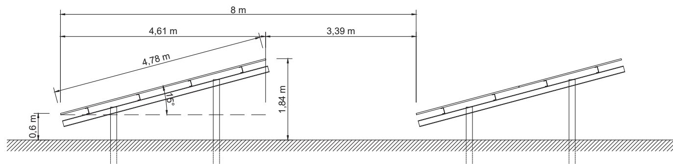
Zijaanzicht zonnepanelen (2 panelen)/ Side view solar panels (2 panels)
