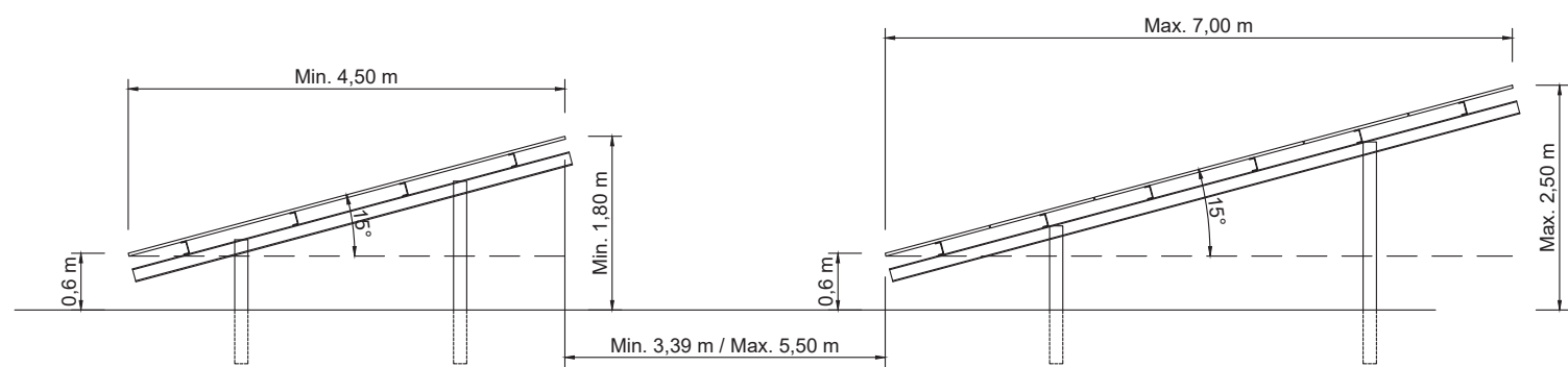
Bandbreedte constructie zonnepark/ Construction bandwidth solar farm
