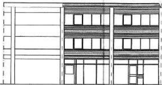
voorgevel
