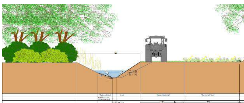
Figuur 11: Basisprofiel 'eénzijdig profiel binnen bestaande beek'
