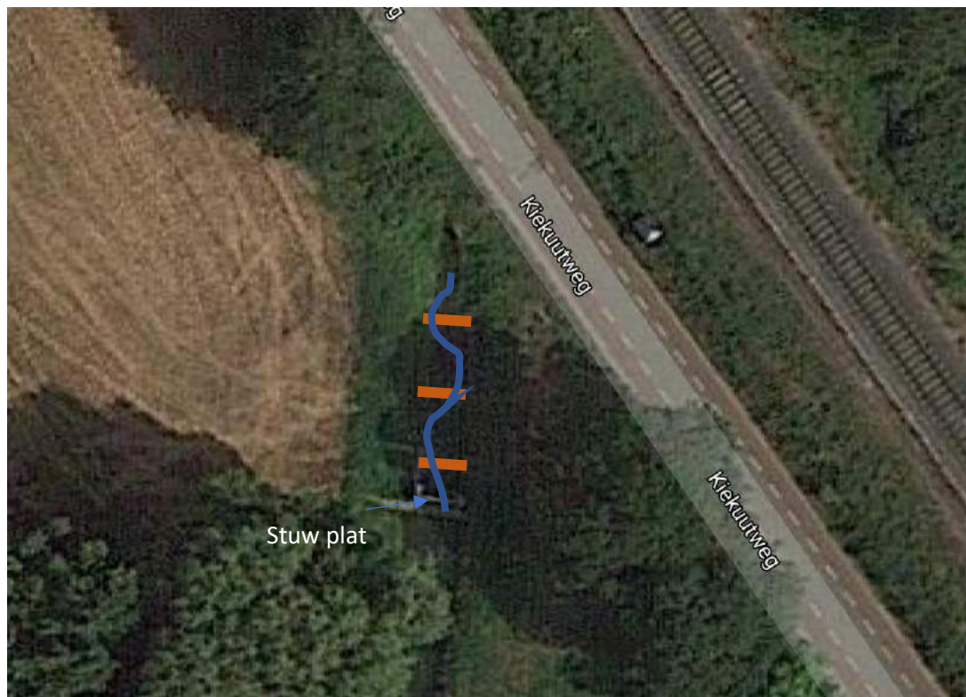
Figuur 9.2. Principeschets van een vispassage benedenstrooms van de stuw
