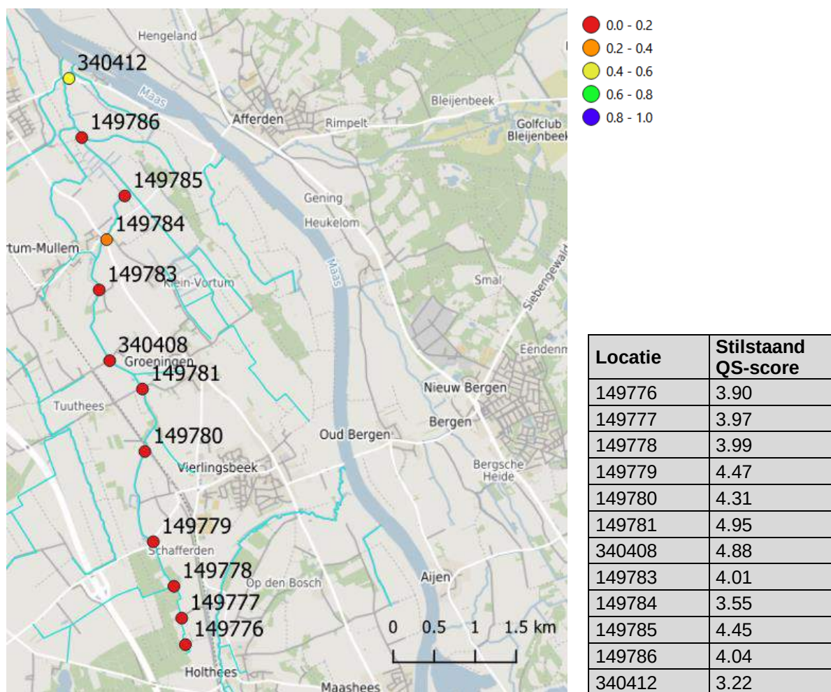
Figuur 5: Quicksan beoordeling meetlocaties St. Jansbeek op basis van het aandeel stilstaand water prefererende taxa in de macrofaunalevensgemeenschap. De kwaliteit, uitgedrukt in een schaal van 0 (slecht) tot 1 (goed), is weergegeven met verschillende kleuren en is gestandaardiseerd naar de waarden die optreden in de slechtste en beste locaties in Nederland. In de tabel worden daarnaast de absolute milieu- en habitatpreferentiescores voor de locaties gegeven, niet gestandaardiseerd.
