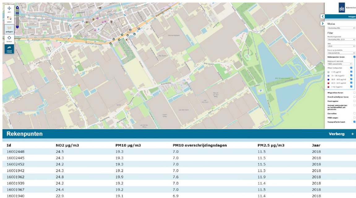
Figuur 2: jaargemiddelde concentraties NO 2 , PM 10 en PM 2,5 ; peiljaar 2018 met de globale ligging van het plangebied
