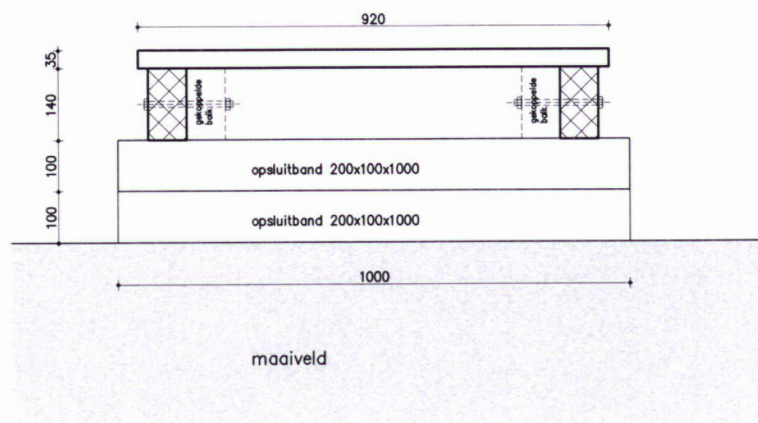
Principe doorsnede
