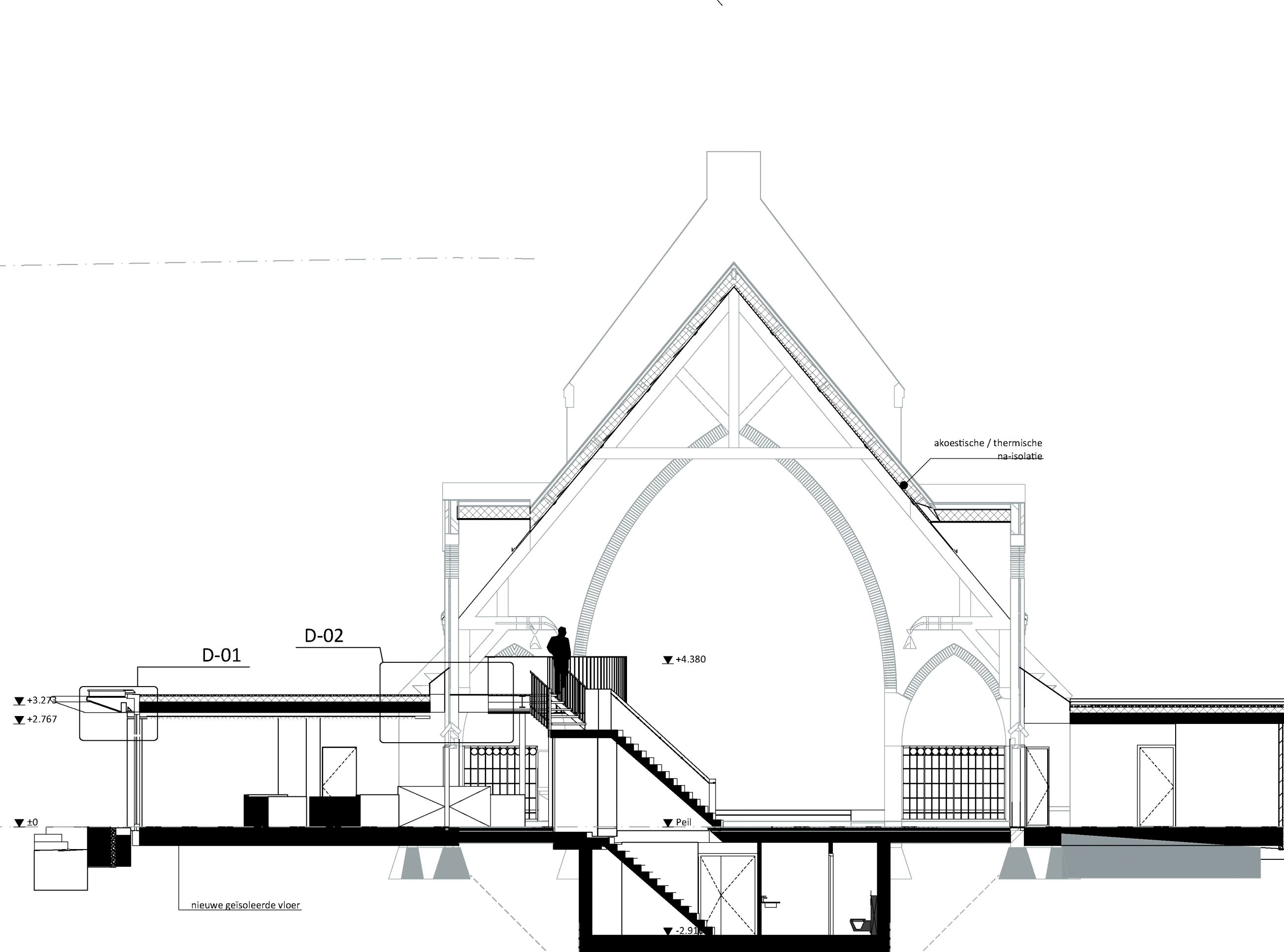
doorsnede D-D
