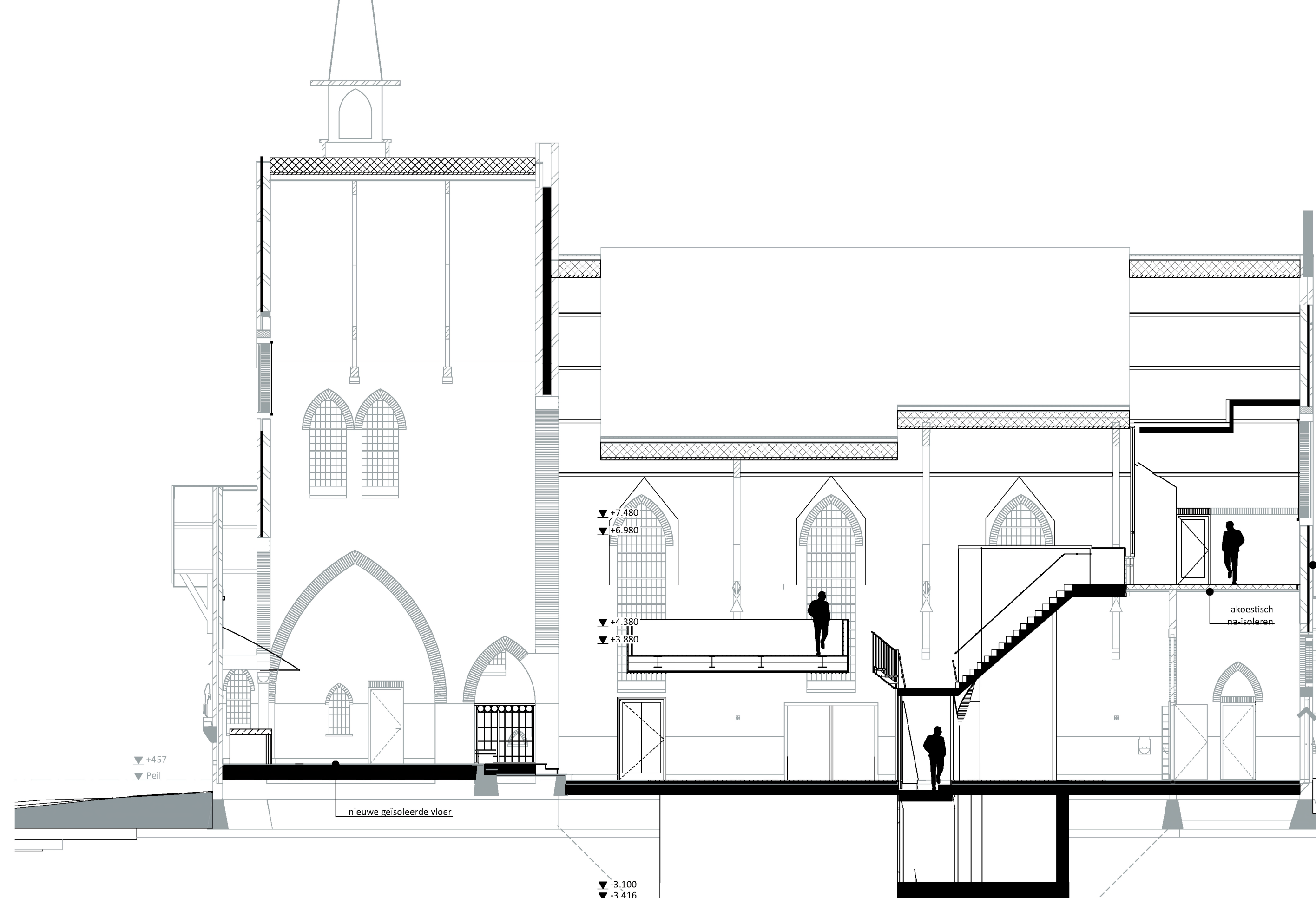
doorsnede B-B
