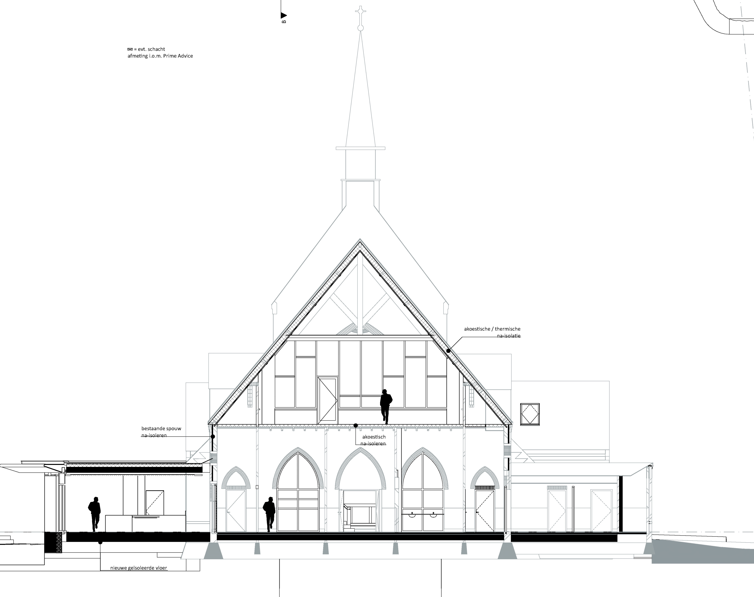
doorsnede A-A
