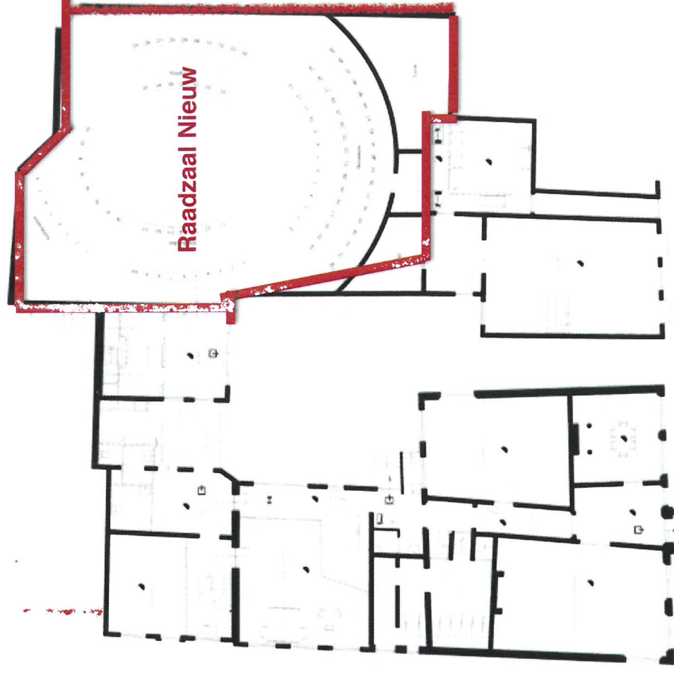
Tekening 4. Toekomstige situatie nr.72-76
