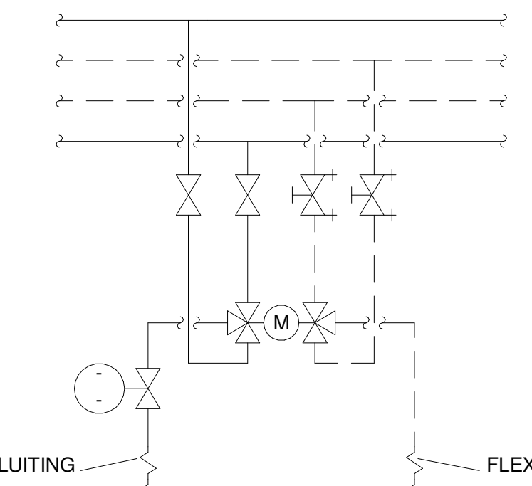
AANSLUITING PLAFOND INDUCTIEUNIT/KLIAMATPLAFOND Detail A
