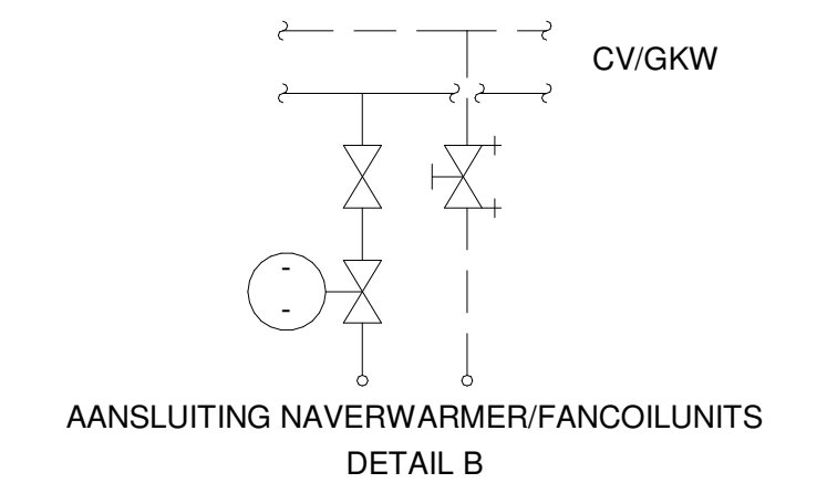
DETAIL AANSLUITING PLAFOND INDUCTIEUNITEN/KLIAMATPLAFOND
