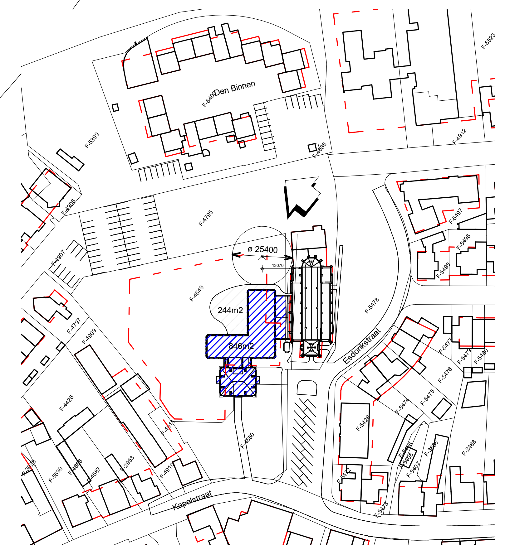
Situatie 1:1000
