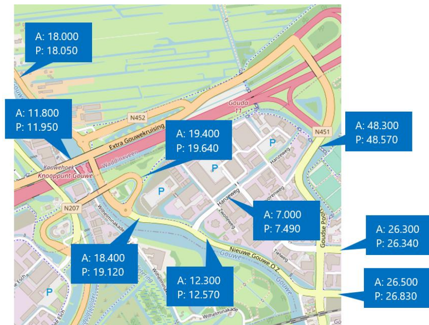
Figuur 3.4: Verkeersintensiteiten (mvt per werkdagemaal) in de autonome situatie 2030 (A) en de plansituatie 2030 (P)
