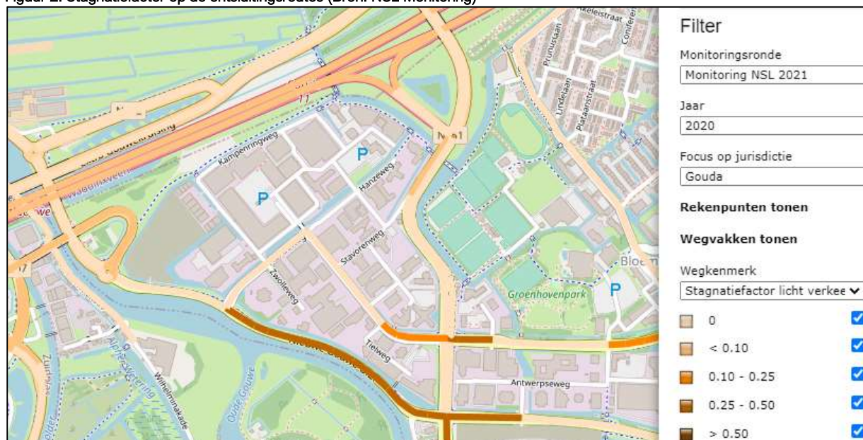
Figuur 2. Stagnatiefactor op de ontsluitingsroutes (Bron: NSL Monitoring)
