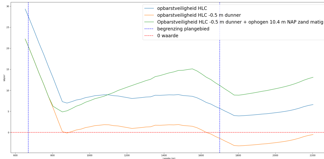
Figuur 6.9 Opbarstrisico verschil tussen gronddruk en opwaartstdruk 1 e watervoerende pakket voor 3 verschillende scenario's
