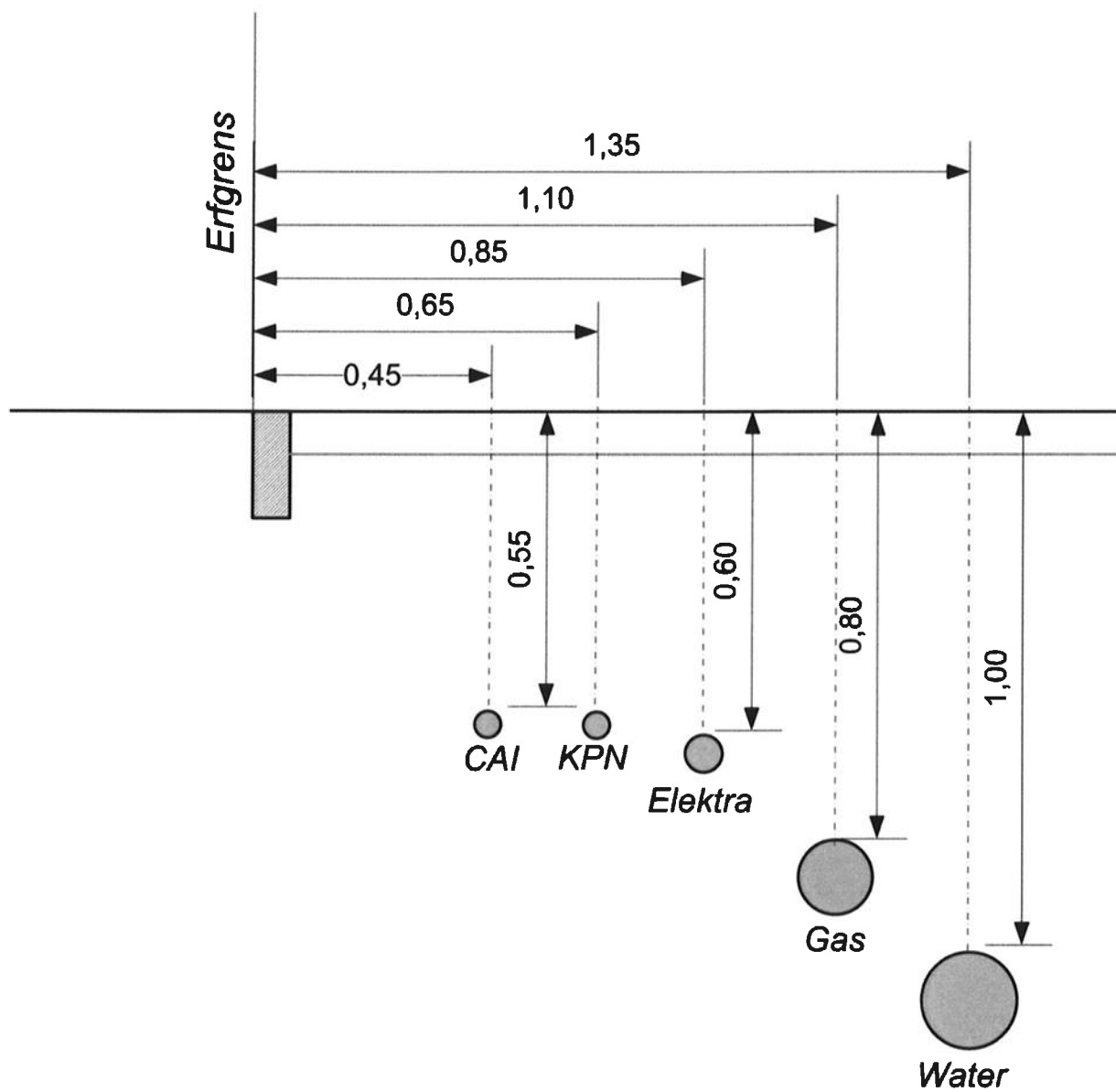
Standaarddwarsprofiel woonstraat
