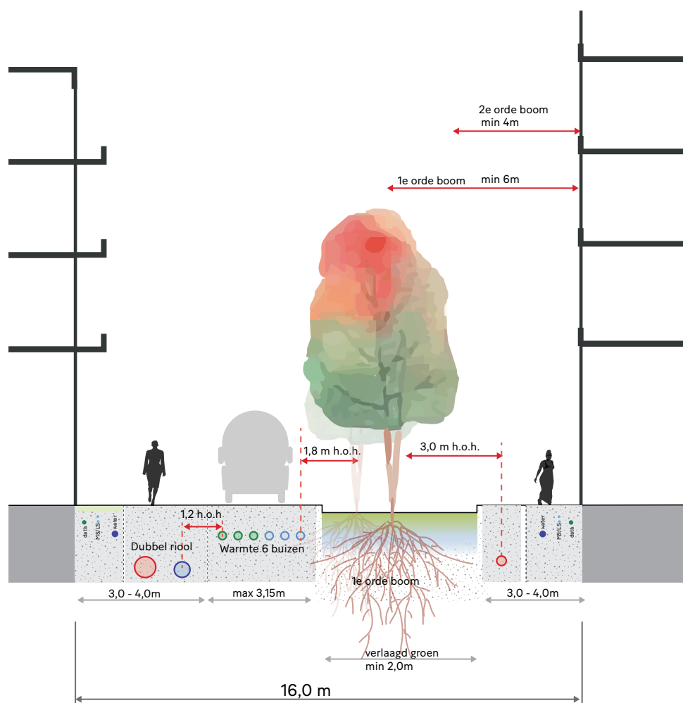
Abbeelding 197. Voorbeeld van ligging van ondergrondse infrastructuur in de straatprofiel
