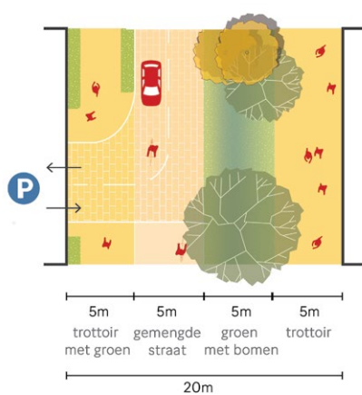
Afbeelding 60. Profielen Entreestraat (inprikker)
