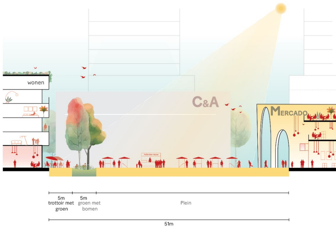
Afbeelding 75. Profiel Mercadoplein
