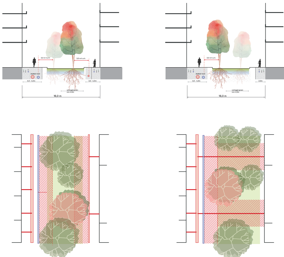
Afbeelding 196. Twee varianten van ligging van het vuilwaterriool en effect op de positie van bomen
