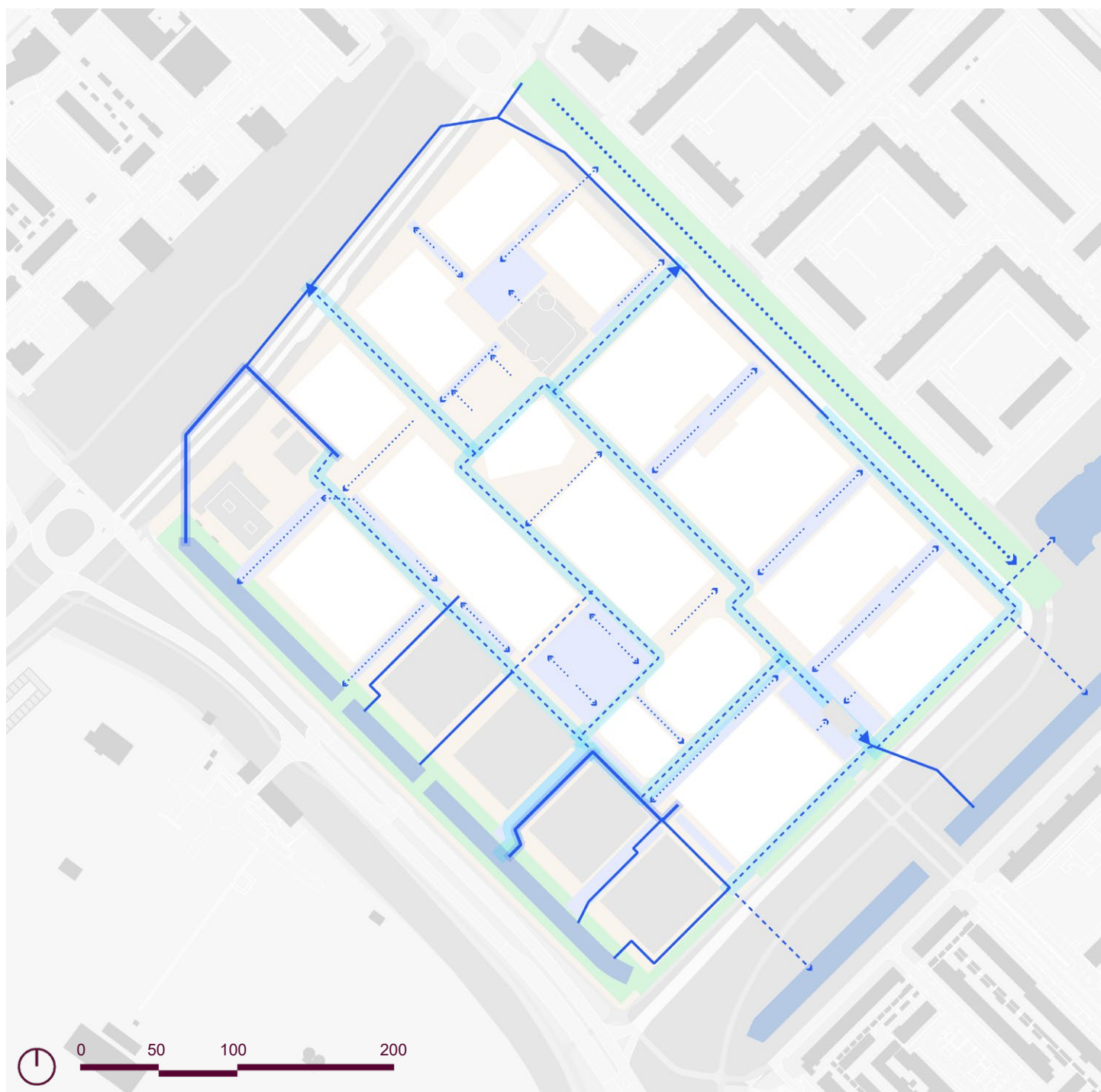
Afbeelding 126. Overzichtskaart afwatering Overvecht Centrum
