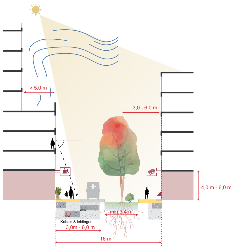
Afbeelding 57. Basisprofiel Overvecht Centrum
