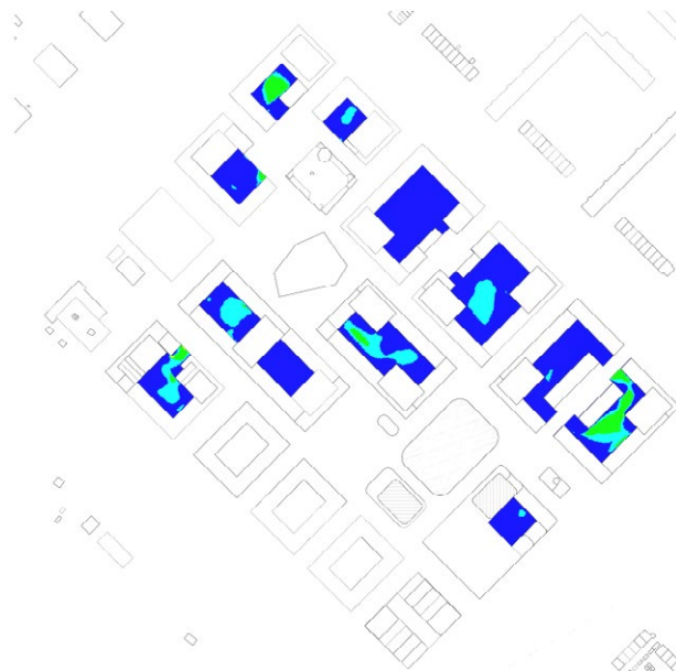
Afbeelding 191. Beoordeling windhinder op daktuinen
