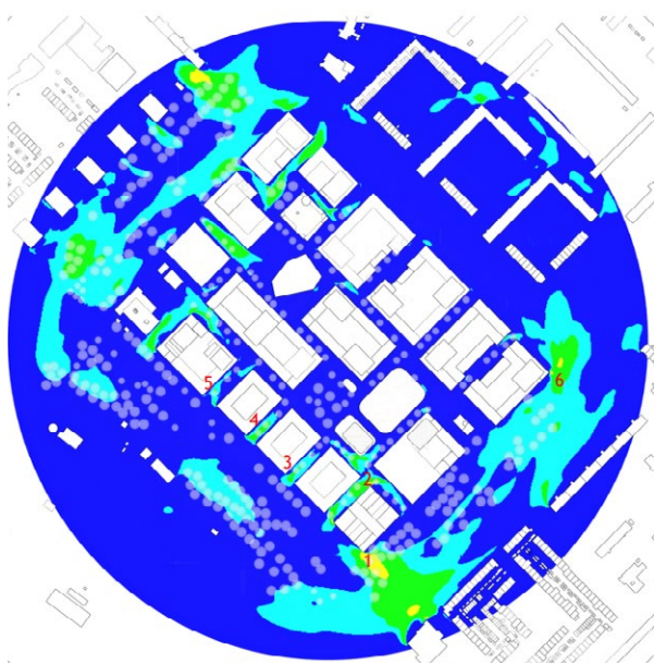
Afbeelding 190. Beoordeling windhinder op straatniveau
