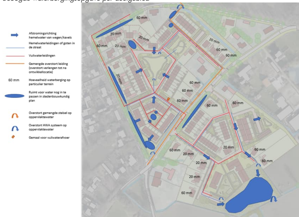
Globale schets waterberging en waterstructuren deelgebied A en B
