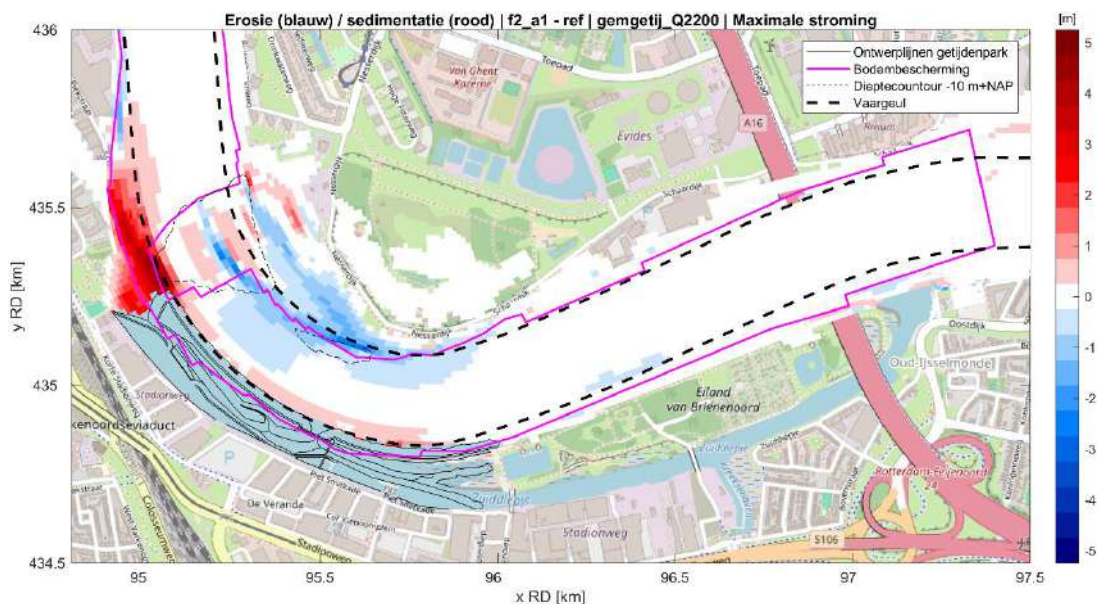
Figuur 4.17: Verwachte beeld van de erosie en sedimentatie door aanleg van het getijdenpark op basis van het verschil in evenwichtsdiepte tussen de referentie en fase 2 van het getijdenpark. Gebaseerd op de waarde tijdens maximale stroming voor iedere roostercel bij mediane rivierafvoer (2200 m 3 /s) en gemiddeld getij. De gebieden van het getijdenpark en het Zuiddiepje zijn hier buiten beschouwing gelaten.
