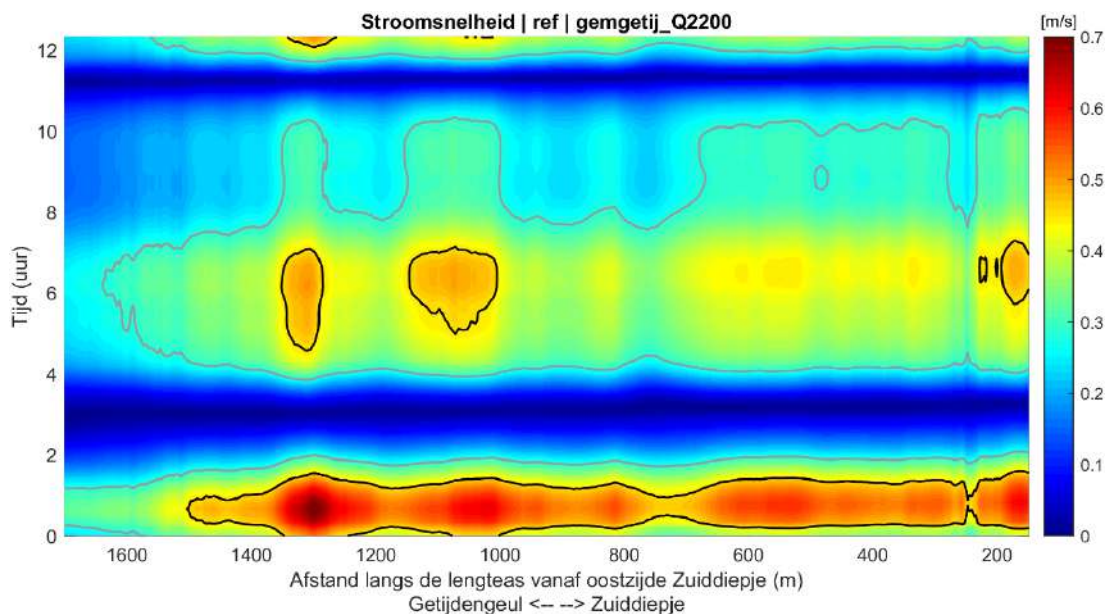
Figuur 4.27: Stroomsnelheid in de tijd (getijcyclus) in de referentiesituatie langs de lengteas van het Zuiddiepje, met contouren van de kritische stroomsnelheid van 0,28 \text{ m/s} (grijze lijn) en 0,45 \text{ m/s} (zwarte lijn).
