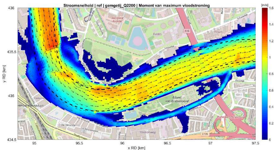
Fig. C.2: Stroomveld in de referentiesituatie tijdens maximale vloedstroom bij mediane rivierafvoer (2200 m 3 /s) en gemiddeld getij.
