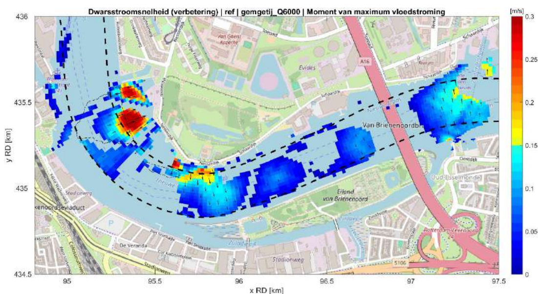
Fig. D.20: Stroomsnelheid dwars op de randen van de vaargeul voor de referentiesituatie tijdens maximale ebstroom bij hoge rivierafvoer ( 6000 \text{ m}^3/\text{s} ) en gemiddeld getij. Alleen cellen met verbetering door het getijdenpark ten opzichte van de referentiesituatie zijn weergegeven. De gebieden van het getijdenpark en het Zuiddiepje zijn hier buiten beschouwing gelaten.
