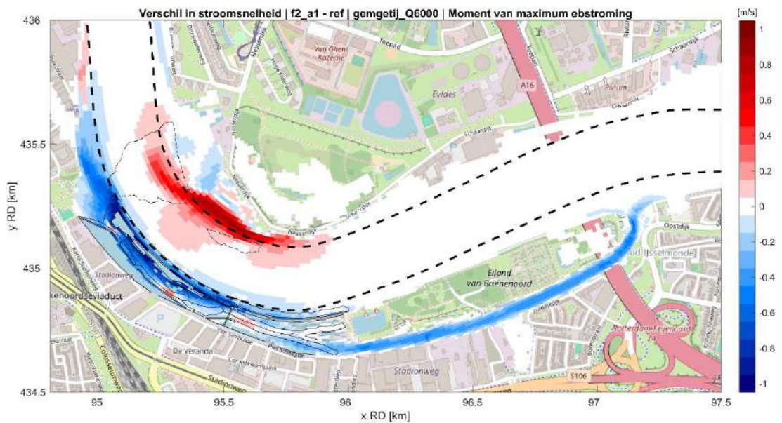
Fig. C.16: Verschil in stroomsnelheid tussen de referentiesituatie en de situatie met getijdenpark (fase 2) tijdens maximale ebstroming bij hoge rivierafvoer ( 6000 \text{ m}^3/\text{s} ) en gemiddeld getij. Rood geeft een toename in stroomsnelheid t.g.v. het getijdenpark weer, blauw een afname in stroomsnelheid.
