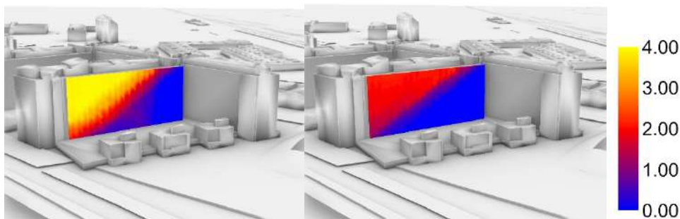
Figuur 8 Bezonning op de gevel in oude en nieuwe situatie voor Bertus Brulstraat (links en rechts respectievelijk)
