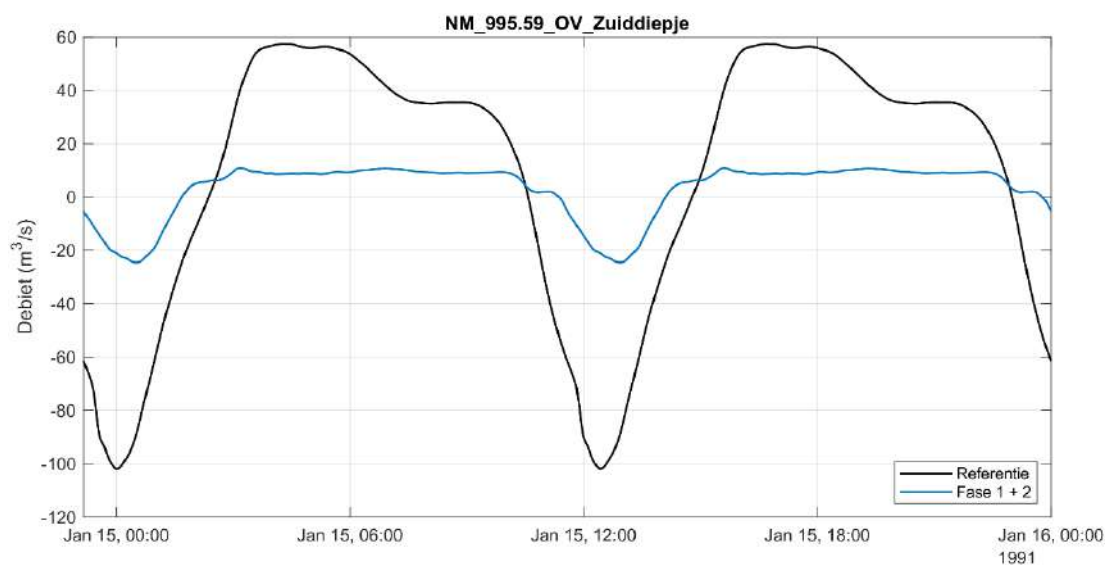
Figuur 4.24: Afvoer door het Zuiddiepje in de referentiesituatie (zwarte lijn) en voor fase 2 van het getijdenpark (blauwe lijn) voor de conditie met gemiddeld getij en mediane rivierafvoer.
