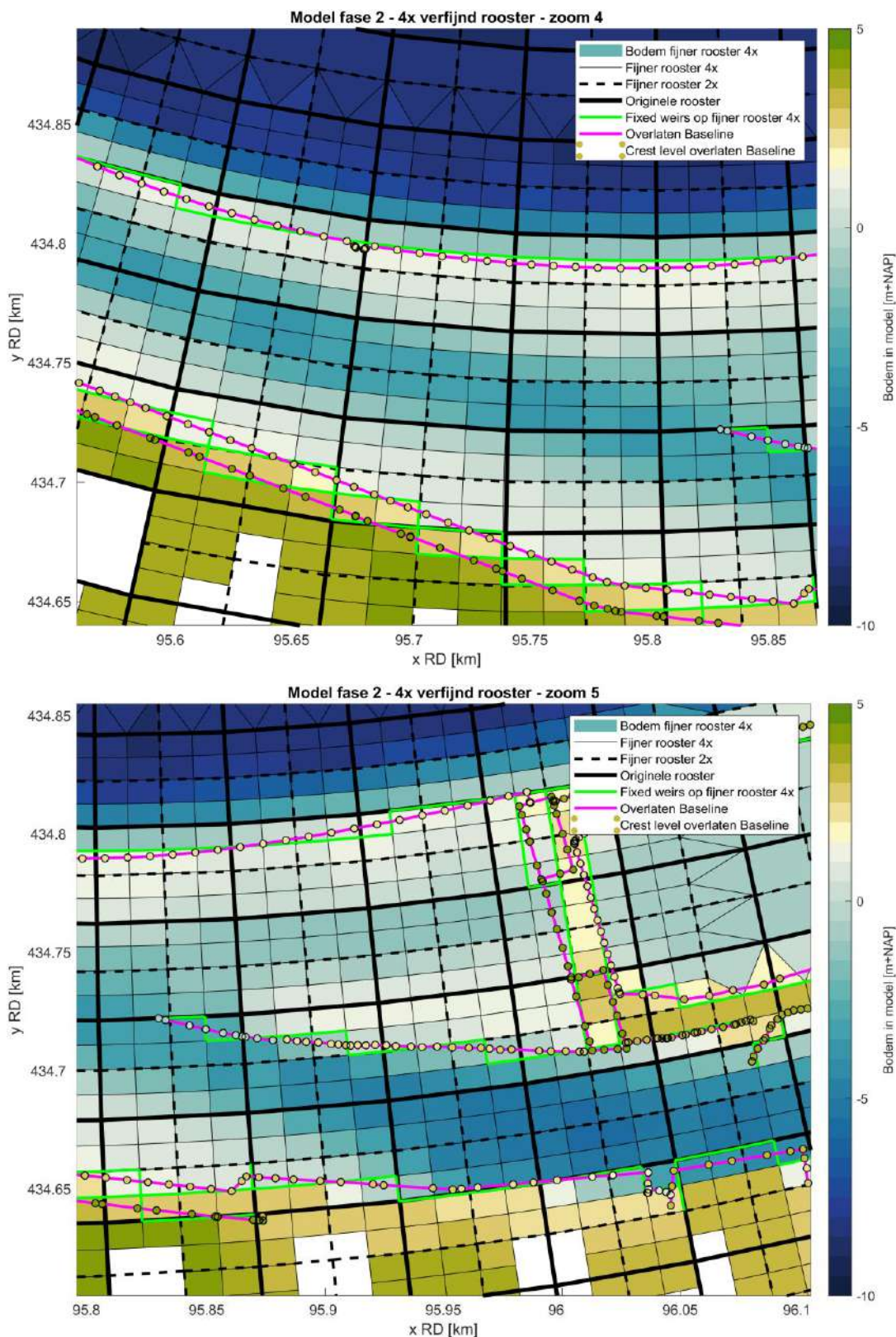
Figuur B.9: Projecties van de Baseline schematisatie van het ontwerp van het getijdenpark op het 4x verfijnde rooster, zie Figuur B.6 voor de locatie van de zooms. De drie verschillende roosters zijn weergegeven met de zwarte (stippel)lijnen, de kleurschaal geeft de bodemligging in het 4x verfijnde rooster weer, de groene lijnen tonen de locaties van de gesnappede overlaten in het D-HYDRO model en de magentalijnen bevatten de locaties van de overlaten vanuit Baseline, met in de gekleurde bolletjes de kruinhoogtes van deze overlaten.
