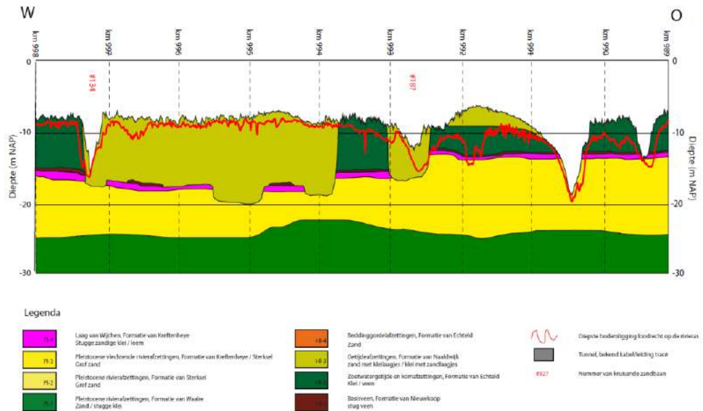
Figuur 4.20: Bodemsoorten langs de lengteas van de Nieuwe Maas. Het invloedsgebied van het getijdenpark (996-997,5km) is te vinden in het linker gedeelte van de figuur. Bron: Deltares, 2015.
