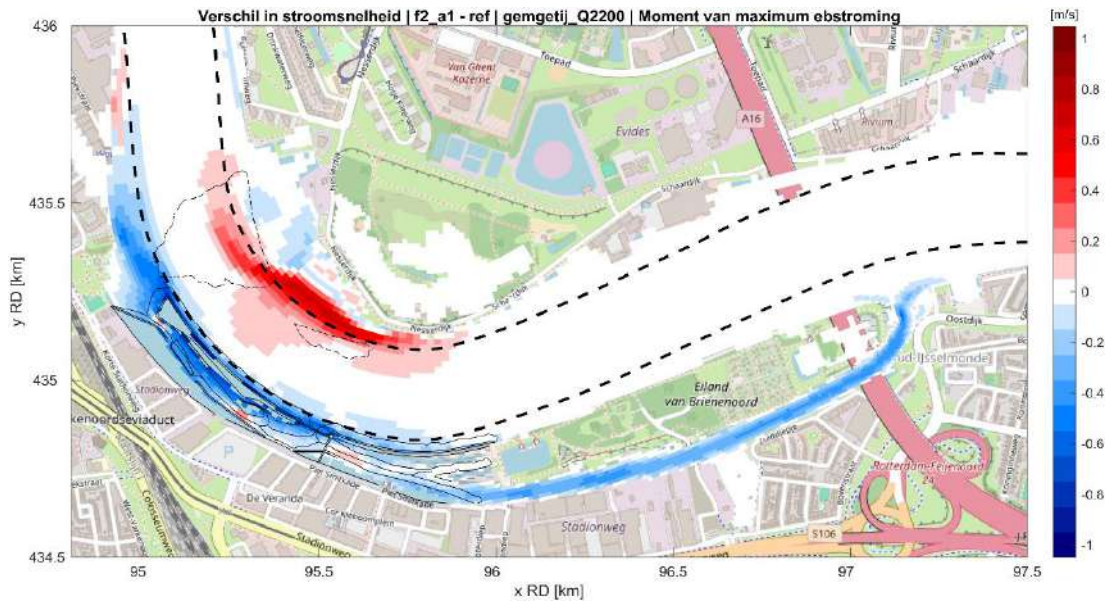
Fig. C.7: Verschil in stroomsnelheid tussen de referentiesituatie en de situatie met getijdenpark (fase 2) tijdens maximale ebstroom bij hoge rivierafvoer ( 6000 \text{ m}^3/\text{s} ) en gemiddeld getij. Rood geeft een toename in stroomsnelheid t.g.v. het getijdenpark weer, blauw een afname in stroomsnelheid.
