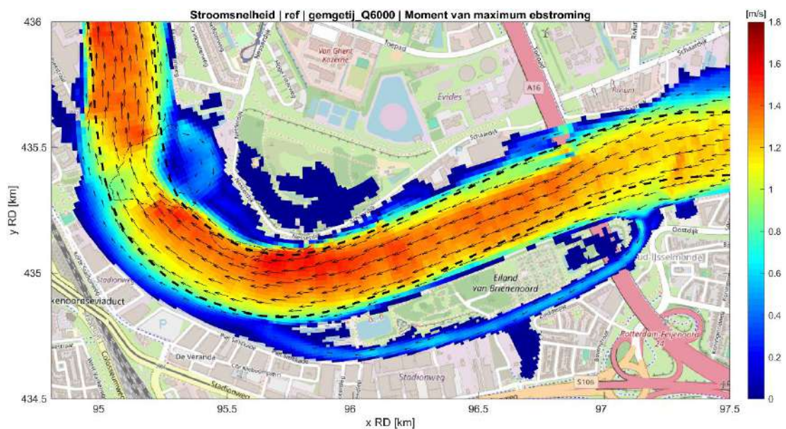
Figuur 4.5: Stroomveld in de Nieuwe Maas in de referentiesituatie tijdens maximale ebstroom bij hoge rivierafvoer (6000 m 3 /s) en gemiddeld getij.
