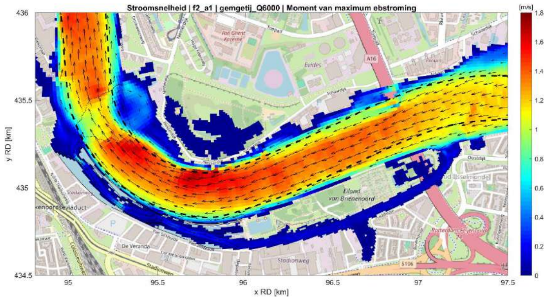
Fig. C.13: Stroomveld in de situatie met getijdenpark (fase 2) tijdens maximale ebstroom bij hoge rivierafvoer (6000 m 3 /s) en gemiddeld getij.
