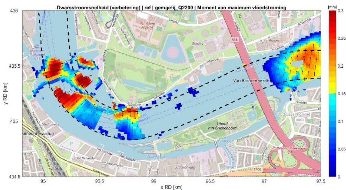
Fig. D.10: Stroomsnelheid dwars op de randen van de vaargeul voor de referentiesituatie tijdens maximale ebstroom bij mediane rivierafvoer ( 2200 \text{ m}^3/\text{s} ) en gemiddeld getij. Alleen cellen met verbetering door het getijdenpark ten opzichte van de referentiesituatie zijn weergegeven. De gebieden van het getijdenpark en het Zuiddiepje zijn hier buiten beschouwing gelaten.
