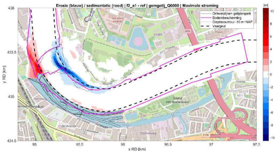
Figuur 4.18: Meer extreem beeld van de erosie door aanleg van het getijdenpark op basis van het verschil in evenwichtsdiepte tussen de referentie en fase 2. Gebaseerd op de waarde tijdens maximale stroming voor iedere rooster cel bij een hoge rivierafvoer (6000 m 3 /s) en gemiddeld getij. De gebieden van het getijdenpark en het Zuiddiepje zijn hier buiten beschouwing gelaten.
