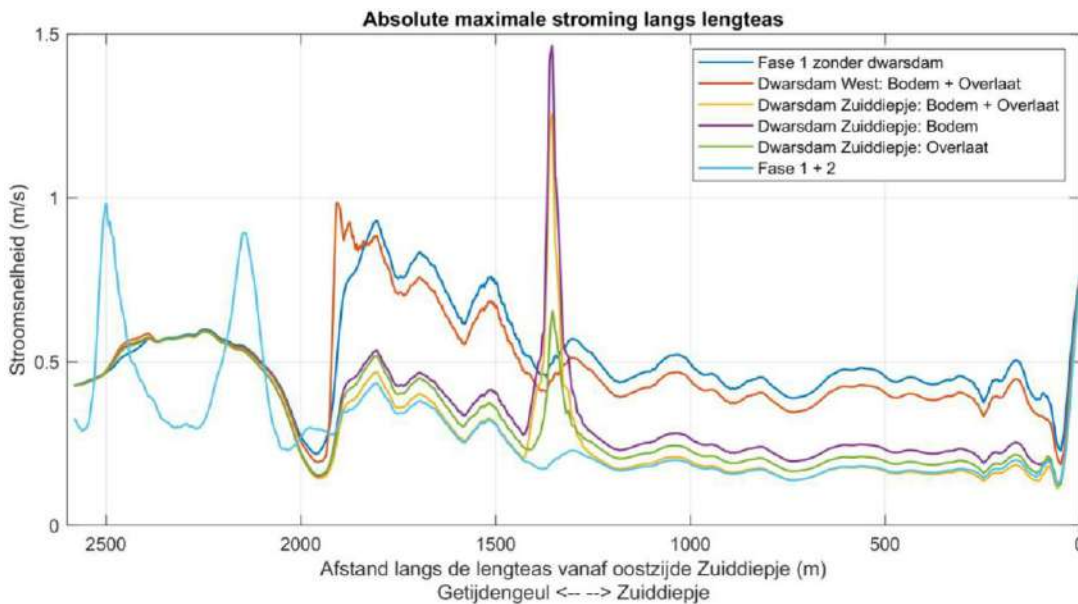
Figuur 4.12. Vergelijking van de maximale stroomsnelheid bij vloed door het Zuiddiepje (0 – 1400 m) en het getijdenpark (fase 1: 1400-1975 m; fase 2: 1975-2580) voor verschillende varianten (Svašek Hydraulics, 2025).
