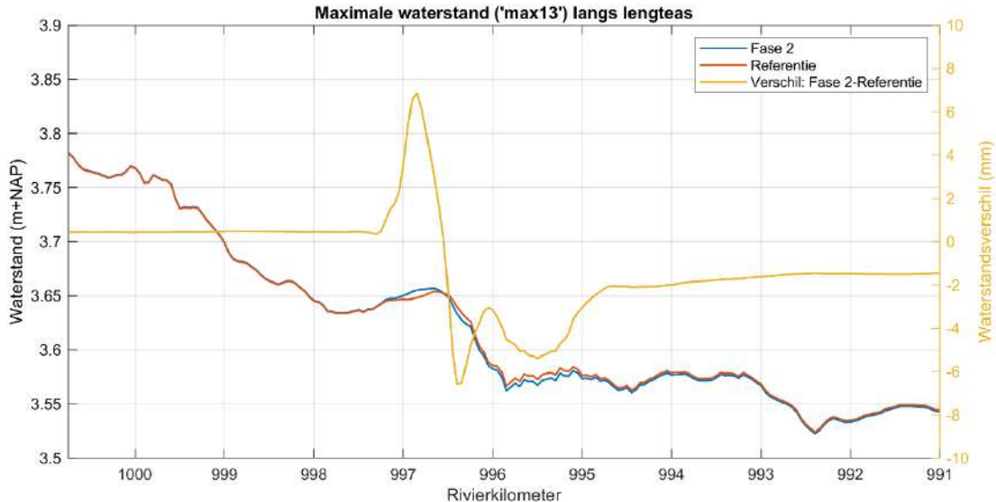
Figuur 4.1: Maximale waterstand in de referentiesituatie (rood) en de situatie met het getijdenpark (fase 2, blauw) en het verschil daartussen (geel).
