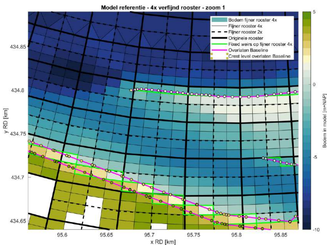
Figuur B.2: Projectie van de Baseline schematisatie van de referentiesituatie op het 4x verfijnde rooster, zie Figuur B.1 voor de locatie van de zoom. De drie verschillende roosters zijn weergegeven met de zwarte (stippel)lijnen, de kleurschaal geeft de bodemligging in het 4x verfijnde rooster weer, de groene lijnen tonen de locaties van de gesnappede overlatten in het D-HYDRO model en de magentalijnen bevatten de locaties van de overlatten vanuit Baseline, met in de gekleurde bolletjes de kruinhoogtes van deze overlatten.
