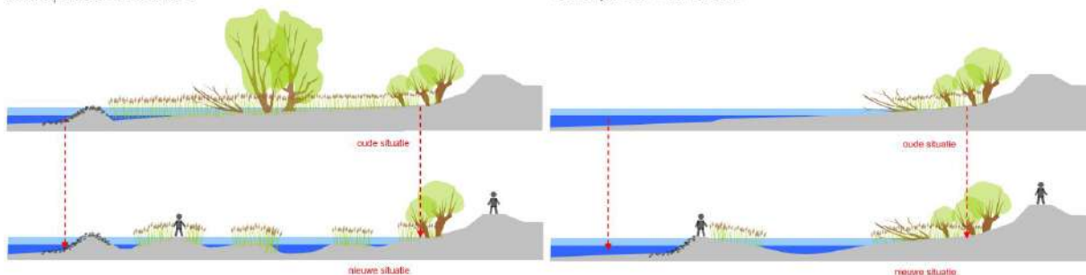
Figuur 3.4. KRW-maatregel Grote en Kleine Zaag (De Jong et al., 2023) met in de dwarsdoorsnedes principeschetsen van de maatregel.
