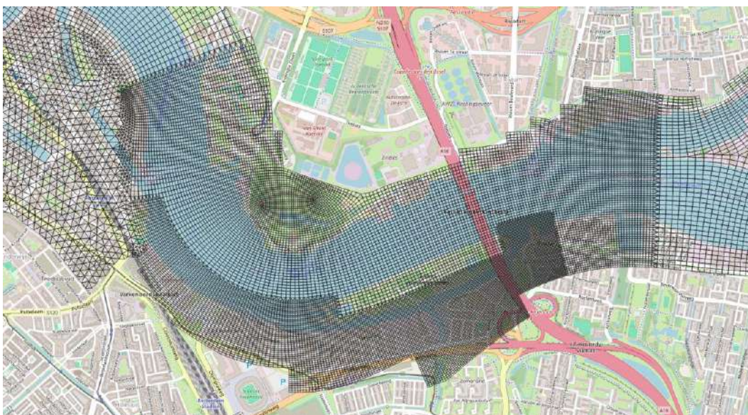
Figuur 3.2: Modelrooster van het 4x verfijnde rooster rondom het projectgebied.
