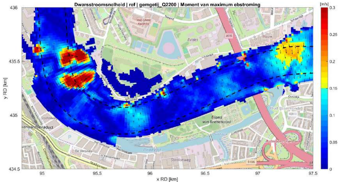
Fig. D.1: Strooming dwars op de randen van de vaargeul in de referentiesituatie tijdens maximale ebstroom bij mediane rivierafvoer (2200 m 3 /s) en gemiddeld getij. Het gebied van het Zuiddiepe zijn hier buiten beschouwing gelaten.
