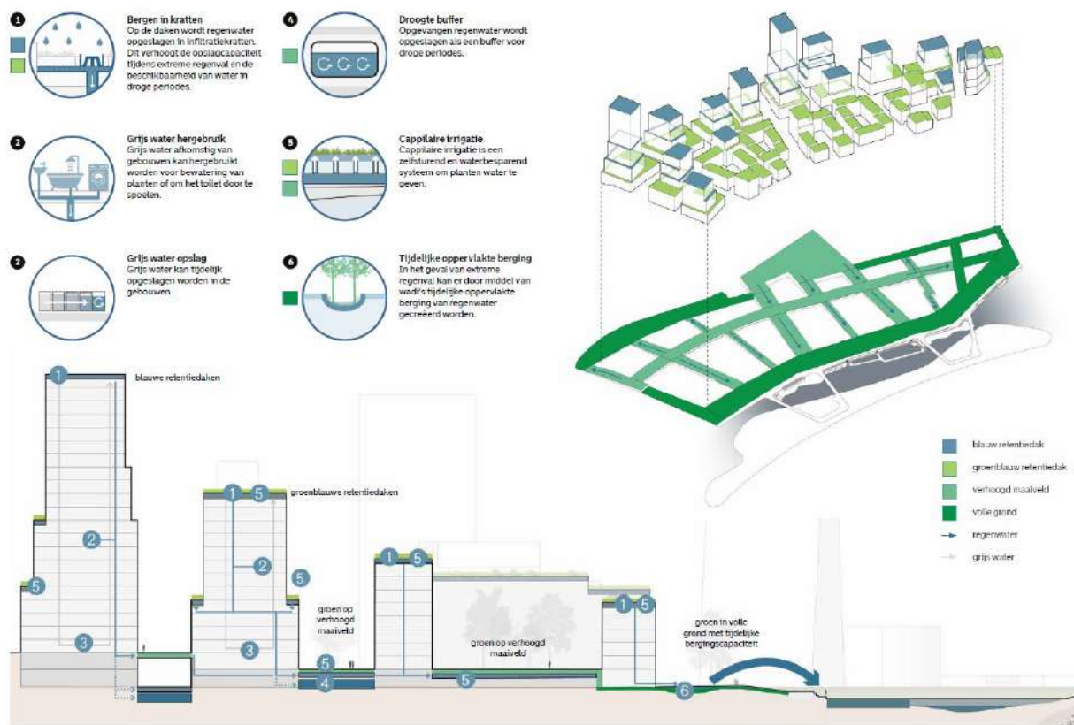
Figuur 4-4: Waterberging Waterkant Ambitiedocument.
