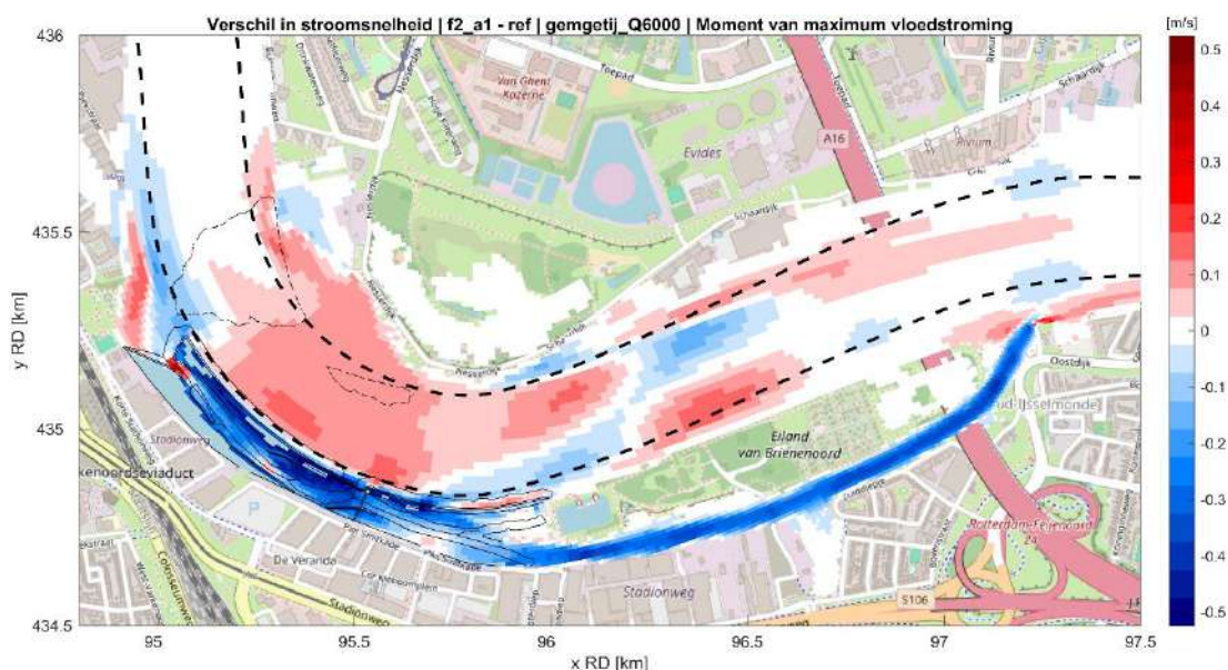
Fig. C.17: Verschil in stroomsnelheid tussen de referentiesituatie en de situatie met getijdenpark (fase 2) tijdens maximale vloedstroom bij hoge rivierafvoer ( 6000 \text{ m}^3/\text{s} ) en gemiddeld getij. Rood geeft een toename in stroomsnelheid t.g.v. het getijdenpark weer, blauw een afname in stroomsnelheid.
