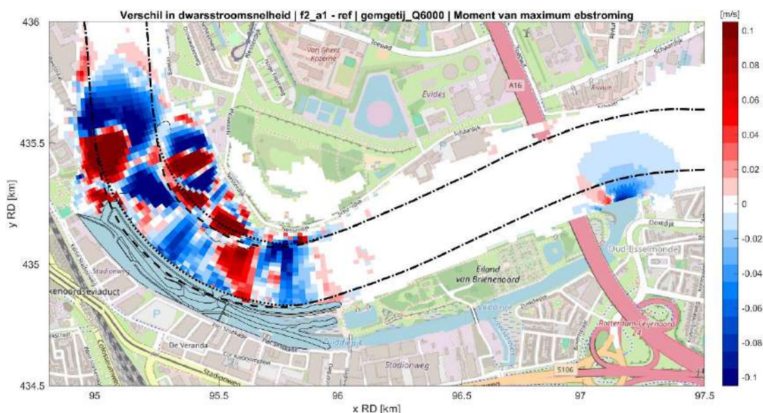
Figuur 4.12: Verschil in stroomsnelheid dwars op de randen van de vaargeul tussen de referentiesituatie en de situatie met getijdenpark (fase 2) tijdens maximale ebstroom bij hoge rivierafvoer ( 6000 \text{ m}^3/\text{s} ) en gemiddeld getij. Rood geeft een toename in dwarsstroomsnelheid t.g.v. het getijdenpark weer, blauw een afname in dwarsstroomsnelheid. De gebieden van het getijdenpark en het Zuiddiepje zijn hier buiten beschouwing gelaten.
