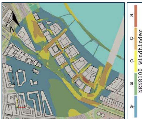
Figuur Bijlage B-2: Overzicht windhinderkaart, nieuwe situatie
