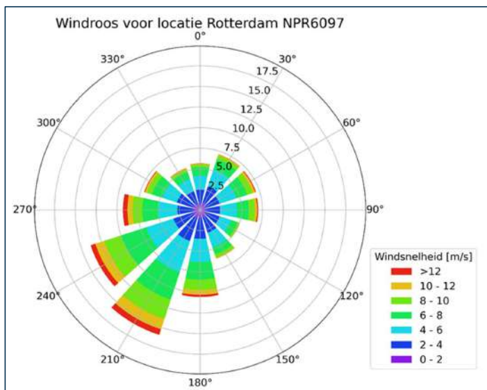
Figuur 3-3: Windroos van Rotterdam uit NPR6097:2006
