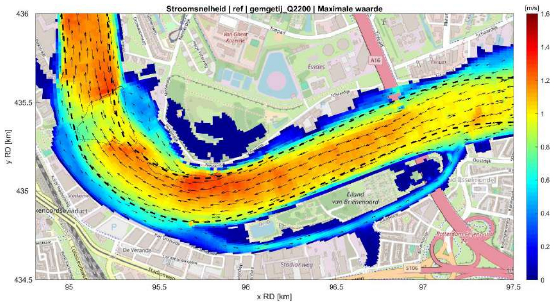
Fig. C.3: Maximale stroming tijdens de simulatie met de referentiesituatie bij mediane rivierafvoer ( 2200 \text{ m}^3/\text{s} ) en gemiddeld getij.
