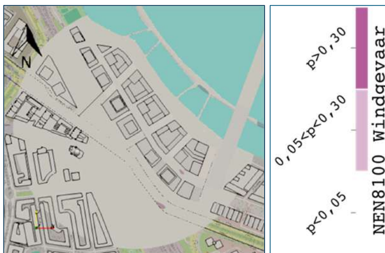
Figuur Bijlage C-2: Overzicht windgevaarkaart, nieuwe situatie
