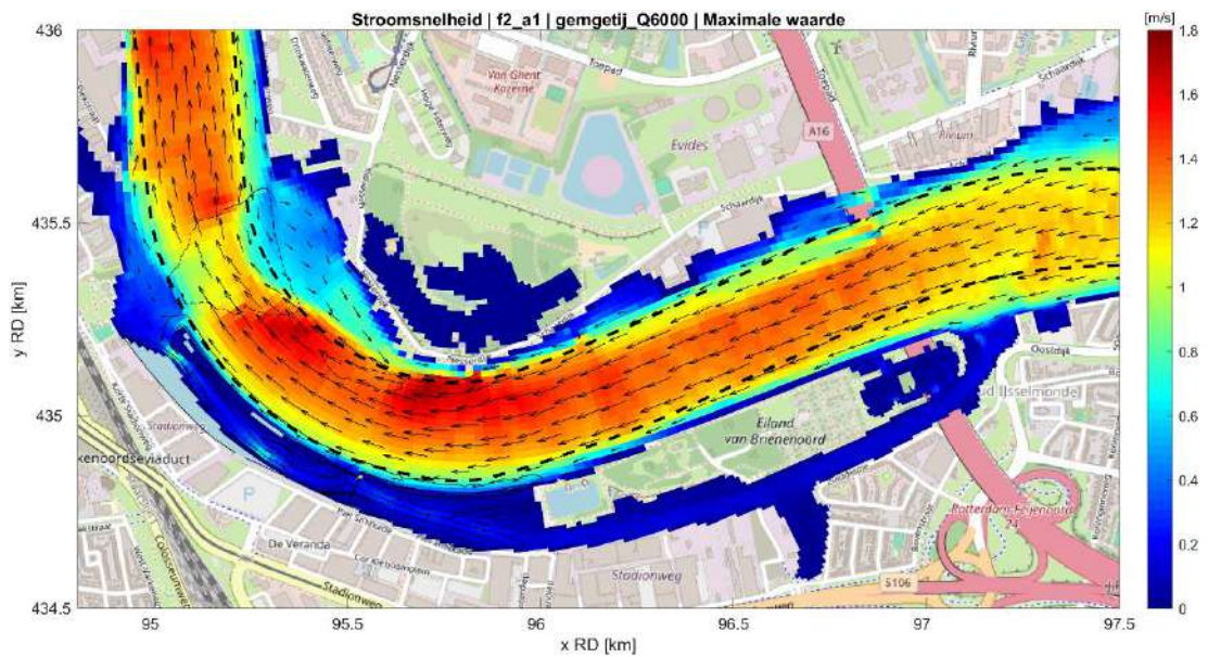
Fig. C.15: Maximale stroming tijdens de simulatie met getijdenpark (fase 2) bij hoge rivierafvoer ( 6000 \text{ m}^3/\text{s} ) en gemiddeld getij.
