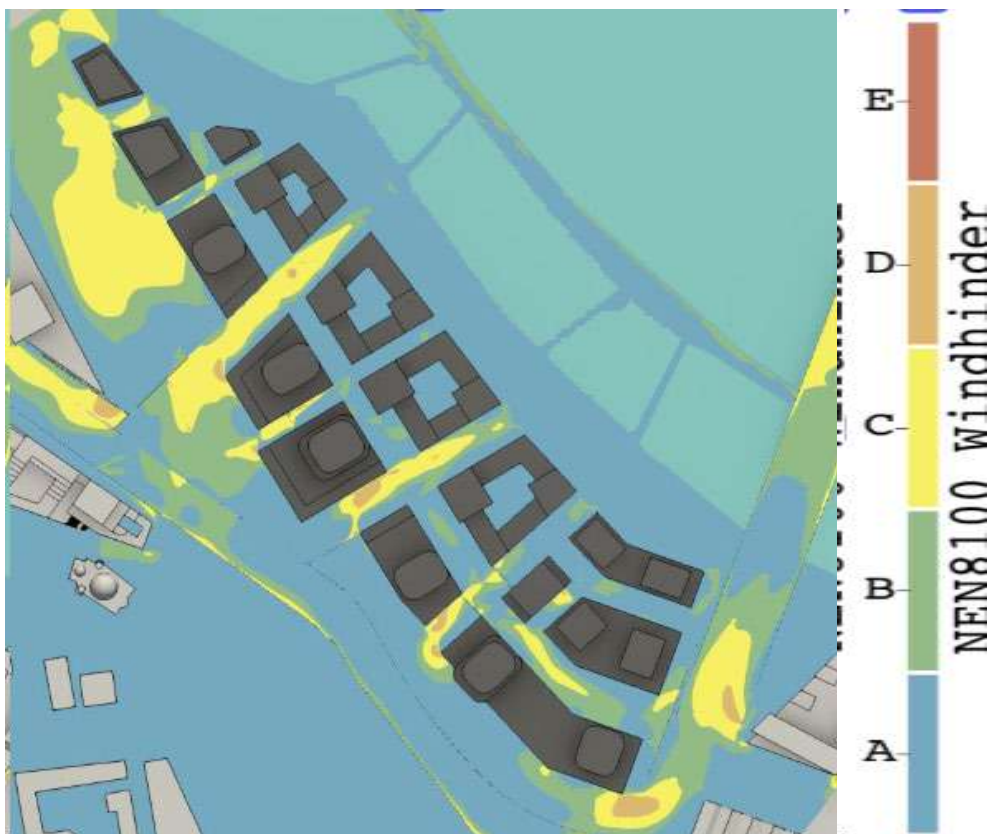
figuur 5.12.5 Kans op windhinder aangepast stedenbouwkundig model
