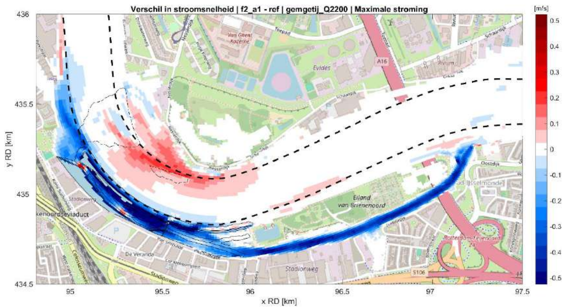
Fig. C.9: Verschil in maximale stroomsnelheid tussen de referentiesituatie en de situatie met getijdenpark (fase 2) tijdens de gehele simulatie met mediane rivierafvoer (2200 m 3 /s) en gemiddeld getij. Rood geeft een toename in stroomsnelheid t.g.v. het getijdenpark weer, blauw een afname in stroomsnelheid.
