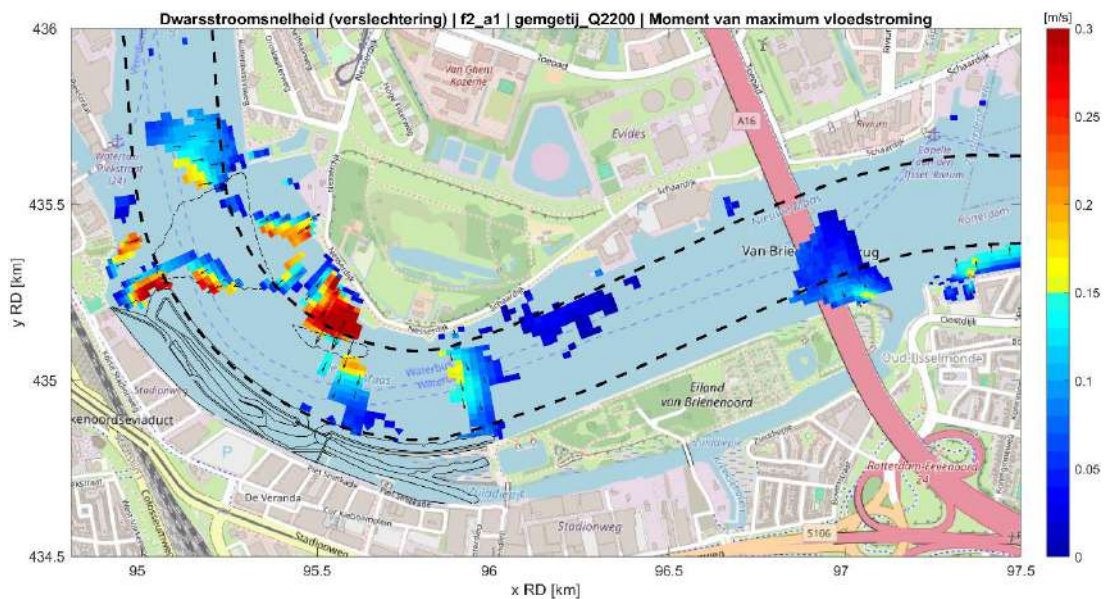
Fig. D.8: Stroomsnelheid dwars op de randen van de vaargeul voor de situatie met getijdenpark (fase 2) tijdens maximale ebstroom bij mediane rivierafvoer ( 2200 \text{ m}^3/\text{s} ) en gemiddeld getij. Alleen cellen met verhoging ten opzichte van de referentiesituatie zijn weergegeven. De gebieden van het getijdenpark en het Zuiddiepje zijn hier buiten beschouwing gelaten.
