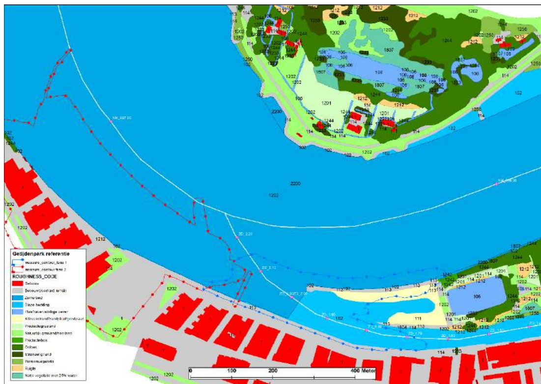
Figuur 3.4: Ruwheden in de Baseline schematisatie van de referentie situatie.
