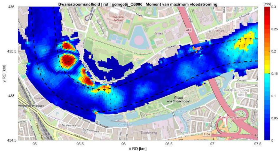
Fig. D.12: Strooming dwars op de randen van de vaargeul in de referentiesituatie tijdens maximale vloedstroom bij hoge rivierafvoer (6000 m 3 /s) en gemiddeld getij. Het gebied van het Zuiddiepje zijn hier buiten beschouwing gelaten.
