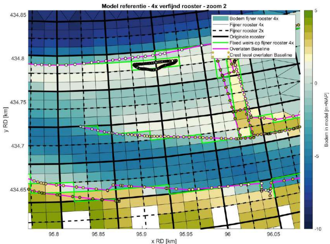
Figuur 3.5: Projectie van de Baseline schematisatie van de referentiesituatie op het 4x verfijnde rooster, zie Figuur B.1 voor de locatie van de zoom. De drie verschillende roosters zijn weergegeven met de zwarte (stippel)lijnen, de kleurschaal geeft de bodemligging in het 4x verfijnde rooster weer, de groene lijnen tonen de locaties van de gesnappede overlaten in het D-HYDRO model en de magentalijnen bevatten de locaties van de overlaten vanuit Baseline, met in de gekleurde bolletjes de kruinhoogtes van deze overlaten.
