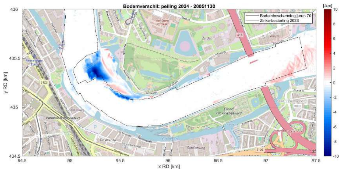
Figuur 4.16: Bodemverschil tussen bodempeilingen uit 2024 en 2005 inclusief ligging van bodembescherming uit jaren 70 (zwart omlijnd) en een zinkerbestorting uit 2023 (grijs omlijnd).
