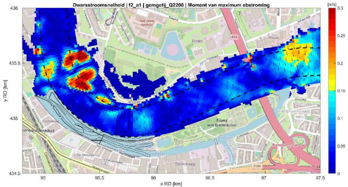
Fig. D.3: Strooming dwars op de randen van de vaargeul in de situatie met getijdenpark (fase 2) tijdens maximale ebstroom bij mediane rivierafvoer ( 2200 \text{ m}^3/\text{s} ) en gemiddeld getij. De gebieden van het getijdenpark en het Zuiddiepje zijn hier buiten beschouwing gelaten.
