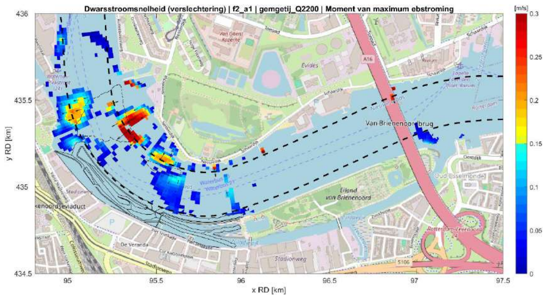
Fig. D.7: Stroomsnelheid dwars op de randen van de vaargeul voor de situatie met getijdenpark (fase 2) tijdens maximale ebstroom bij mediane rivierafvoer ( 2200 \text{ m}^3/\text{s} ) en gemiddeld getij. Alleen cellen met verhoging ten opzichte van de referentiesituatie zijn weergegeven. De gebieden van het getijdenpark en het Zuiddiepje zijn hier buiten beschouwing gelaten.
