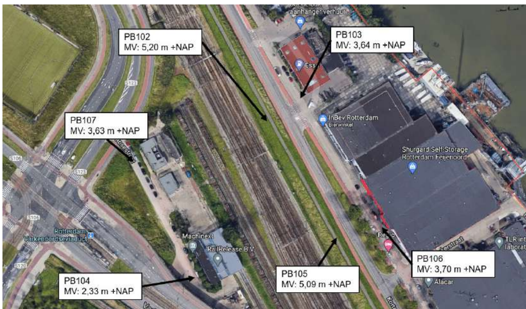
Figuur 2: Locaties van de zes recent geplaatste peilbuizen inclusief maximaal gemeten grondwaterstand.
