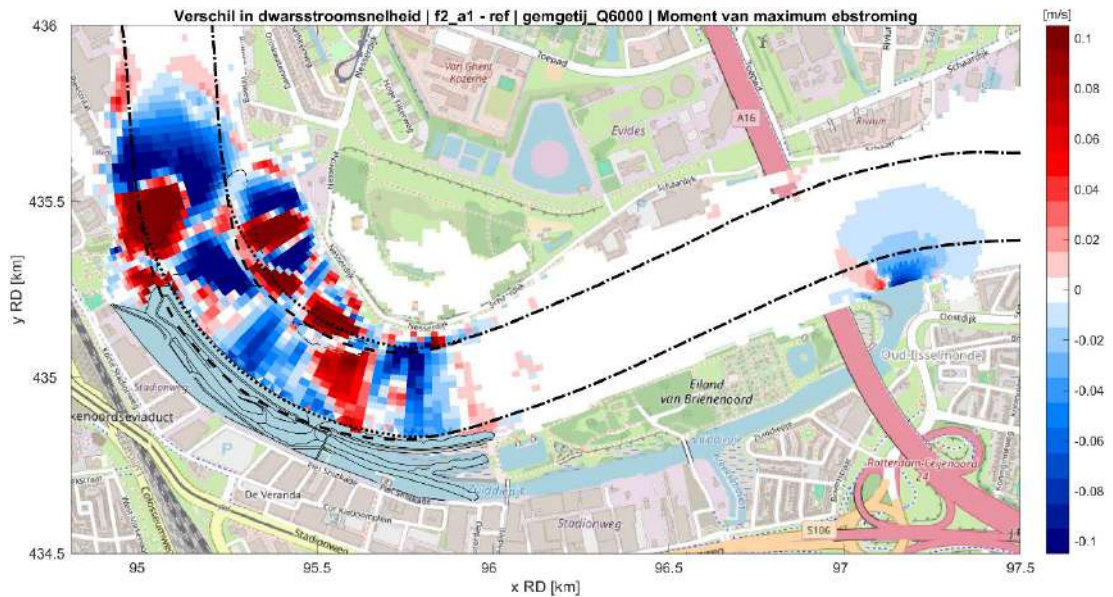
Fig. D.15: Verschil in stroomsnelheid dwars op de randen van de vaargeul tussen de referentiesituatie en de situatie met getijdenpark (fase 2) tijdens maximale ebstroom bij hoge rivierafvoer ( 6000 \text{ m}^3/\text{s} ) en gemiddeld getij. Rood geeft een toename in dwarsstroomsnelheid t.g.v. het getijdenpark weer, blauw een afname in dwarsstroomsnelheid. De gebieden van het getijdenpark en het Zuiddiepje zijn hier buiten beschouwing gelaten.
