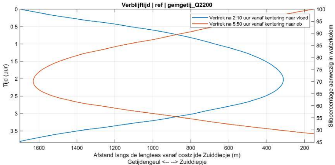
Figuur 4.25: Maximale verblijftijd voor slib en de bijbehorende slibpercentage aanwezig in de waterkolom (rechter y-as) in het Zuiddiepje in de referentiesituatie. Voor slib binnenkomend vanaf de westelijke monding (blauwe lijn) tijdens vloed en vanaf de oostelijke monding (rode lijn) tijdens eb.
