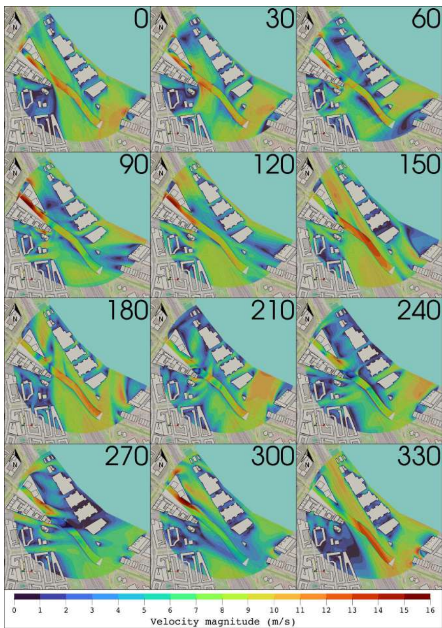
Figuur Bijlage D-1: Overzicht windsnelheidskaart op 1,75m hoogte voor alle 12 windrichtingen, huidige situatie
