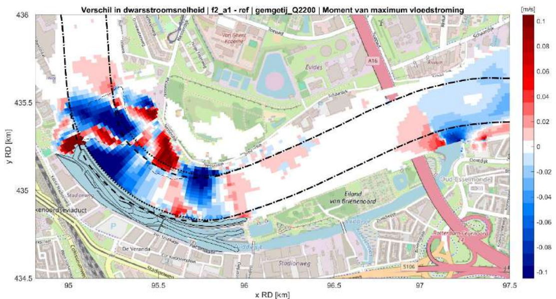
Fig. D.6: Verschil in stroomsnelheid dwars op de randen van de vaargeul tussen de referentiesituatie en de situatie met getijdenpark (fase 2) tijdens maximale vloedstroom bij mediane rivierafvoer (2200 m 3 /s) en gemiddeld getij. Rood geeft een toename in dwarsstroomsnelheid t.g.v. het getijdenpark weer, blauw een afname in dwarsstroomsnelheid. De gebieden van het getijdenpark en het Zuiddiepe zijn hier buiten beschouwing gelaten.
