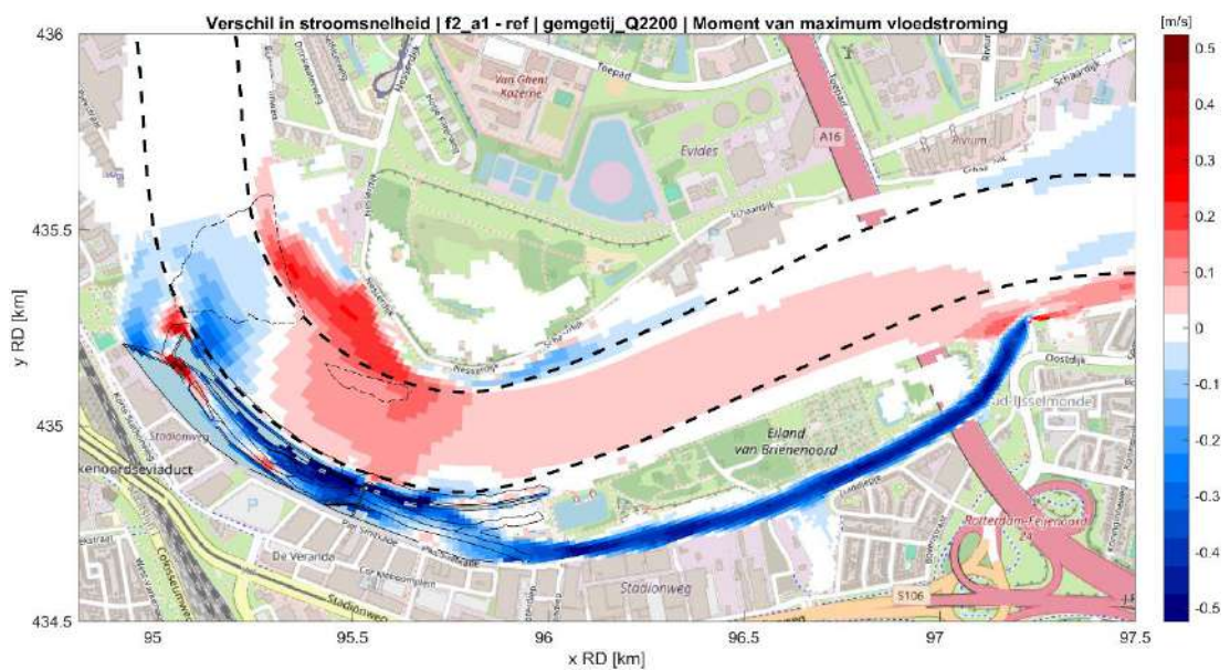
Fig. C.8: Verschil in stroomsnelheid tussen de referentiesituatie en de situatie met getijdenpark (fase 2) tijdens maximale vloedstroom bij hoge rivierafvoer ( 6000 \text{ m}^3/\text{s} ) en gemiddeld getij. Rood geeft een toename in stroomsnelheid t.g.v. het getijdenpark weer, blauw een afname in stroomsnelheid.
