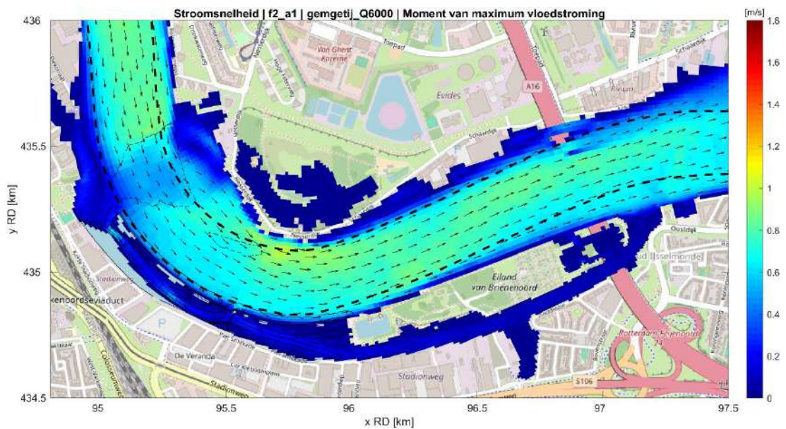
Fig. C.14: Stroomveld in de situatie met getijdenpark (fase 2) tijdens maximale vloedstroom bij hoge rivierafvoer (6000 m 3 /s) en gemiddeld getij.
