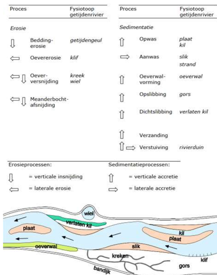
Figuur 2.7. Kenmerkende fysiotoepen in een getijdenrivier met bijbehorende processen (Middelkoop et al., 2003). Vegetatie speelt bij het ontstaan en de instandhouding van fysiotoepen een belangrijke rol.
