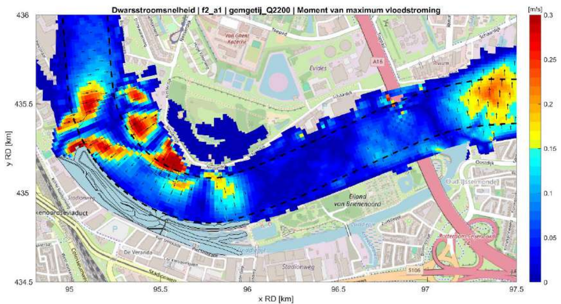
Fig. D.4: Strooming dwars op de randen van de vaargeul in de situatie met getijdenpark (fase 2) tijdens maximale vloedstroom bij mediane rivierafvoer ( 2200 \text{ m}^3/\text{s} ) en gemiddeld getij. De gebieden van het getijdenpark en het Zuiddiepje zijn hier buiten beschouwing gelaten.
