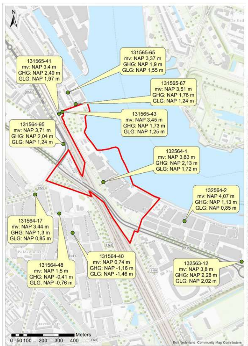
Figuur 1: Locaties peilbuizen en GHG en GLG voor de periode 2012-2019.
