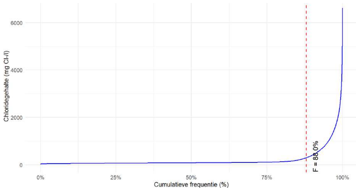
Figuur 2.5. Cumulatieve frequentie van chloridegehalten van meetpunt Brienenoordbrug op 2,5 m diepte. De verticale lijn toont waar 300 mg Cl- /l wordt bereikt (periode 2010 t/m 2024; Brienenoordbrug rechter oever (kilometer 995.2); bron: Waterinfo.rws.nl).
