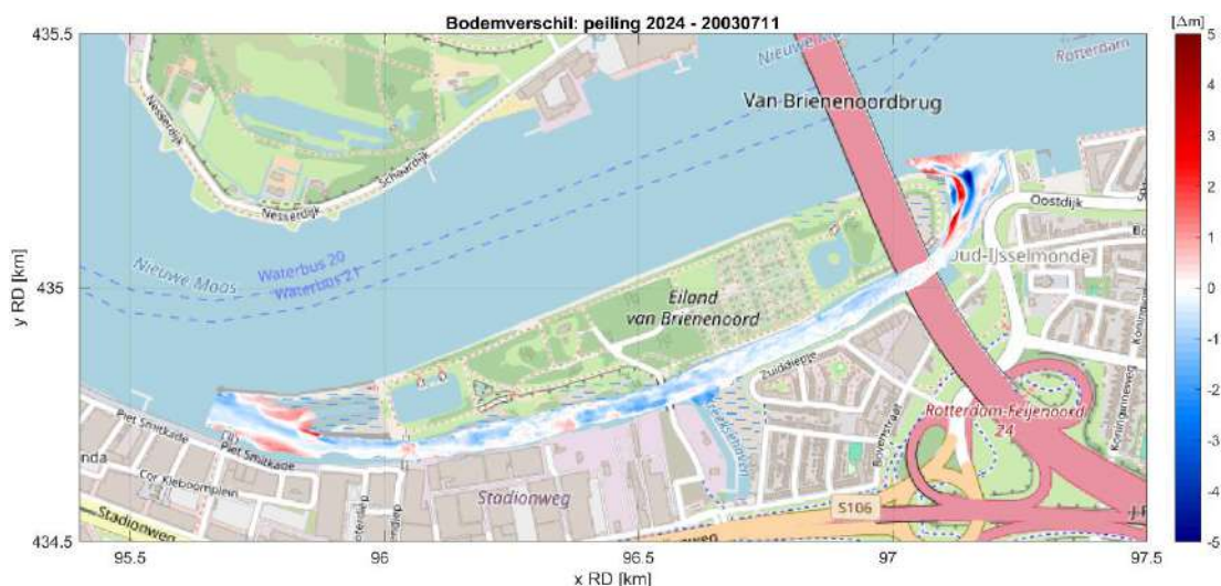
Figuur 4.23: Bodemverschil tussen bodempeilingen uit 2024 en 2003.
