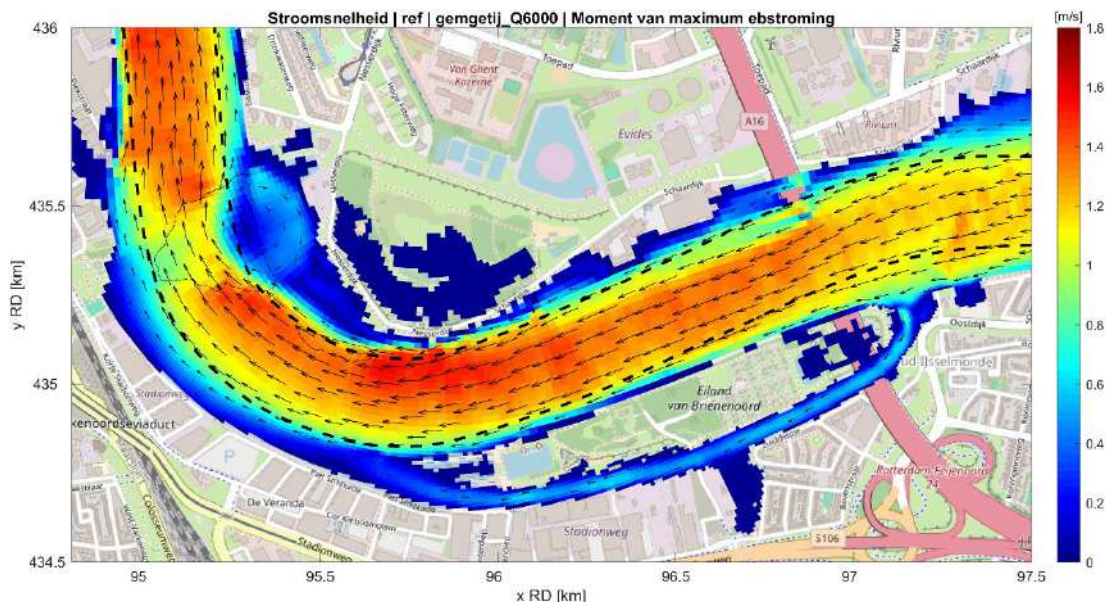
Fig. C.10: Stroomveld in de referentiesituatie tijdens maximale ebstroom bij hoge rivierafvoer (6000 m 3 /s) en gemiddeld getij.
