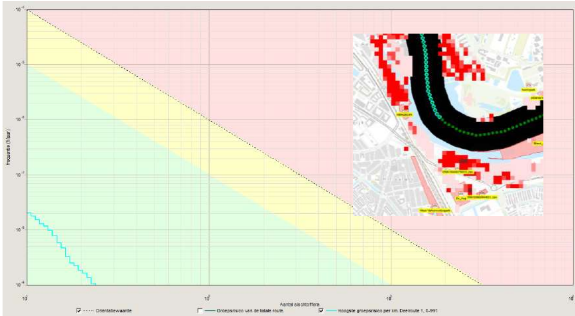
Figuur 9-3: fN-curve en maatgevende kilometer huidige situatie
