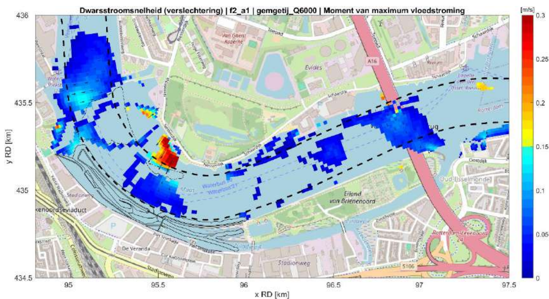
Fig. D.18: Stroomsnelheid dwars op de randen van de vaargeul voor de situatie met getijdenpark (fase 2) tijdens maximale ebstroom bij hoge rivierafvoer ( 6000 \text{ m}^3/\text{s} ) en gemiddeld getij. Alleen cellen met verhoging ten opzichte van de referentiesituatie zijn weergegeven. De gebieden van het getijdenpark en het Zuiddiepje zijn hier buiten beschouwing gelaten.
