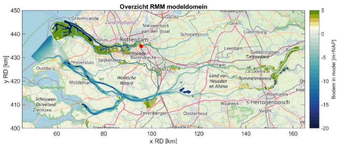
Figuur 3.1: Overzicht van het modeldomein van het gebruikte Rijn-Maasmonding D-HYDRO model. De projectlocatie van het getijdenpark is weergegeven met het rode bolletje.
