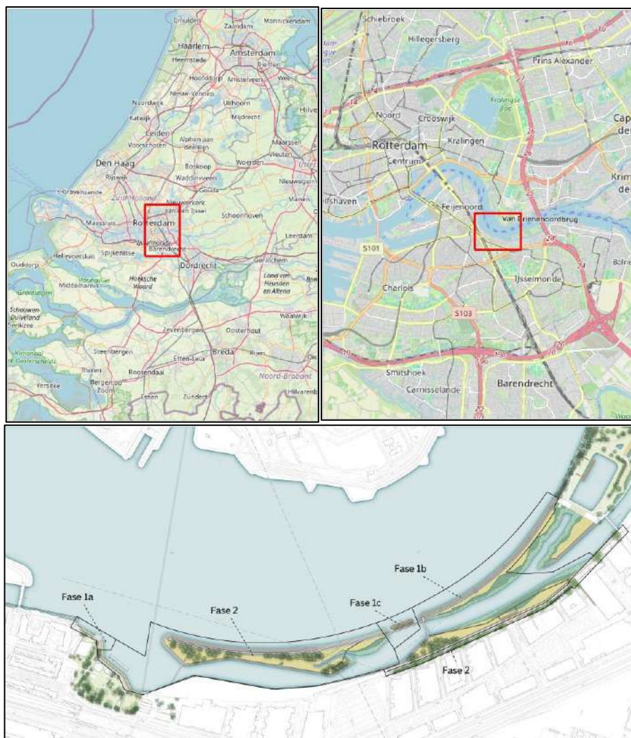
Figuur 1.1: Projectlocatie van het getijdenpark bij het Eiland van Brienenoord. In de onderste figuur is het ontwerp van het getijdenpark weergegeven.
