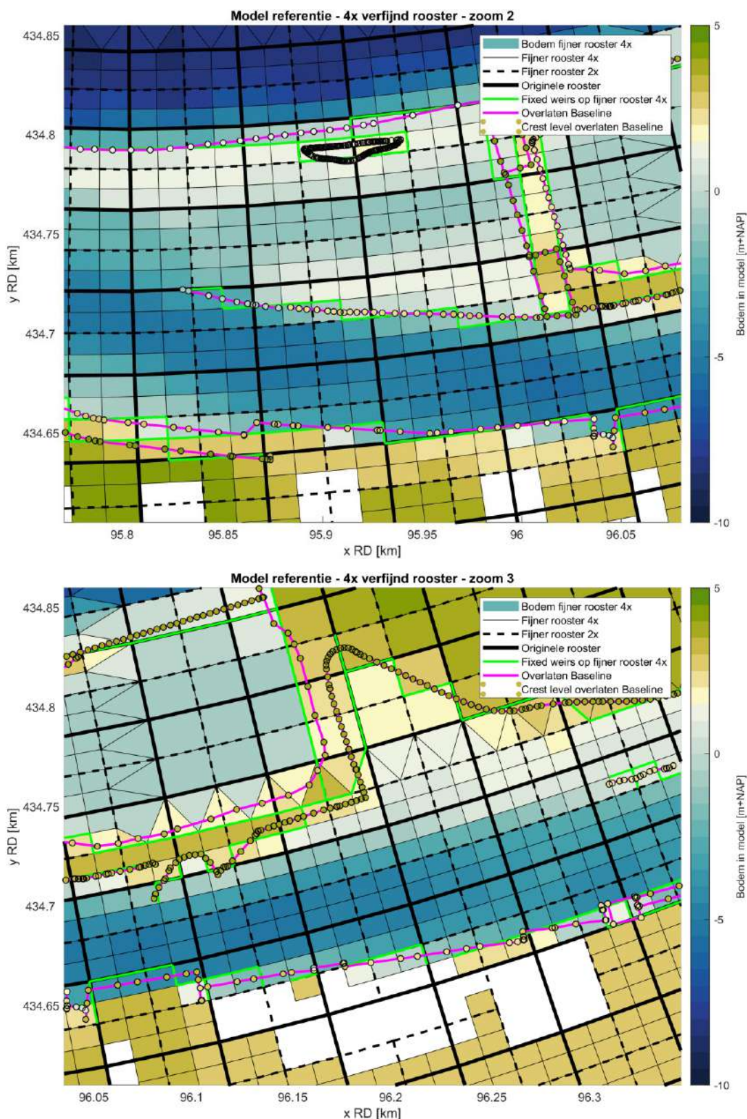
Figuur B.3: Projecties van de Baseline schematisatie van de referentiesituatie op het 4x verfijnde rooster, zie Figuur B.1 voor de locatie van de zooms. De drie verschillende roosters zijn weergegeven met de zwarte (stippel)lijnen, de kleurschaal geeft de bodemligging in het 4x verfijnde rooster weer, de groene lijnen tonen de locaties van de gesnappede overlatten in het D-HYDRO model en de magentalijnen bevatten de locaties van de overlatten vanuit Baseline, met in de gekleurde bolletjes de kruinhoogtes van deze overlatten.
