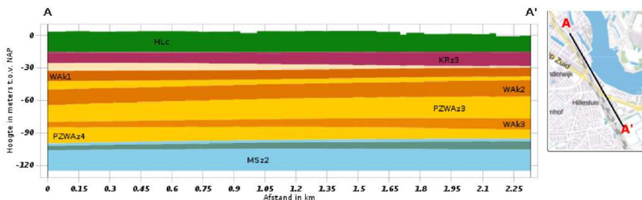
Figuur 2-3: Schematisatie bodemopbouw REGIS II v2.2.2.
