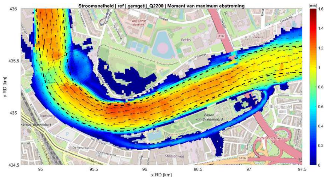
Fig. C.1: Stroomveld in de referentiesituatie tijdens maximale ebstroom bij mediane rivierafvoer (2200 m 3 /s) en gemiddeld getij.
