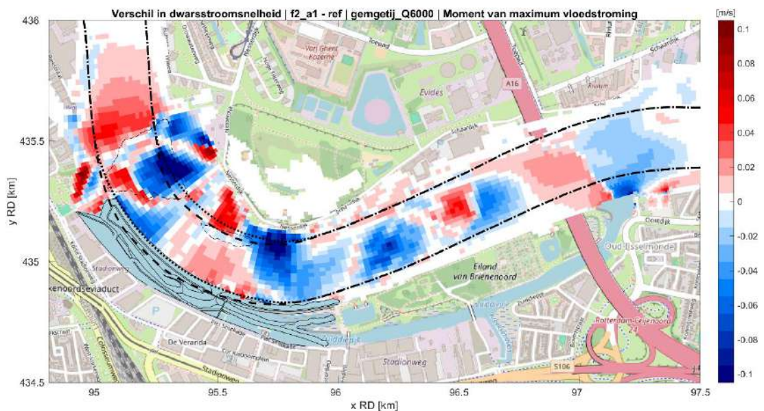
Fig. D.16: Verschil in stroomsnelheid dwars op de randen van de vaargeul tussen de referentiesituatie en de situatie met getijdenpark (fase 2) tijdens maximale vloedstroom bij hoge rivierafvoer ( 6000 \text{ m}^3/\text{s} ) en gemiddeld getij. Rood geeft een toename in dwarsstroomsnelheid t.g.v. het getijdenpark weer, blauw een afname in dwarsstroomsnelheid. De gebieden van het getijdenpark en het Zuiddiepje zijn hier buiten beschouwing gelaten.
