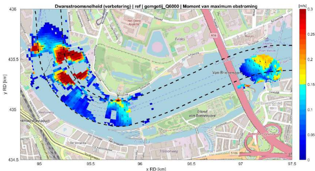
Fig. D.19: Stroomsnelheid dwars op de randen van de vaargeul voor de referentiesituatie tijdens maximale ebstroom bij hoge rivierafvoer ( 6000 \text{ m}^3/\text{s} ) en gemiddeld getij. Alleen cellen met verbetering door het getijdenpark ten opzichte van de referentiesituatie zijn weergegeven. De gebieden van het getijdenpark en het Zuiddiepje zijn hier buiten beschouwing gelaten.
