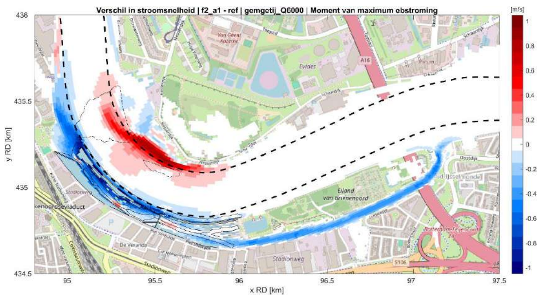
Figuur 4.7: Verschil in stroomsnelheid tussen de referentiesituatie en de situatie met getijdenpark (fase 2) tijdens maximale ebstroom bij hoge rivierafvoer ( 6000 \text{ m}^3/\text{s} ) en gemiddeld getij. Rood geeft een toename in stroomsnelheid t.g.v. het getijdenpark weer, blauw een afname in stroomsnelheid.
