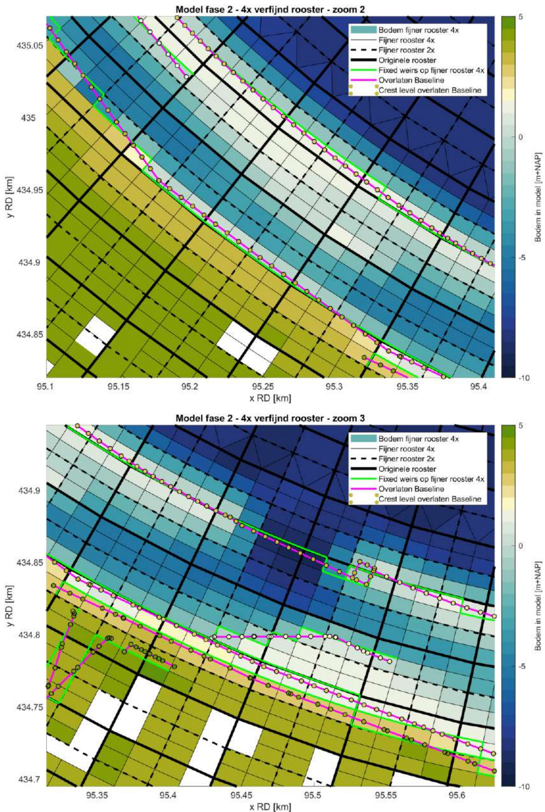
Figuur B.8: Projecties van de Baseline schematisatie van het ontwerp van het getijdenpark op het 4x verfijnde rooster, zie Figuur B.6 voor de locatie van de zooms. De drie verschillende roosters zijn weergegeven met de zwarte (stippell)lijnen, de kleurenschaal geeft de bodemligging in het 4x verfijnde rooster weer, de groene lijnen tonen de locaties van de gesnappede overlaten in het D-HYDRO model en de magentalijnen bevatten de locaties van de overlaten vanuit Baseline, met in de gekleurde bolletjes de kruinhoogtes van deze overlaten.
