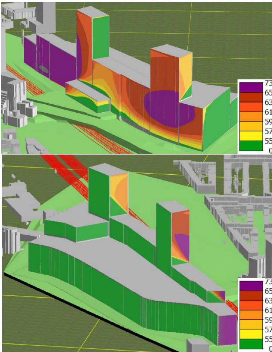
Figuur 5.14.3 Geluid spoorwegen zonder maatregelen (Bron: Akoestisch onderzoek DGMR, M.2024.0597.04.R001)
