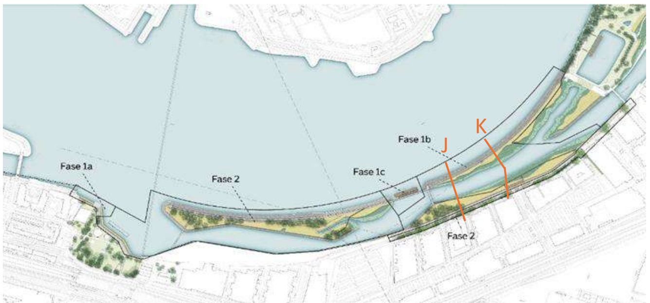
Figuur 4.3 Fases aanleg Getijdenpark Feijenoord. De dwarsdoorsnedes J en K zijn verderop opgenomen.
