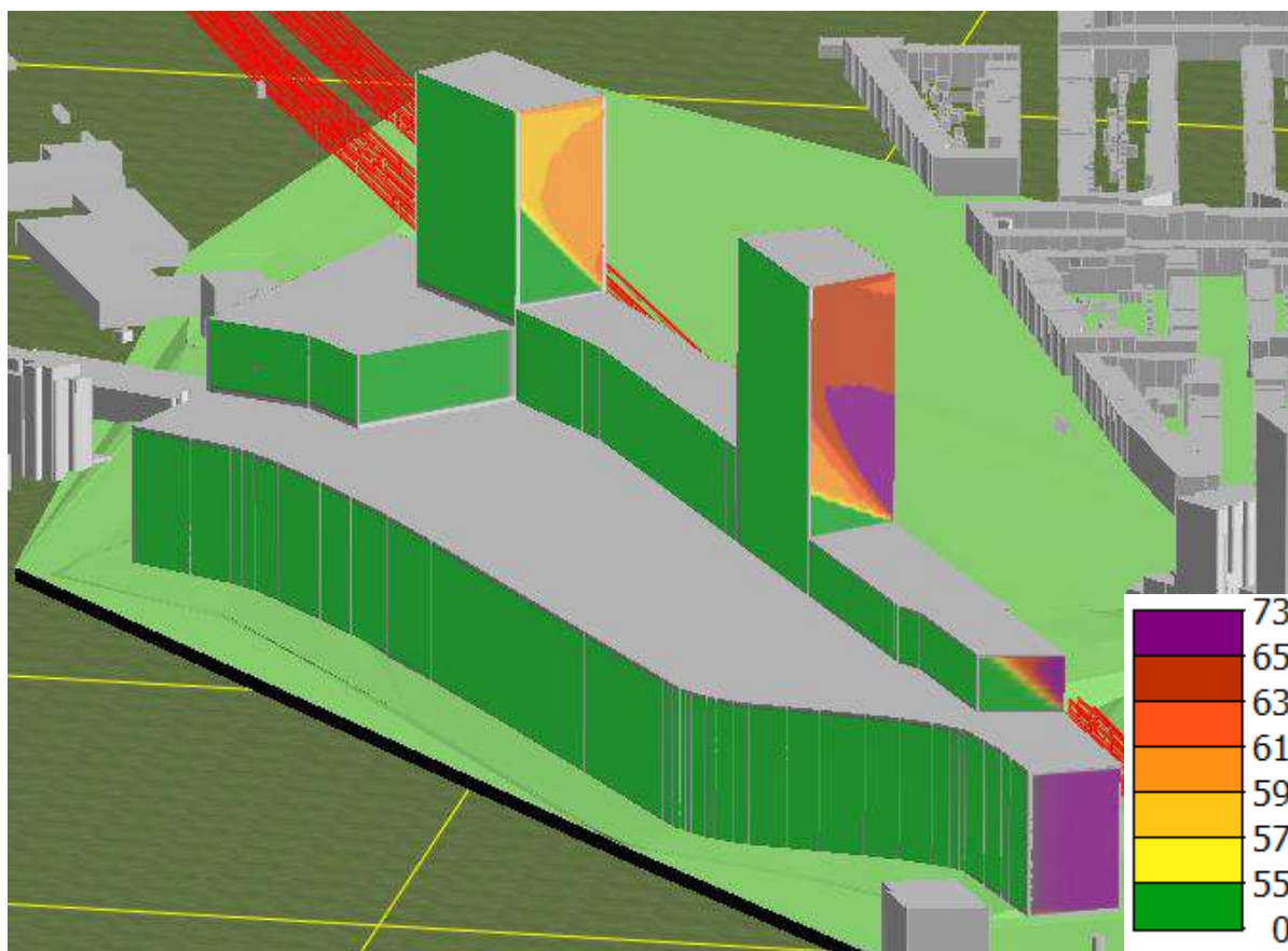
figuur 8: geluid spoorwegen zonder maatregelen
