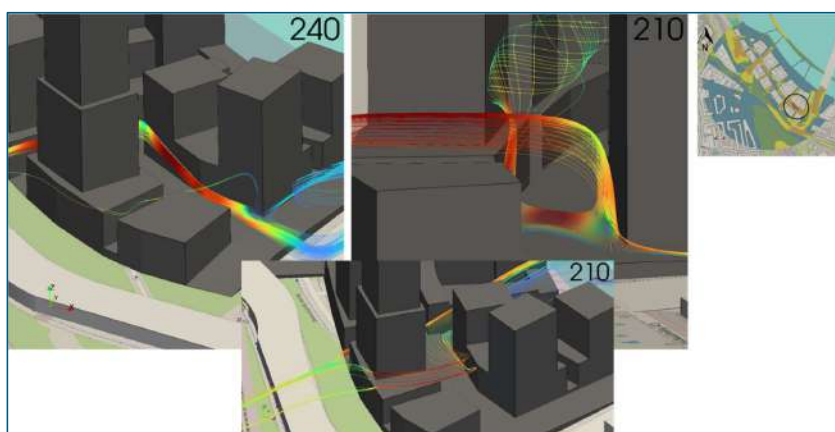
Figuur 4-8: Windstroming bij zuidelijke torens, voor de windrichting westzuidwest en west.
