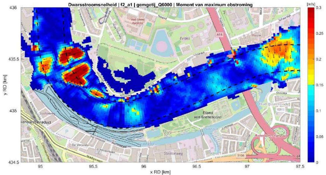
Fig. D.13: Strooming dwars op de randen van de vaargeul in de situatie met getijdenpark (fase 2) tijdens maximale ebstroom bij hoge rivierafvoer ( 6000 \text{ m}^3/\text{s} ) en gemiddeld getij. De gebieden van het getijdenpark en het Zuiddiepje zijn hier buiten beschouwing gelaten.
