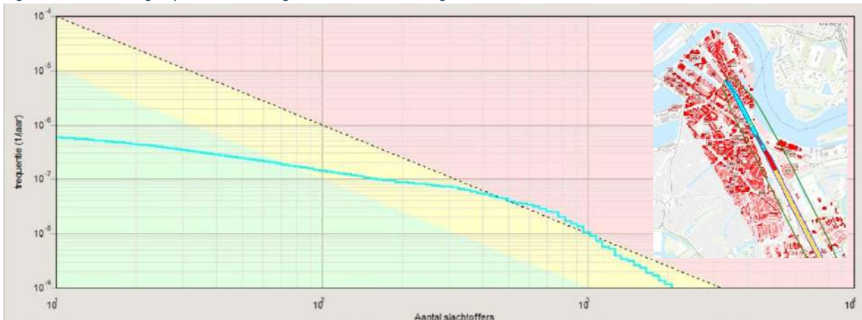
Figuur 9-1: FN-curve groepsrisico en maatgevende kilometer huidige situatie
