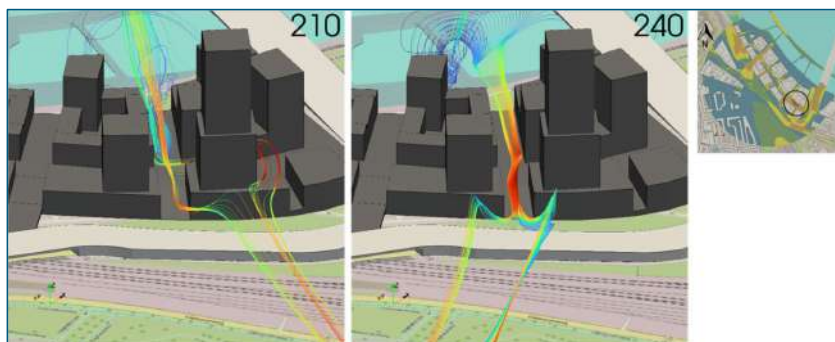
Figuur 4-7: Windstroming bij de zuidelijke verbinding richting de Maas voor de windrichting westzuidwest en west.
