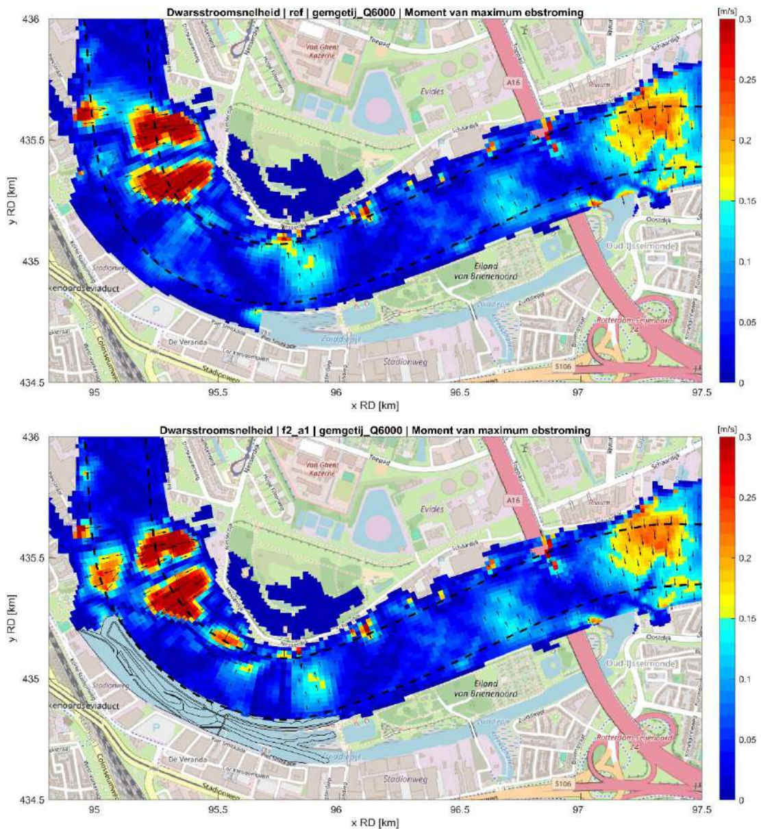
Figuur 4.11: Strooming dwars op de randen van de vaargeul in de referentiesituatie (boven) en de situatie met getijdenpark (fase 2, onder) tijdens maximale ebstroom bij hoge rivierafvoer ( 6000 \text{ m}^3/\text{s} ) en gemiddeld getij. De gebieden van het getijdenpark en het Zuiddiepe zijn hier buiten beschouwing gelaten.
