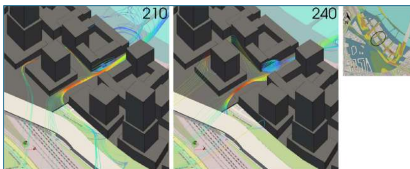
Figuur 4-6: Windstroming bij de middelste verbinding richting de Maas, voor de windrichting westzuidwest en west.
