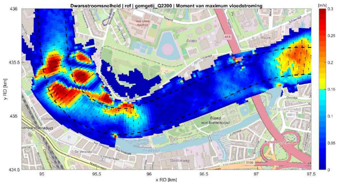
Fig. D.2: Strooming dwars op de randen van de vaargeul in de referentiesituatie tijdens maximale vloedstroom bij mediane rivierafvoer (2200 m 3 /s) en gemiddeld getij. Het gebied van het Zuiddiepe zijn hier buiten beschouwing gelaten.
