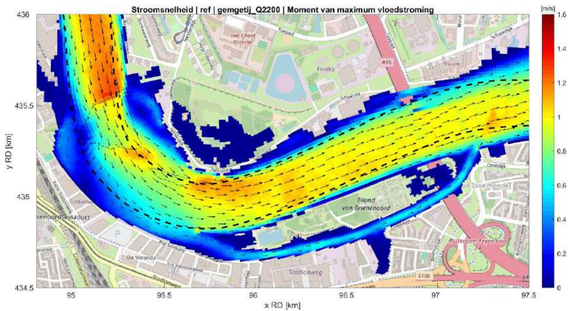
Figuur 4.8: Stroomveld in de Nieuwe Maas in de referentiesituatie tijdens maximale vloedstroom bij mediane rivierafvoer ( 2200 \text{ m}^3/\text{s} ) en gemiddeld getij.
