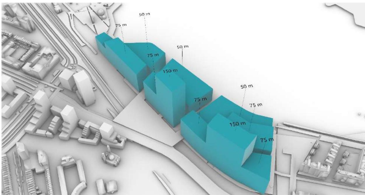
Figuur 4 Getoetst model voor bezonning, maximale bouwvolumes inclusief indicatie maximale bouwhoogtes.
