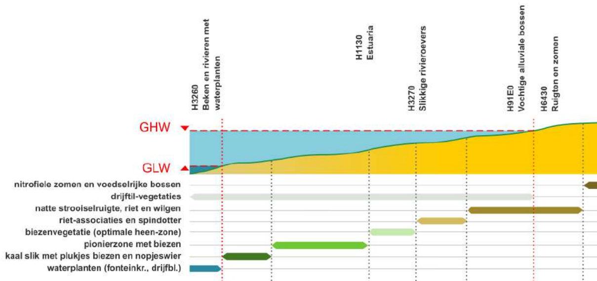
Figuur 3.3. Opbouw van slikken en schorren met specifieke vegetatiezones in een zoet getijdenwater zoals in het studiegebied (naar Zonneveld 1960).
