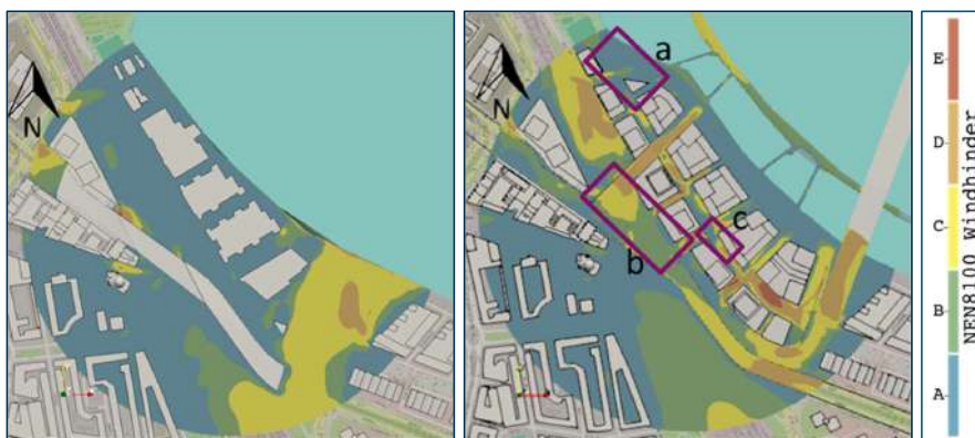
Figuur 4-1: Grafische weergave van het windklimaat voor de activiteit “langdurig zitten”, voor de huidige (links) en nieuwe (rechts) situatie. De paarse kaders binnen stippellijnen geven de pleinen aan.
