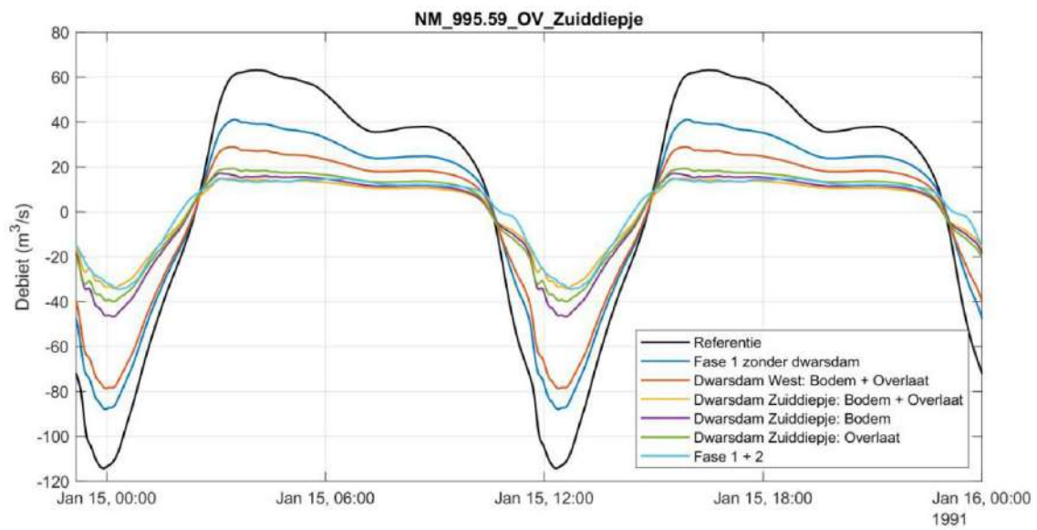
Figuur 4.11. Vergelijking van het debiet in het Zuiddiepje voor verschillende simulaties van fase 1 met en zonder dwarsdammen en voor fase 1 + 2 (Svašek Hydraulics, 2025).
