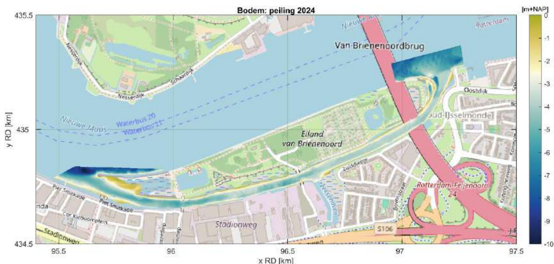
Figuur 4.22: Bodempeiling 2024 van het Zuiddiepje.
