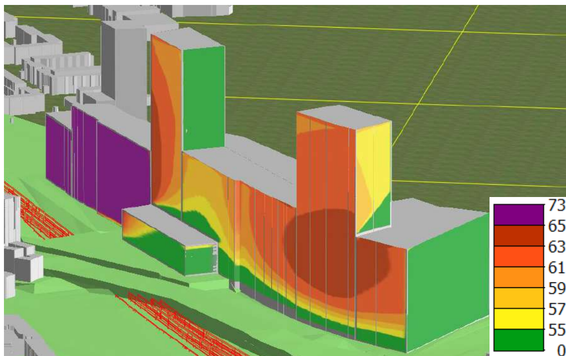
figuur 9: geluid hoofdspoorwegen met potentiële GPP-reductie 2 dB
