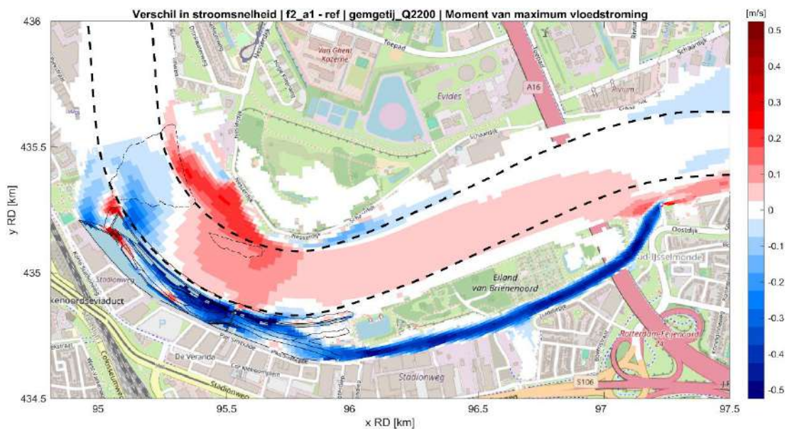
Figuur 4.10: Verschil in stroomsnelheid tussen de referentiesituatie en de situatie met getijdenpark (fase 2) tijdens maximale vloedstroom bij mediane rivierafvoer ( 2200 \text{ m}^3/\text{s} ) en gemiddeld getij. Rood geeft een toename in stroomsnelheid t.g.v. het getijdenpark weer, blauw een afname in stroomsnelheid.
