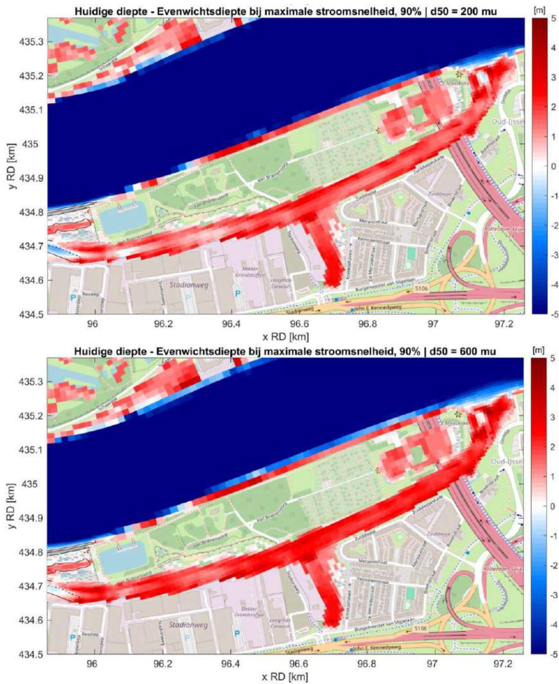
Figuur 4.13. Huidige diepte minus evenwichtsdiepte voor fase 1 + fase 2 in het Zuiddiepje bij verschillende korreldiameters (200 \mu of 600 \mu ). Er treed sedimentatie op in het Zuiddiepje van 0 tot enkele meters (rode kleur).
