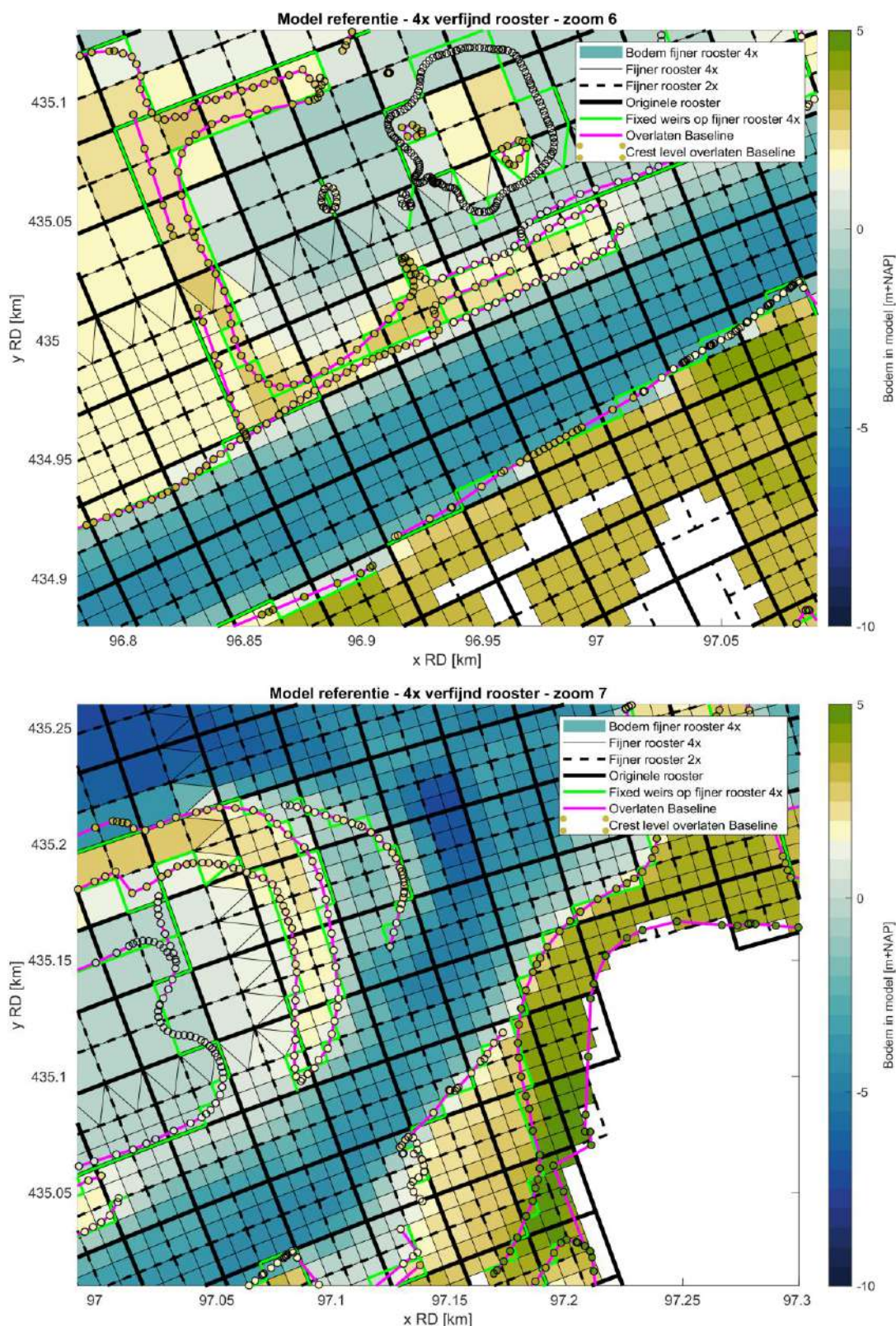
Figuur B.5: Projecties van de Baseline schematisatie van de referentiesituatie op het 4x verfijnde rooster, zie Figuur B.1 voor de locatie van de zooms. De drie verschillende roosters zijn weergegeven met de zwarte (stippel)lijnen, de kleurschaal geeft de bodemligging in het 4x verfijnde rooster weer, de groene lijnen tonen de locaties van de gesnappede overlaten in het D-HYDRO model en de magentalijnen bevatten de locaties van de overlaten vanuit Baseline, met in de gekleurde bolletjes de kruinhoogtes van deze overlaten.
