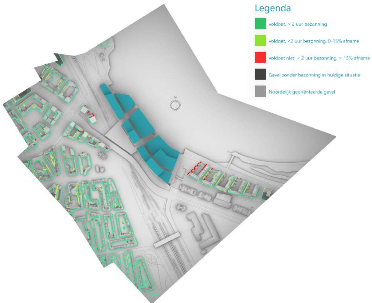
Figuur 5 Bezinning op de gevels in het te onderzoek plangebied op de 15.000 toetspunten (exclusief noord georiënteerde gevels)
