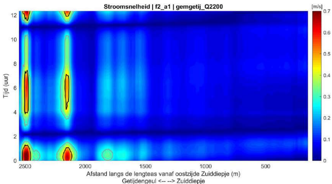
Figuur 4.28: Stroomsnelheid over de tijd (getijcyclus) voor fase 2 van het getijdenpark langs de lengteas van het Zuiddiepje (0 – 1400m) en het getijdenpark (1400 – 2580m), met contouren van de kritische stroomsnelheid 0,28m/s (grijze lijn) en 0,45 m/s (zwarte lijn).
