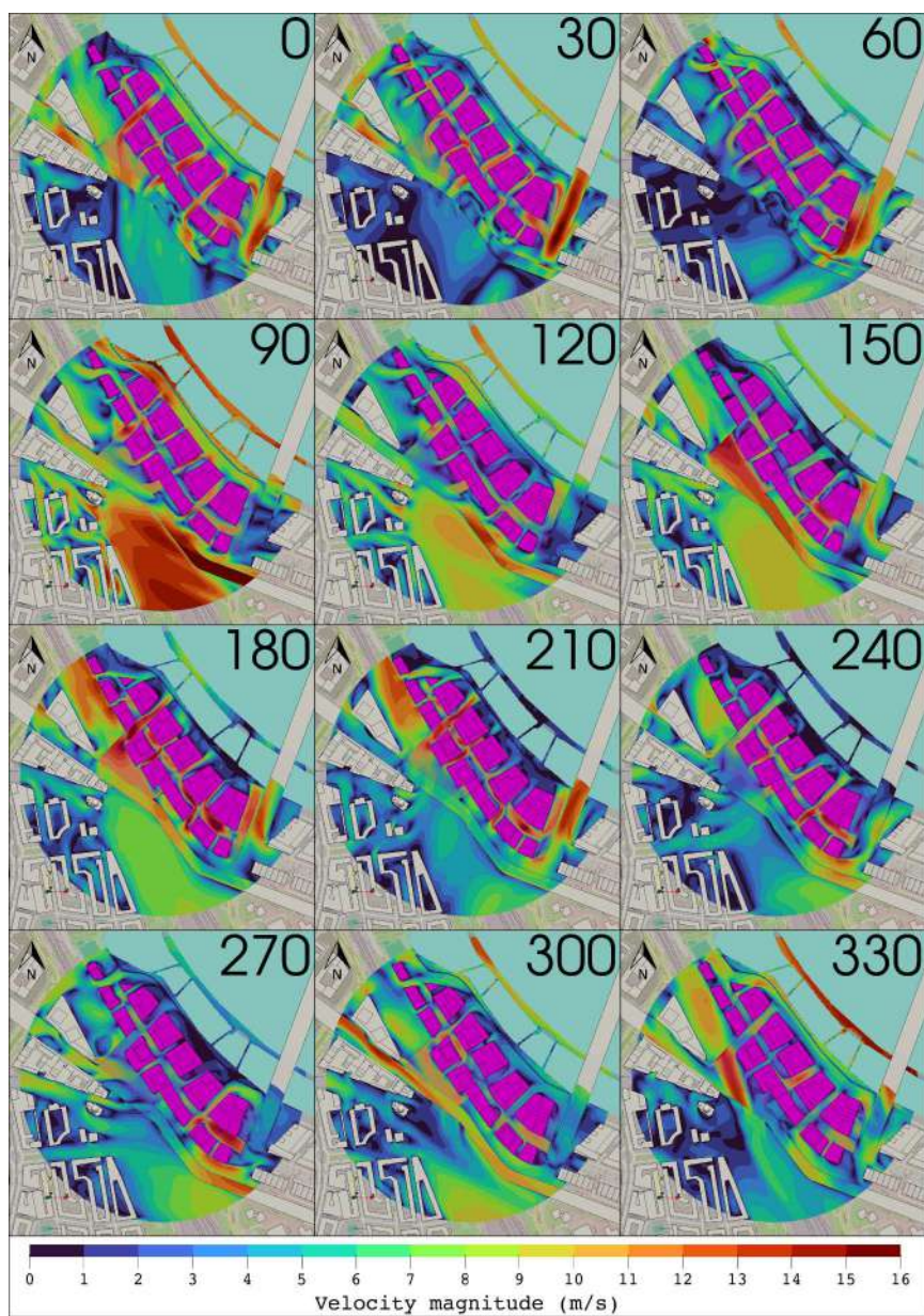
Figuur Bijlage D-2: Overzicht windsnelheidskaart op 1,75m hoogte voor alle 12 windrichtingen, nieuwe situatie
