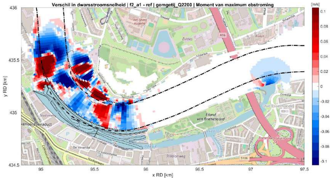
Fig. D.5: Verschil in stroomsnelheid dwars op de randen van de vaargeul tussen de referentiesituatie en de situatie met getijdenpark (fase 2) tijdens maximale ebstroom bij mediane rivierafvoer (2200 m 3 /s) en gemiddeld getij. Rood geeft een toename in dwarsstroomsnelheid t.g.v. het getijdenpark weer, blauw een afname in dwarsstroomsnelheid. De gebieden van het getijdenpark en het Zuiddiepe zijn hier buiten beschouwing gelaten.
