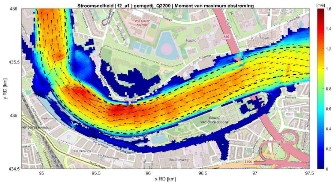
Fig. C.4: Stroomveld in de situatie met getijdenpark (fase 2) tijdens maximale ebstroom bij mediane rivierafvoer ( 2200 \text{ m}^3/\text{s} ) en gemiddeld getij.
