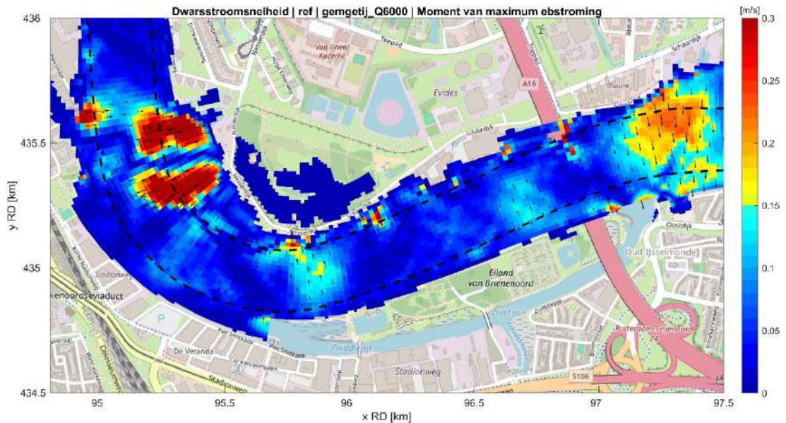
Fig. D.11: Strooming dwars op de randen van de vaargeul in de referentiesituatie tijdens maximale ebstroom bij hoge rivierafvoer (6000 m 3 /s) en gemiddeld getij. Het gebied van het Zuiddiepje zijn hier buiten beschouwing gelaten.
