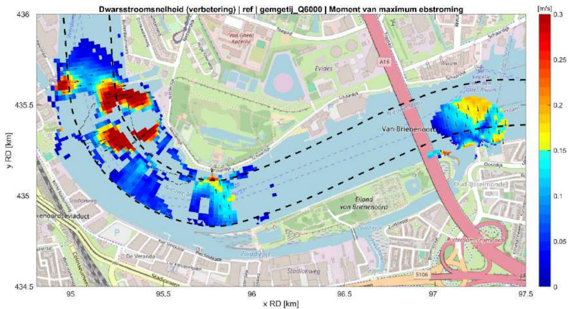
Figuur 4.14: Stroming dwars op de randen van de vaargeul in de referentiesituatie tijdens maximale ebstroom bij hoge rivierafvoer (6000 m 3 /s) en gemiddeld getij. Alleen cellen met verbetering door het getijdenpark ten opzichte van de referentiesituatie zijn weergegeven. De gebieden van het Zuiddiepje is hier buiten beschouwing gelaten.
