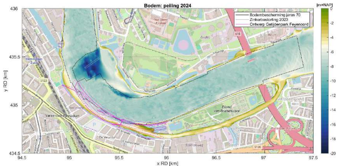
Figuur 4.15: Bodempeiling 2024 inclusief ligging van bodembescherming uit jaren 70 (zwart omlijnd), zinkerbestorting uit 2023 (grijs omlijnd) en het ontwerp van het Getijdenpark Feyenoord, fase 2 (magenta lijnen).
