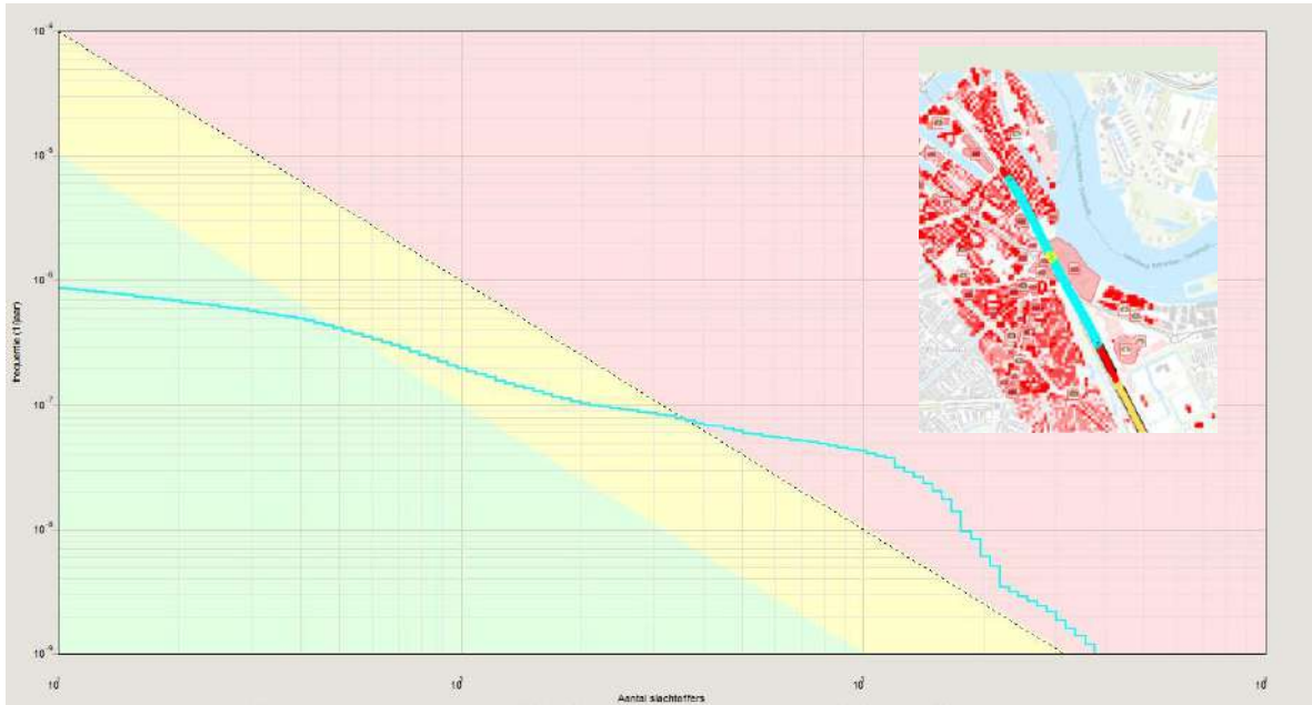
Figuur 9-2: FN-curve groepsrisico en maatgevende kilometer toekomstige situatie
