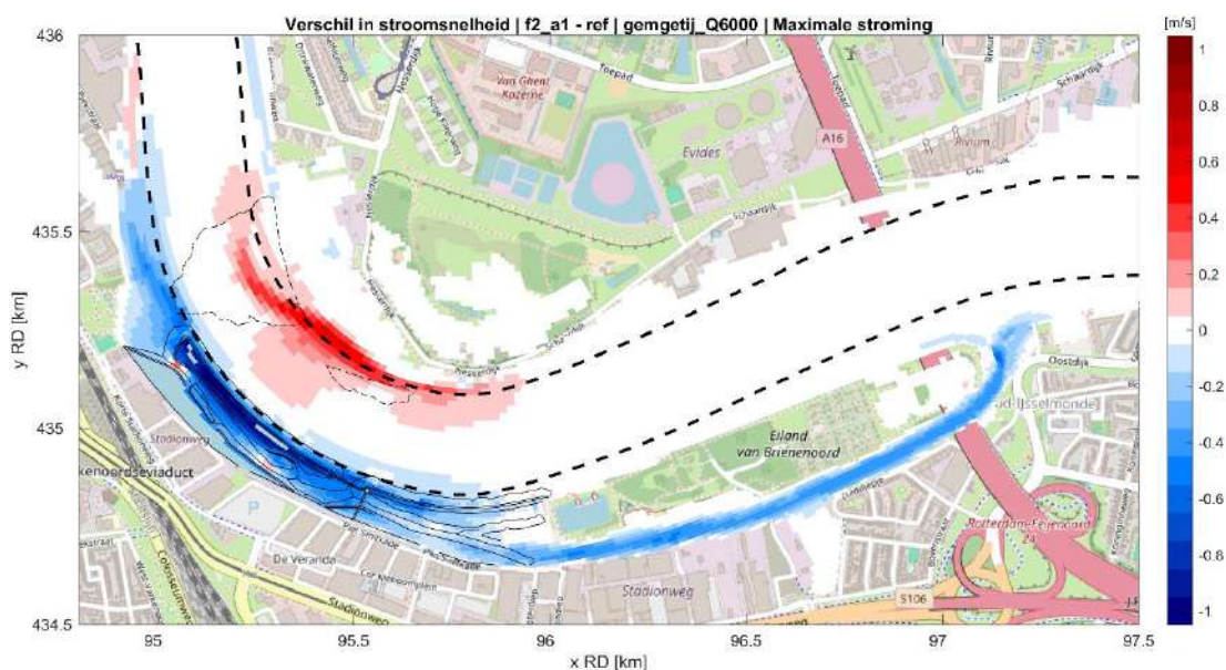
Fig. C.18: Verschil in maximale stroomsnelheid tussen de referentiesituatie en de situatie met getijdenpark (fase 2) tijdens de gehele simulatie met hoge rivierafvoer ( 6000 \text{ m}^3/\text{s} ) en gemiddeld getij. Rood geeft een toename in stroomsnelheid t.g.v. het getijdenpark weer, blauw een afname in stroomsnelheid.
