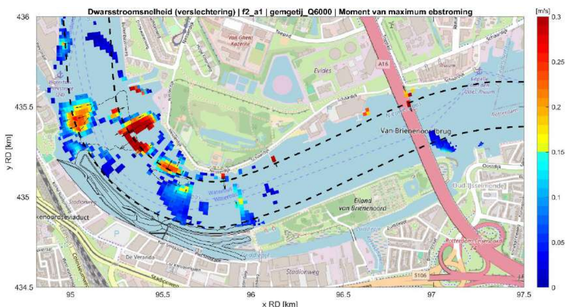
Figuur 4.13: Strooming dwars op de randen van de vaargeul in de situatie met getijdenpark (fase 2) tijdens maximale ebstroom bij hoge rivierafvoer ( 6000 \text{ m}^3/\text{s} ) en gemiddeld getij. Alleen cellen met verhoging ten opzichte van de referentiesituatie zijn weergegeven. De gebieden van het getijdenpark en het Zuiddiepje zijn hier buiten beschouwing gelaten.
