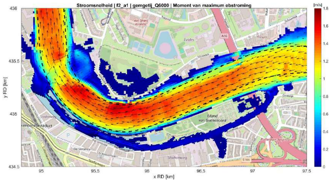
Figuur 4.6: Stroomveld in de Nieuwe Maas in de situatie met getijdenpark (fase 2) tijdens maximale ebstroom bij hoge rivierafvoer ( 6000 \text{ m}^3/\text{s} ) en gemiddeld getij.
