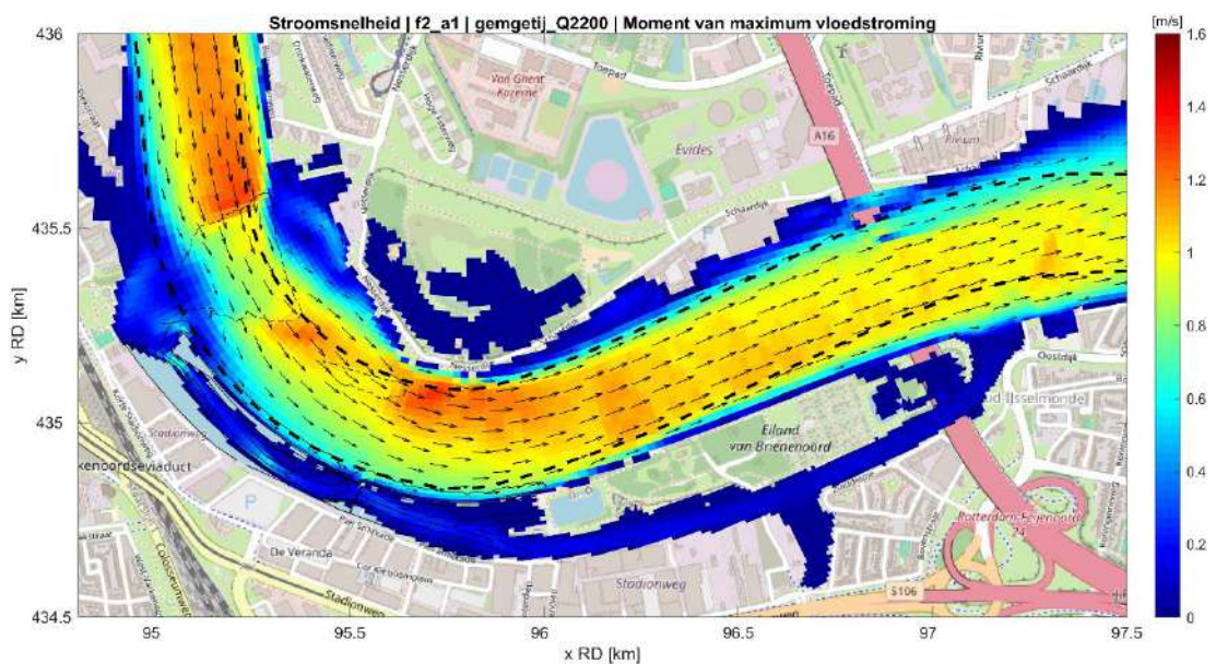
Figuur 4.9: Stroomveld in de Nieuwe Maas in de situatie met getijdenpark (fase 2) tijdens maximale vloedstroom bij mediane rivierafvoer ( 2200 \text{ m}^3/\text{s} ) en gemiddeld getij.
