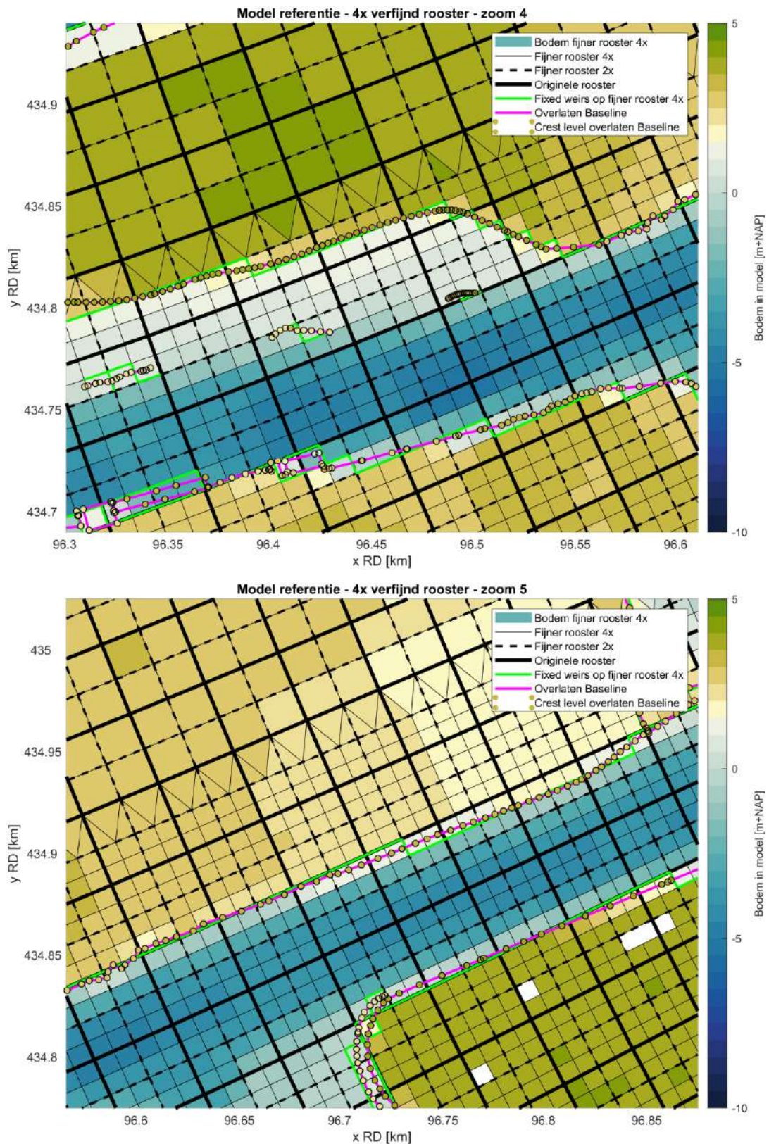
Figuur B.4: Projecties van de Baseline schematisatie van de referentiesituatie op het 4x verfijnde rooster, zie Figuur B.1 voor de locatie van de zooms. De drie verschillende roosters zijn weergegeven met de zwarte (stippel)lijnen, de kleurschaal geeft de bodemligging in het 4x verfijnde rooster weer, de groene lijnen tonen de locaties van de gesnappede overlaten in het D-HYDRO model en de magentalijnen bevatten de locaties van de overlaten vanuit Baseline, met in de gekleurde bolletjes de kruinhoogtes van deze overlaten.
