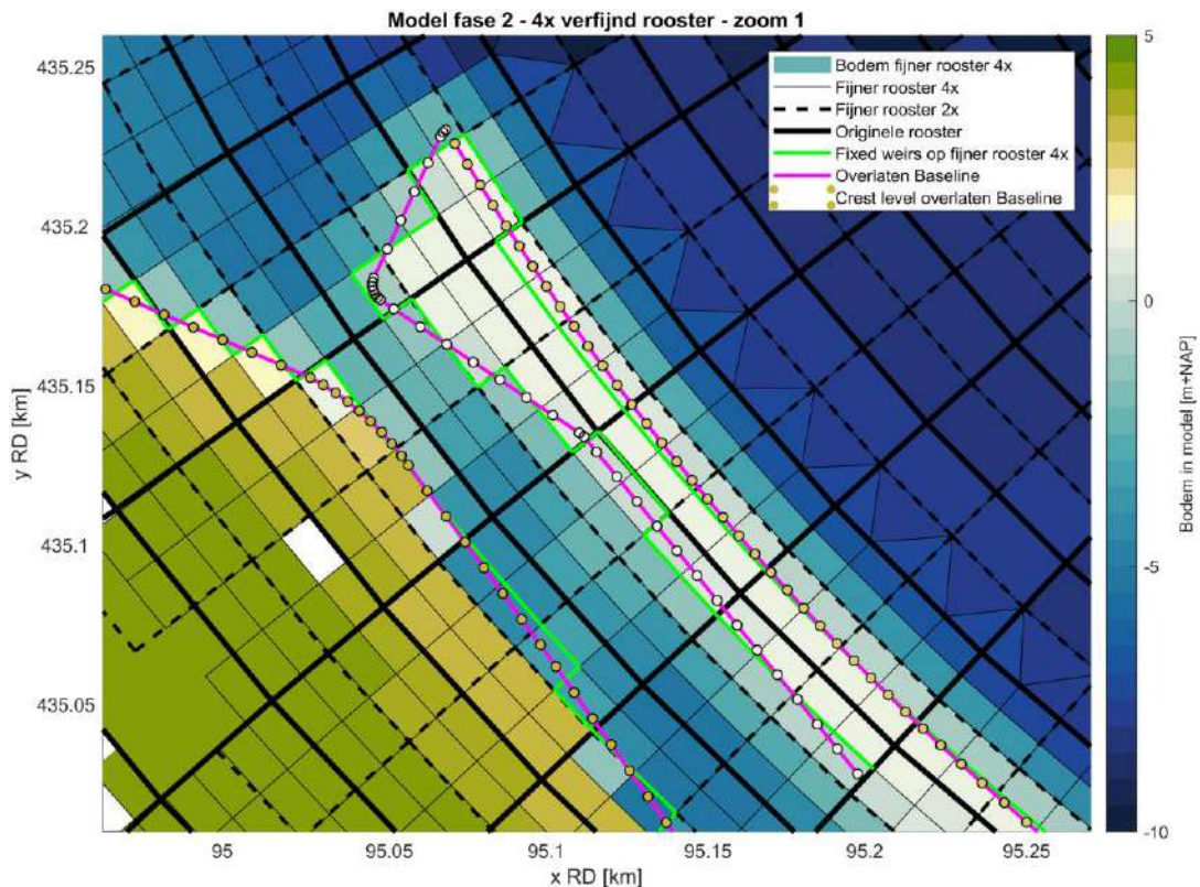
Figuur 3.8: Projectie van de Baseline schematisatie van het ontwerp van het getijdenpark (fase 2) op het 4x verfijnde rooster, zie Figuur B.6 voor de locatie van de zoom. De drie verschillende roosters zijn weergegeven met de zwarte (stippel)lijnen, de kleurschaal geeft de bodemligging in het 4x verfijnde rooster weer, de groene lijnen tonen de locaties van de gesnappede overlaten in het D-HYDRO model en de magentalijnen bevatten de locaties van de overlaten vanuit Baseline, met in de gekleurde bolletjes de kruinhoogtes van deze overlaten.
