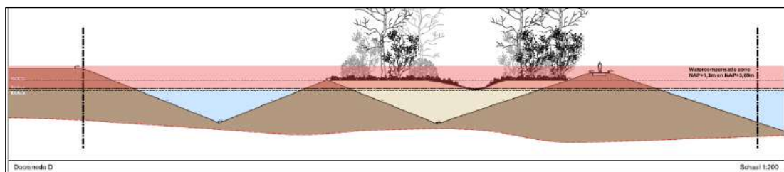
Figuur 4.3: Doorsnede van het getijdenpark met indicatie van gebied voor watercompensatie in rood.
