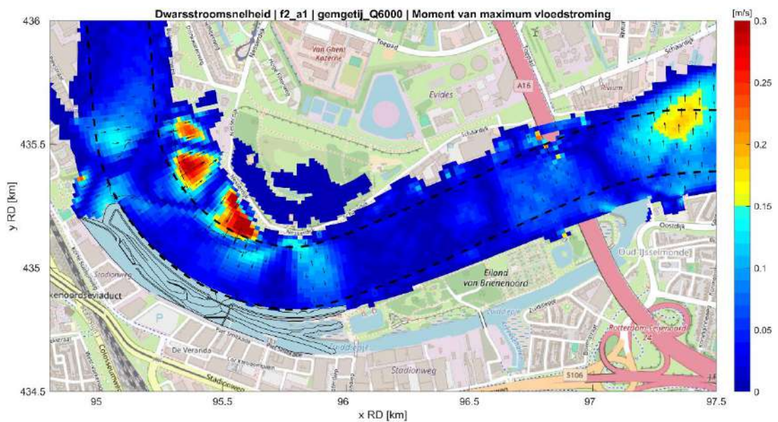
Fig. D.14: Strooming dwars op de randen van de vaargeul in de situatie met getijdenpark (fase 2) tijdens maximale vloedstroom bij hoge rivierafvoer ( 6000 \text{ m}^3/\text{s} ) en gemiddeld getij. De gebieden van het getijdenpark en het Zuiddiepje zijn hier buiten beschouwing gelaten.
