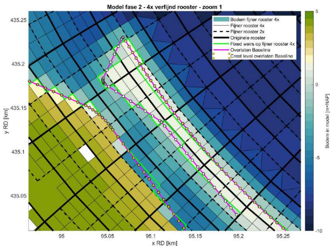
Figuur B.7: Projectie van de Baseline schematisatie van het ontwerp van het getijdenpark op het 4x verfijnde rooster, zie Figuur B.6 voor de locatie van de zoom. De drie verschillende roosters zijn weergegeven met de zwarte (stippel)lijnen, de kleurenschaal geeft de bodemligging in het 4x verfijnde rooster weer, de groene lijnen tonen de locaties van de gesnappede overlatten in het D-HYDRO model en de magentalijnen bevatten de locaties van de overlatten vanuit Baseline, met in de gekleurde bolletjes de kruinhoogtes van deze overlatten.
