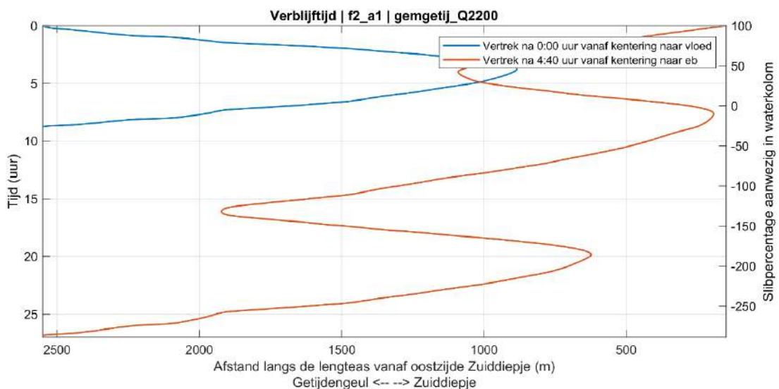
Figuur 4.26: Maximale verblijftijd voor slib en de bijbehorende slibpercentage aanwezig in de waterkolom (rechter y-as) in het getijdenpark (1400 – 2580m) en Zuiddiepje (0 – 1400m) voor fase 2. Voor slib binnenkomend vanaf de westelijke monding (blauwe lijn) tijdens vloed en vanaf de oostelijke monding (rode lijn) tijdens eb.
