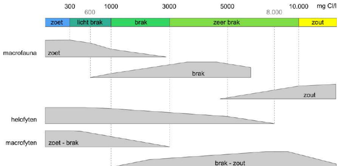
Figuur 2.6. De relatie tussen zoutklasse en de aanwezigheid van flora en fauna (naar Verbeke, 2012; Van Geest, 2022).
