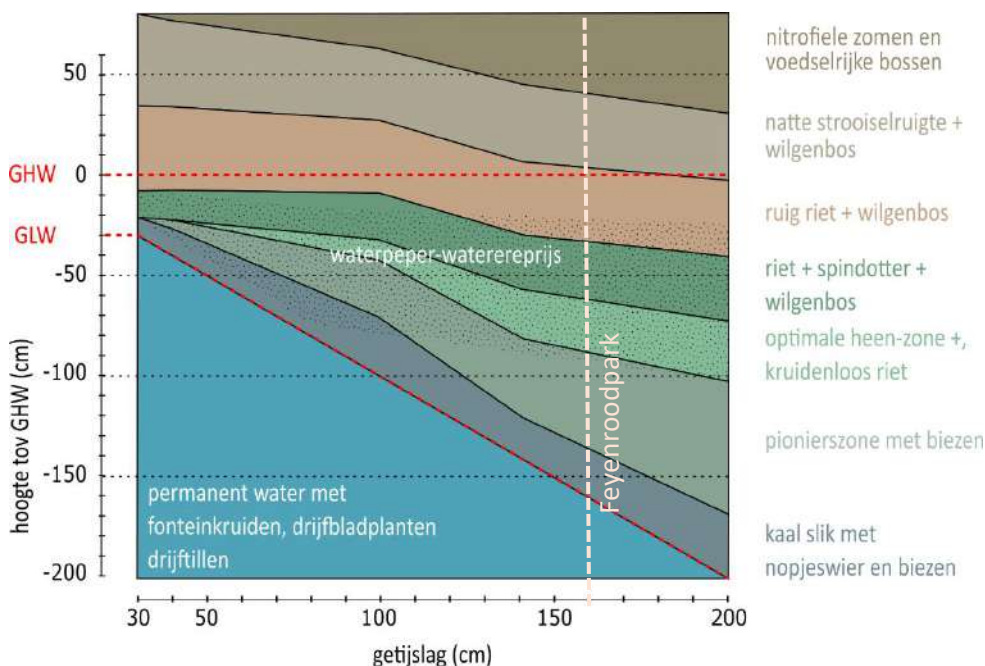
Figuur 2.8. De ligging van kenmerkende vegetatiezones in een zoetwatergetijdenrivier afhankelijk van de getijslag (naar Zonneveld, 1960; 2000). Feyenoordpark heeft een getijslag van ca. 160 cm.
