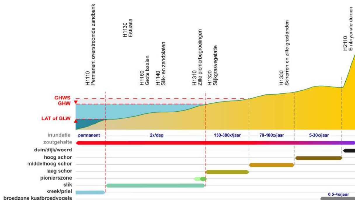
Figuur 3.2. Opbouw van slikken en schorren (wad en kwelder) met specifieke vegetatiezones in een zout getijdenwater zoals gebruikt in de KRW-methodiek voor type O2 (naar Dijkema et al. , 2005; Bouma et al. , 2005).
