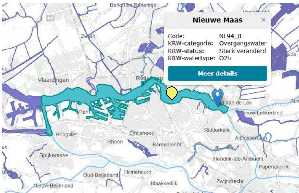
Figuur 3.1 KRW-status van oppervlaktewaterlichaam "Nieuwe Maas" (NL94_8) en de locatie van Getijdenpark Feijenoord (gele pin) (bron: waterkwaliteitsportaal.nl).
