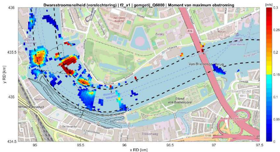
Fig. D.17: Stroomsnelheid dwars op de randen van de vaargeul voor de situatie met getijdenpark (fase 2) tijdens maximale ebstroom bij hoge rivierafvoer ( 6000 \text{ m}^3/\text{s} ) en gemiddeld getij. Alleen cellen met verhoging ten opzichte van de referentiesituatie zijn weergegeven. De gebieden van het getijdenpark en het Zuiddiepje zijn hier buiten beschouwing gelaten.
