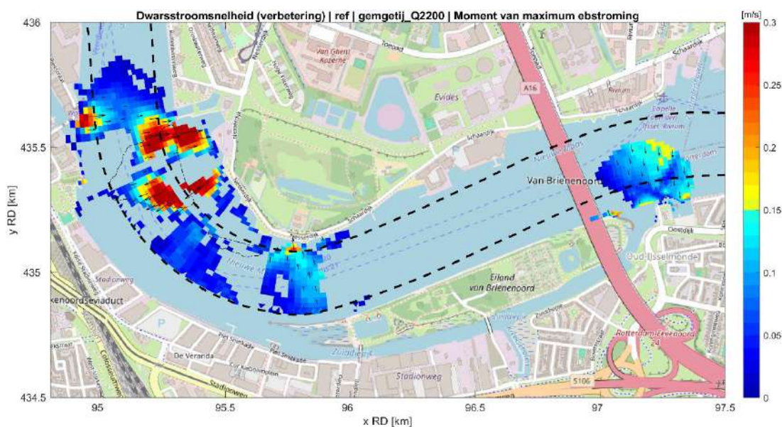
Fig. D.9: Stroomsnelheid dwars op de randen van de vaargeul voor de referentiesituatie tijdens maximale ebstroom bij mediane rivierafvoer ( 2200 \text{ m}^3/\text{s} ) en gemiddeld getij. Alleen cellen met verbetering door het getijdenpark ten opzichte van de referentiesituatie zijn weergegeven. De gebieden van het getijdenpark en het Zuiddiepje zijn hier buiten beschouwing gelaten.
