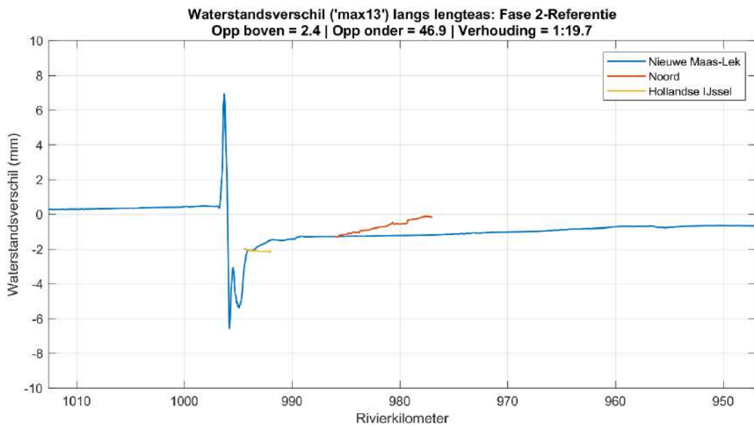
Figuur 4.2: Waterstandsverschil tussen getijdenpark fase 2 en de referentie bij maximale waterstand langs de rivieras in de Nieuwe Maas en Lek (blauw), Noord (rood) en Hollandse IJssel (geel).
