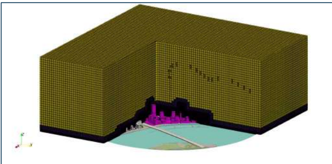
Figuur 3-4: Overzicht rekenrooster, nieuwe situatie
