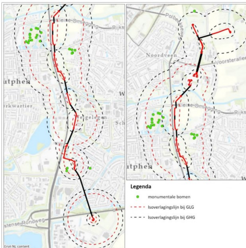
Figuur 4.1: Monumentale bomen binnen en verlagingcontouren (0,5 en 0,05 m) GHG (zwart) en GLG (rood) situatie
