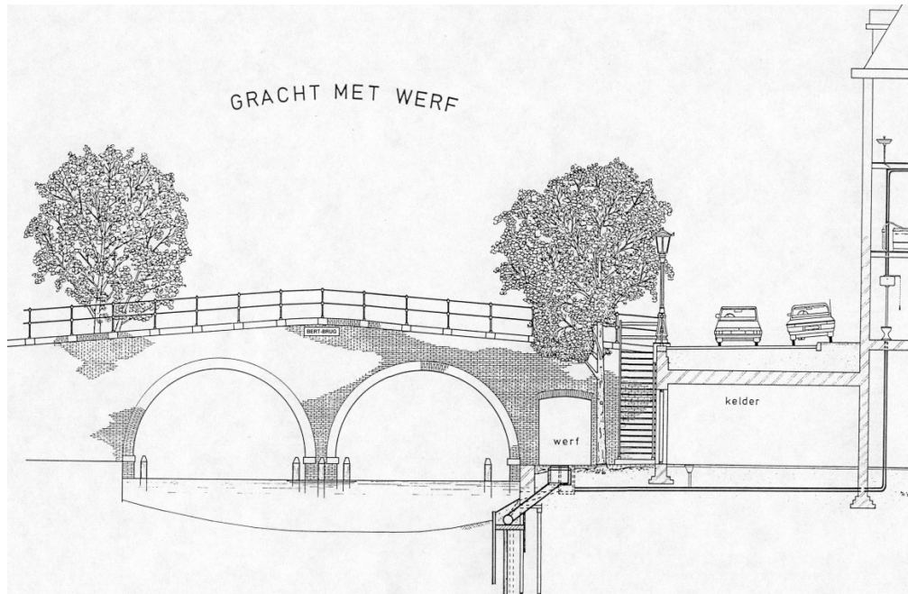
Figuur 4 – schematisatie van het watersysteem. In de jaren '80 is de lozing op het open grachtwater vervangen door een riool die in de grachten, voor de walmuren, zijn aangebracht.
