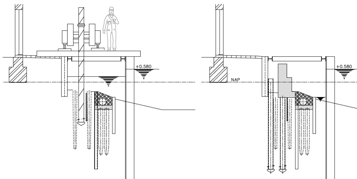
Figuur 9 – ontworpen bouwmethode/bouwfasering Nieuwegracht
