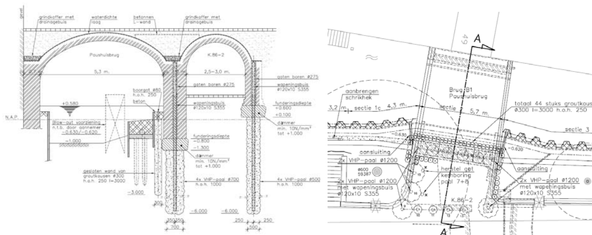
Figuur 46 – uitsnede bestekstekening funderingsherstel brug Paushuize (Kromme Nieuwegrachtbrug 49)
