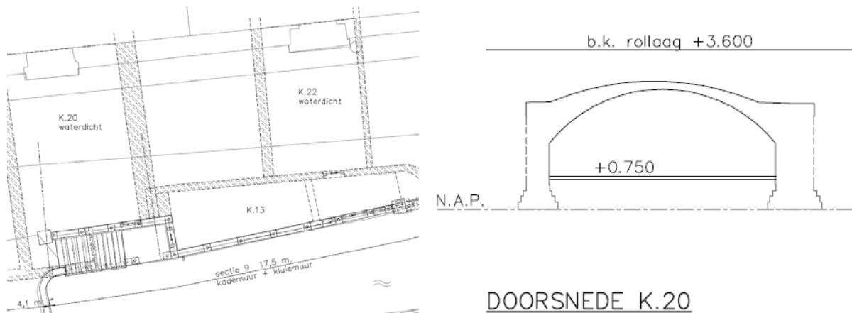
Figuur 22 – [links] reconstructie huidige situatie met de gerealiseerde trap en de schakelruimte in kelder K.13. [rechts] reconstructie van de kelder doorsnede waarop de informatie uit de foto nog niet is verwerkt.
