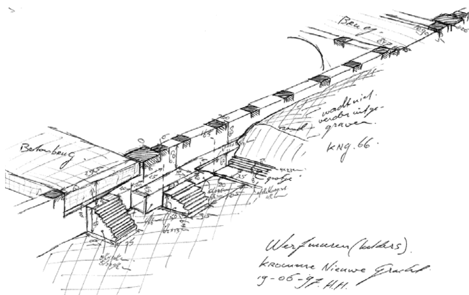
Figuur 33 – in deze schets zijn een aantal trekberen vereeuwigd (getrapte metselwerk steunbeer linksonder).
