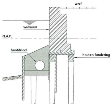
Principeddoorsnede bestaande situatie (type 1)
