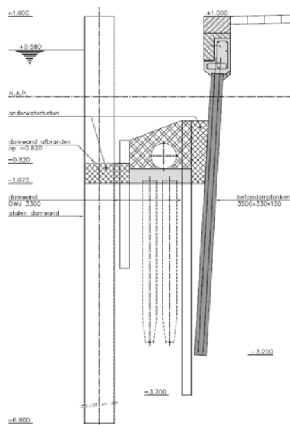
Figuur 2 – werfmuur type 3: betonnen damwand (getekend in eindsituatie met stabilisatie)
