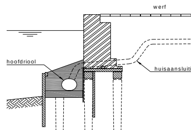
Afb. 5 Oorspronkelijke constructie met rioolkoffer uit de jaren 80
