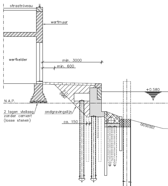
Figuur 15 – uitvoeringsmethode Nieuwegracht met invloedsgebied
