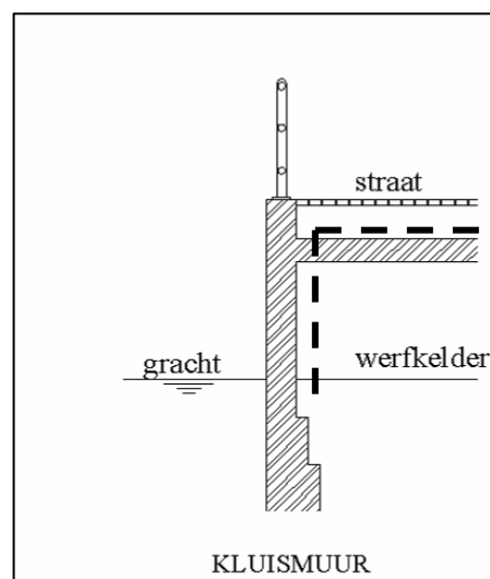
Afb. 3 overzicht kluismuur
