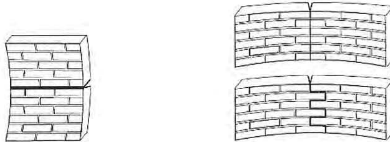
a) bezwijkvlak evenwijdig aan lintvoegen, f_{xk1}
