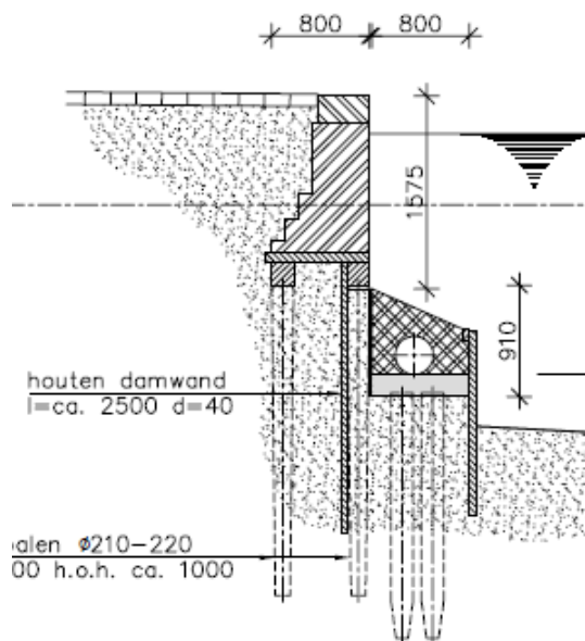
Afbeelding 1 – Walmuurconstructie type I
