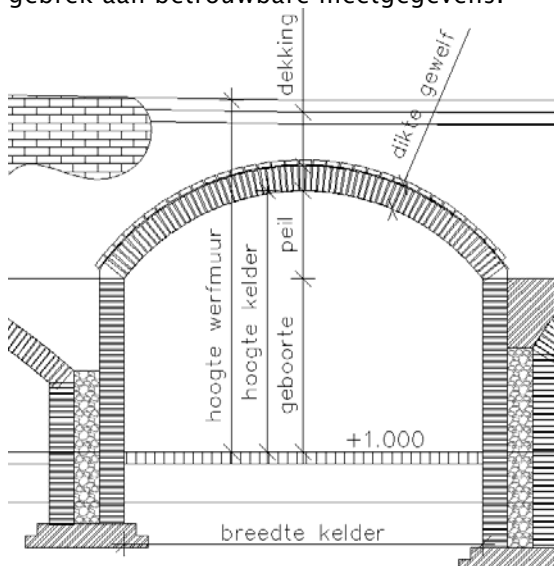
Figuur 4 - Schematische doorsnede kelder
