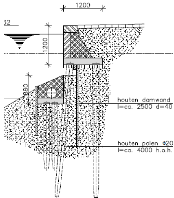
Afbeelding 2 – Walmuurconstructie type II
