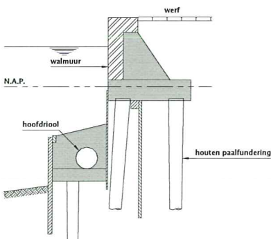
Principeddoorsnede bestaande situatie (type 2)
