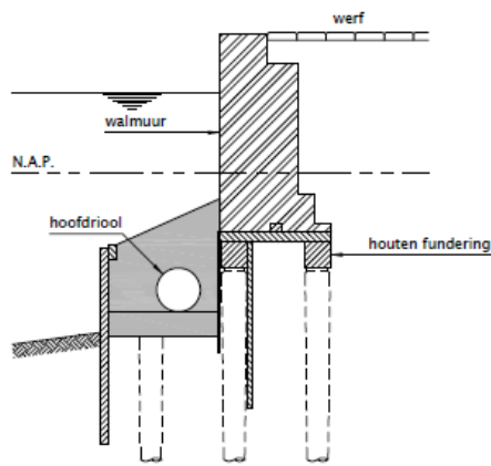
Principeddoorsnede bestaande situatie (type 1)
