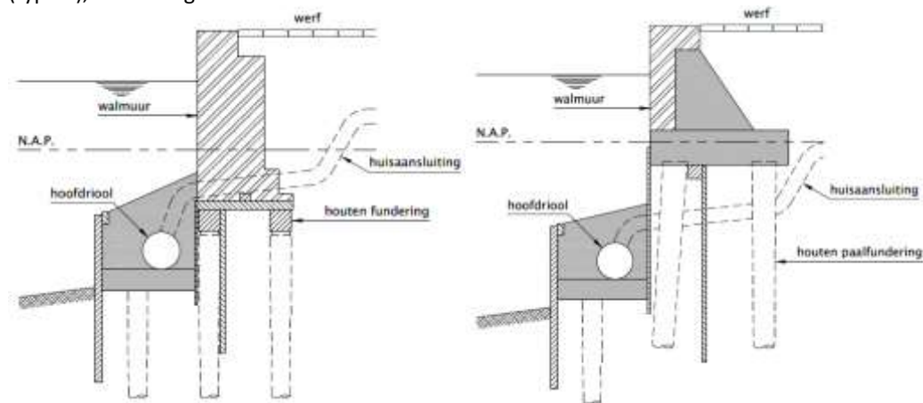
Figuur 7: Walmuur type 1 en 2 (uit Ontwerpnootie herstel lage walmuren)
