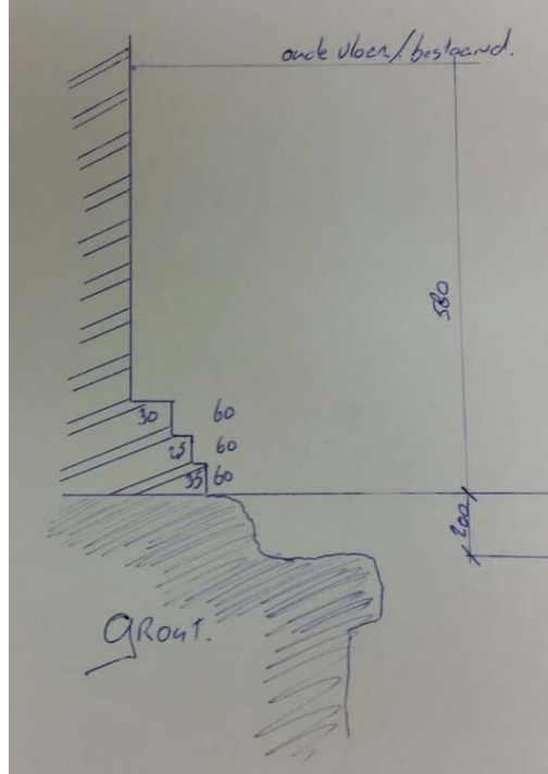
Figuur 49 – foto proefsleuf vrijgegraven groutpaal en schets opbouw fundering brugkelder
