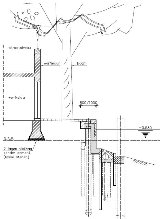
Figuur 10 – ontworpen bouwmethode palenwand (boomspecial)
