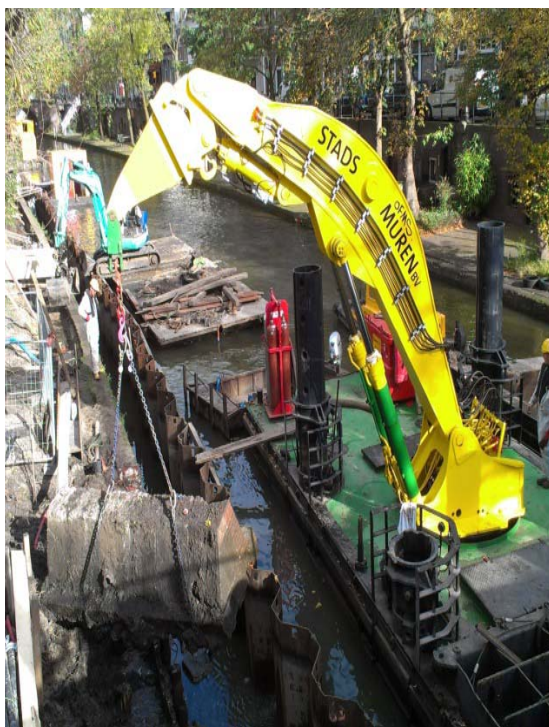
Figuur 39 – de walmuur wordt ontmanteld, vervolgens wordt tussen de oude houten funderingspalen een stalen damwand aangebracht: hier wordt de damwandmethode toegepast
