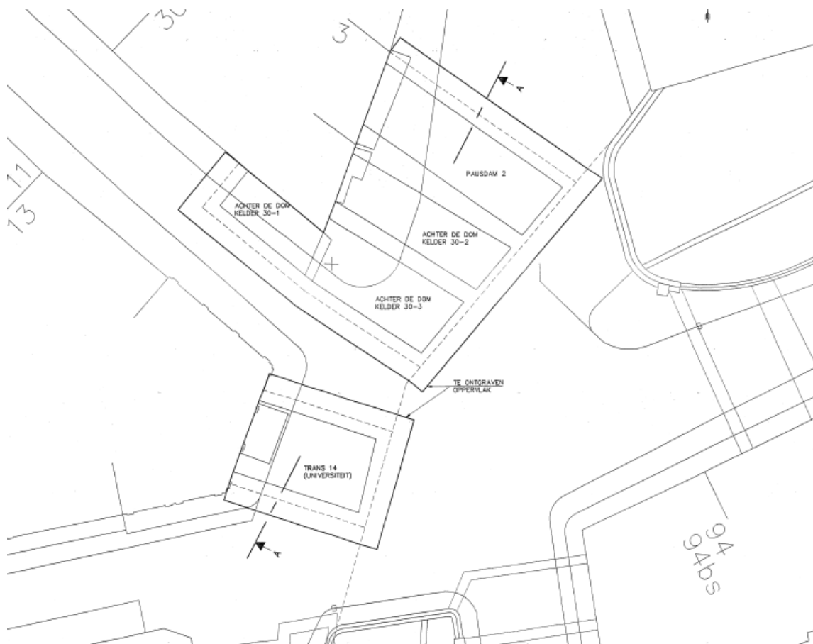
Figuur 13 – ter hoogte van de Pausdam zijn de pleinkelders die aansluiten op de Pausdambrug voorzien van een overkluizing om deze route bereikbaar te houden voor vrachtverkeer
