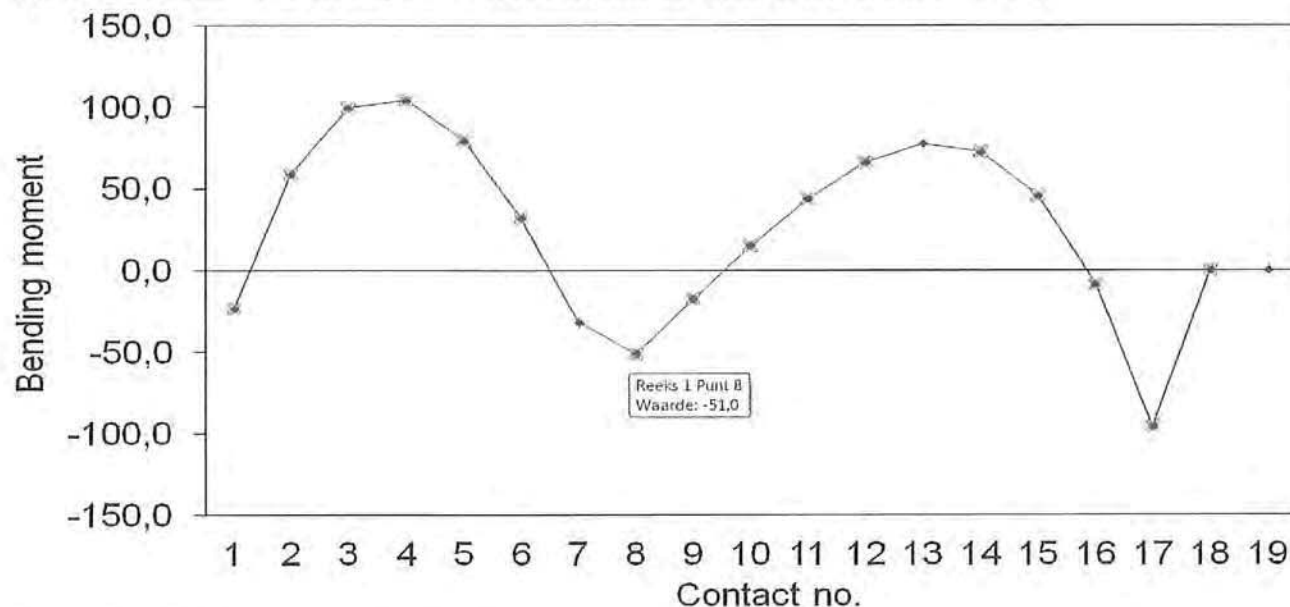
Figuur 2-8: uitvoer Excelsheet, momentelij
