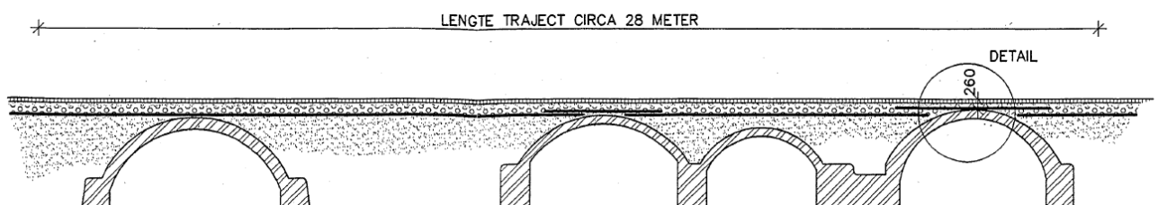
Figuur 14 – doorsnede van de overkluizing
