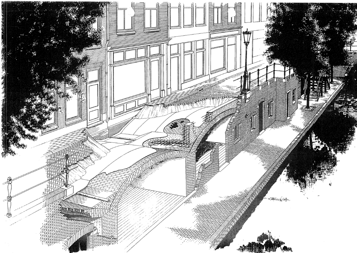
Figuur 30 – artist impression die is gemaakt om de werking van de L-wanden toe te lichten. Voor dit herstel is een samenwerkingsverband aangegaan tussen de private eigenaren en de gemeente in de Stichting Herstel Werfkelders die op 16 september 1993 is opgericht (acte SM14625 opgemaakt door Swane & Holtman notarissen te Utrecht)
