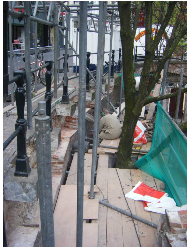
Foto 10 Verwijderen en herstel slecht metselwerk
