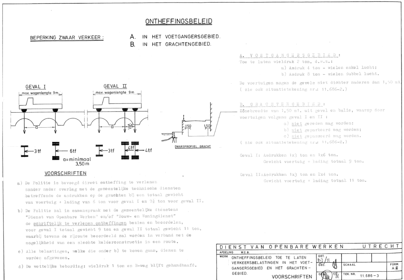
Figuur 64 – ontheffingsbeleid. In 1976 blijkt dat er een wioldruk van maximaal 1 ton werd gehanteerd, en is een voorstel aan B&W gezonden met voorstel om een ontheffingsbeleid vast te stellen waarbij de wioldruk van 1 ton (2 ton aslast) gehandhaafd bleef, maar via een ontheffing tot 2 ton kon worden verleend. Hiervoor kreeg de politie de bevoegdheid om in bepaalde gevallen direct ontheffingen te verlenen, en in andere gevallen in overleg met het toenmalige ingenieursbureau van de gemeente.
