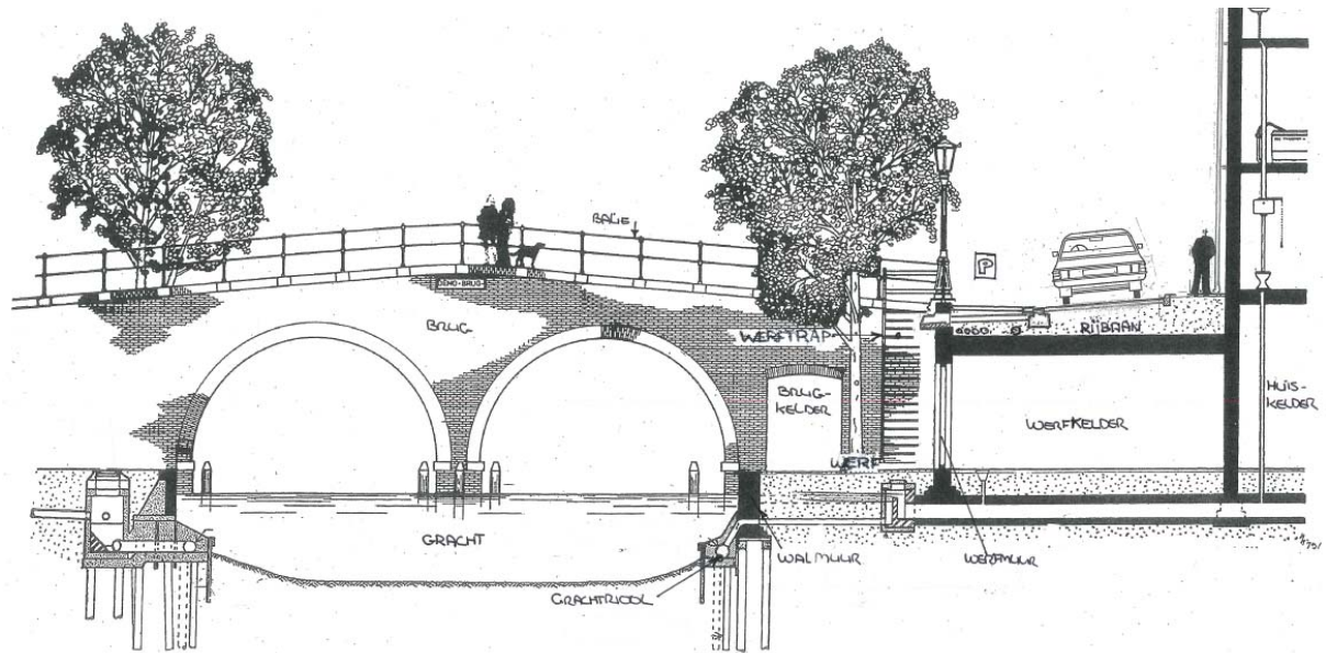
Figuur 1 – begrippen voor grachtprofiel met werf (walmuur, werfmuur, werfkelder en brugkelder)
