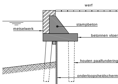
Afb. 6 Constructie uit de jaren 50 en 60
