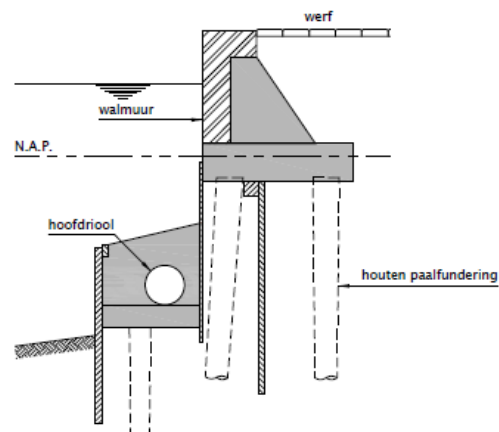
Principeddoorsnede bestaande situatie (type 2)
