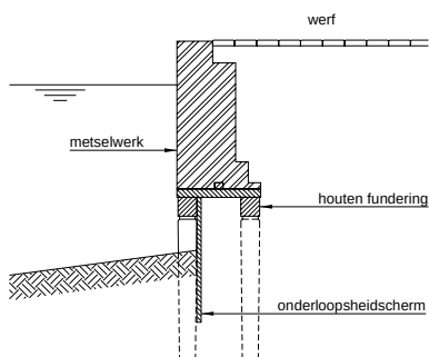
Afb. 4 Oorspronkelijke constructie
