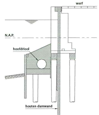
Nieuwe situatie met houten damwand
