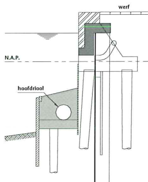
Nieuwe situatie met stalen damwand
