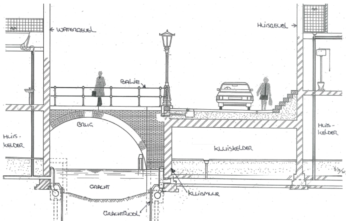
Figuur 2 – begrippen voor grachtprofiel zonder werf (kluismuur, kluiskelder & watergebonden woning met watergevel)
