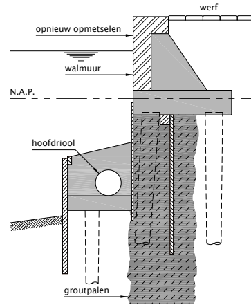
Nieuwe situatie met grootpaalwand (type 2)
