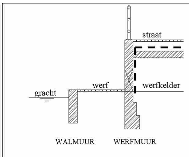
Afb. 1 overzicht wal- en werfmuur
