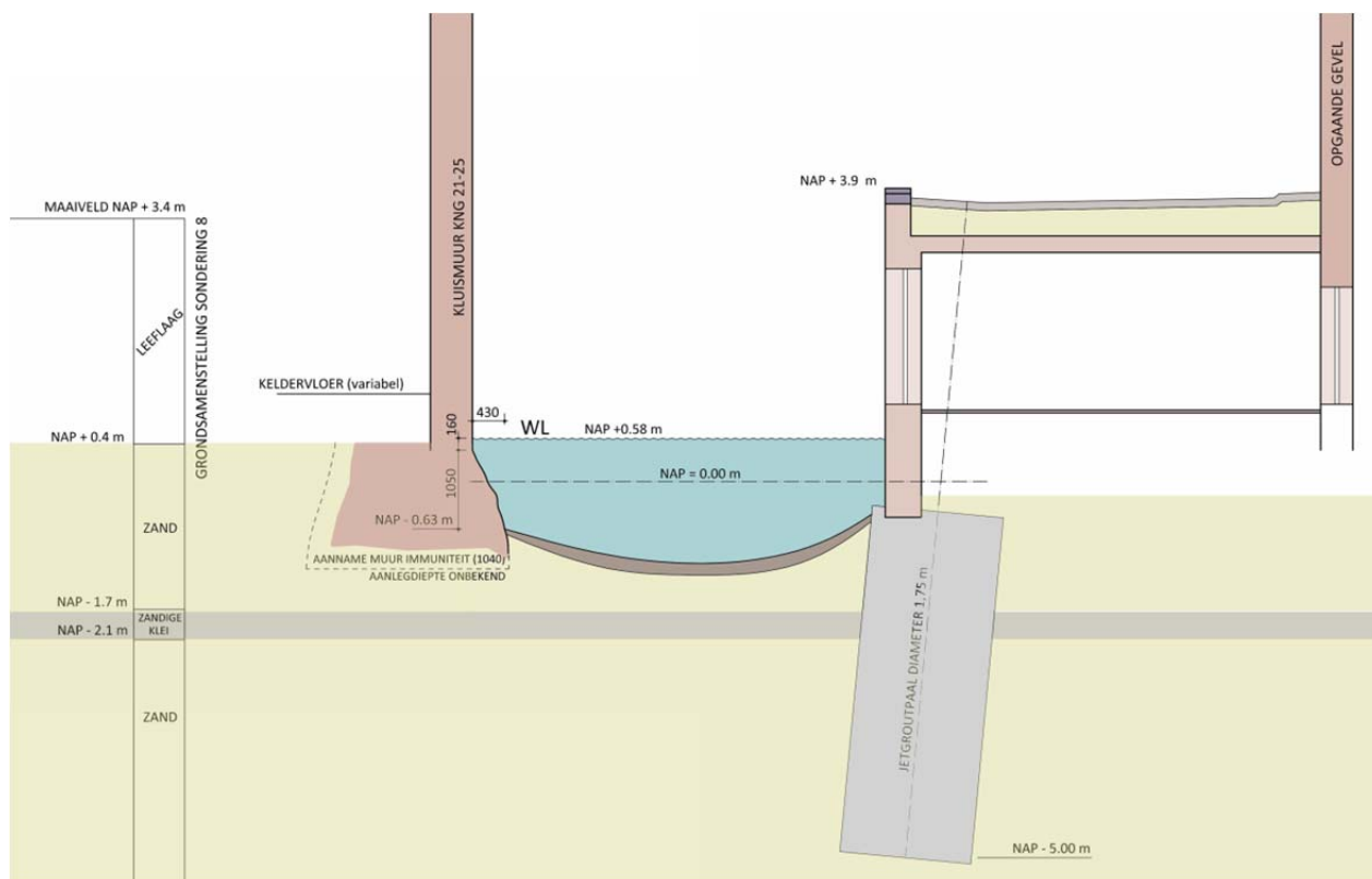
Figuur 9 – schema renovatie (in dit geval de Kromme Nieuwegracht) en invloed op grondwaterstromen
