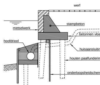
Afb. 7 Constructie uit de jaren 50 en 60 met rioolkoffer uit de jaren 80
