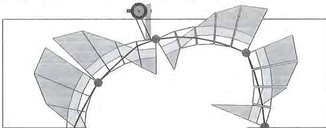
Figuur 2-5: uitvoer RING, moment in contactvlak 50,5 kNm (50481 KNmm)
