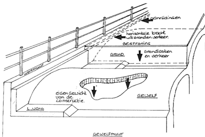
Figuur 31 – schematisatie krachtwerving
