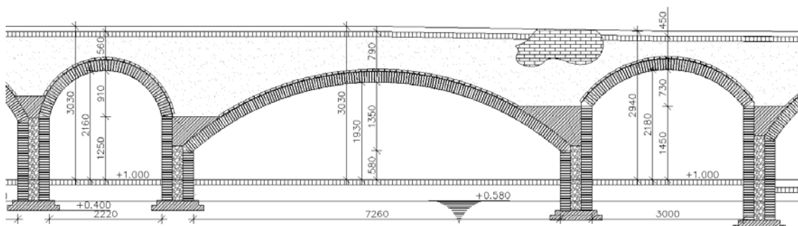
Figuur 5 - drie maatgevende kelders naast elkaar, de smalste, de breedste (OG #1#) en een gemiddelde
