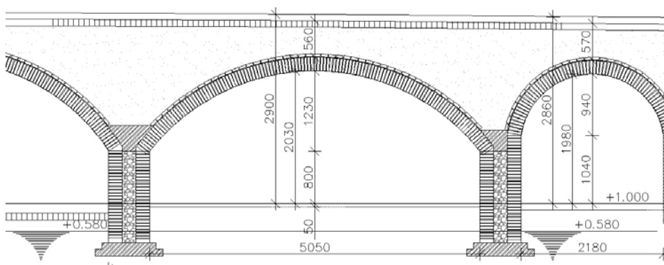
Figuur 6 - een gemiddelde maat kelder (OG#2#).
