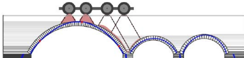
Figuur 10 – rekenmodel kelder OG #3#
