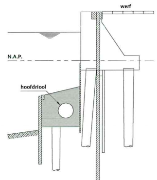
Nieuwe situatie met houten damwand
