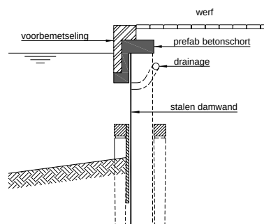
Afb. 9 Oplossing zonder rioolkoffer
