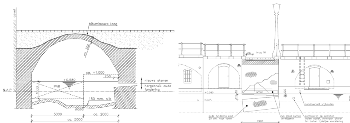
Figuur 56 – reconstructie schade fundering Kromme Nieuwegrachtbrug 07; In 2018 kwam naar voren dat de gehele fundering van de toegangsbrug naar woonhuis Kromme Nieuwegracht 7 onder de brug was weggezakt, net buiten het zicht (ca. 1 strek onder grachtpeil). Bij eerdere duikonderzoeken werd de fundering van deze toegangsbrug niet aangetroffen en werd geen schade aan de brugfundering geconstateerd, maar deze schade geeft aan dat het bruggenhoofd op staal is gefundeerd. Dergelijke schades worden in de literatuur gelinkt aan erosie. Dit mechanisme is mogelijk door beperkte graafwerkzaamheden bij het duikonderzoek om de funderingsopbouw te bepalen versneld. Deze schade geeft aan dat de funderingen relatief ondiep zijn gefundeerd en gevoelig zijn voor ontgroningen. Hetzelfde zou gesteld kunnen worden voor de kluisuren die op de middeleeuwse fundering zijn herbouwd.
