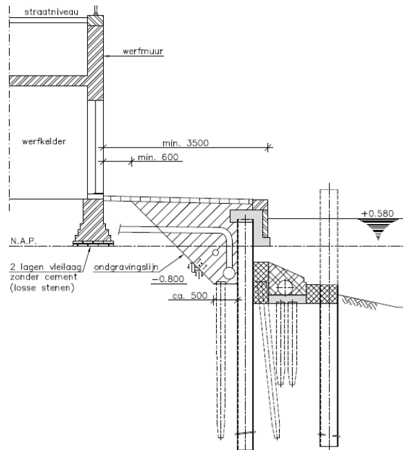
Figuur 14 – uitvoeringsmethode Oudegracht met invloedsgebied
