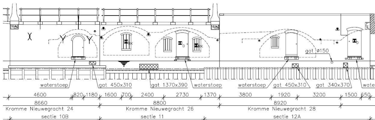
Figuur 57 – reconstructie aanzicht kluisuren Kromme Nieuwegracht 24, 26 en 28. Dit aanzicht is samengesteld uit duikonderzoek, geveltekeningen uit de '90-er jaren van de kluisuren per adres, inmeting rollaag en spuwers. De kelderprofielen zijn samengesteld uit uitslagen (globale inmeting + schadepatroon binnenzijde kelder) die voor het project waterdicht maken kelders zijn gemaakt en zijn gecombineerd met schetsen van de meetdienst van de bovenzijde. Het dikteverloop van het gewelf is een resultaat van meetfouten! Bij sommige gevelhersteltekeningen is ook het keldergewelf getekend en dan ook in deze tekening verwerkt. Op dit aanzicht aan de rechterzijde een kluisuur met een gemetselde muur, de borstwering , terwijl links de meer reguliere balie aanwezig is. Voor de deuren van de kluisuren zijn de waterstoepen aanwezig. Tussen beide kelders van Kromme Nieuwegracht 26 is een zeer grote uitsparing in de wand aanwezig van 1,37 meter breed. Aangenomen wordt dat dit een waterafvoer van het achterland is, de zogenaamde slokop .
