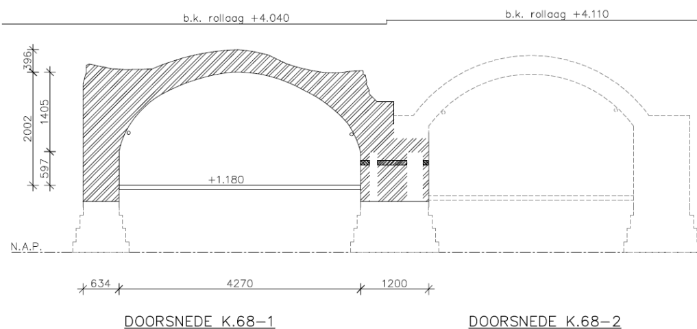
Figuur 53 – reconstructie kelder KNG 68 en KNG 70 t.b.v. herbouw gedeelte kelder KNG 68. Uit een horizontale kernboring blijken de scheidingswanden dun uitgevoerd \frac{1}{2} tot 1 steens met een spouw. Daartussen is echter massief metselwerk aanwezig, een opbouw die ons voor raadsels stelt.
