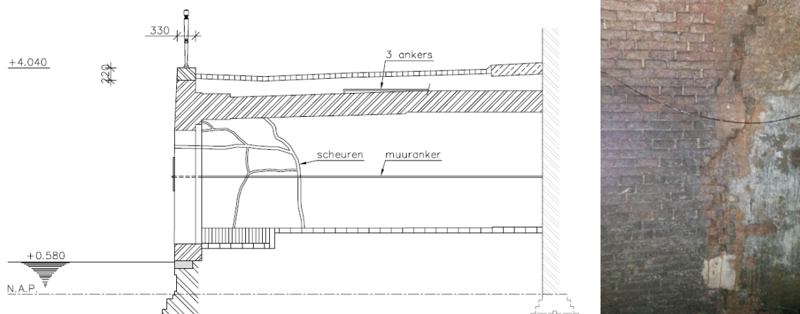
Figuur 54 – reconstructie schadepatroon bij kluiskelder Kromme Nieuwegracht 68 (links) en foto detail van schade KNG 64 in zuidwand. De schade bij kelder 68 was voor start van de renovatie reeds aanwezig. Door het aanbrengen van een plat damwandprofiel als blow-out protectie bezweek de fundering geheel waardoor de voorzijde herbouwd zal moeten worden. Dit schadepatroon is niet uniek, en werd ook aangetroffen bij de kluiskelder van Kromme Nieuwegracht 64, die overigens met de nodige moeite succesvol een nieuwe fundering heeft gekregen en momenteel gerenoveerd wordt. In kelder 68 is aan beide zijde een doorlopend anker in de geboorte aangebracht, het kelderanker . Daarnaast zijn aan de bovenzijde van de kelder 3 gewelfankers aangebracht die aan de bovenzijde van de boog zijn aangebracht en richting de woning zijn verankerd, wat opmerkelijk genoemd mag worden. Zie ook Figuur 52. Dergelijke ankers zullen in het verleden zijn toegepast als herstelmaatregel.
