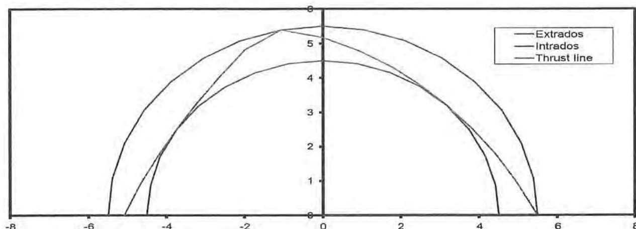
Figuur 2-8: uitvoer Excelsheet, momentelij
