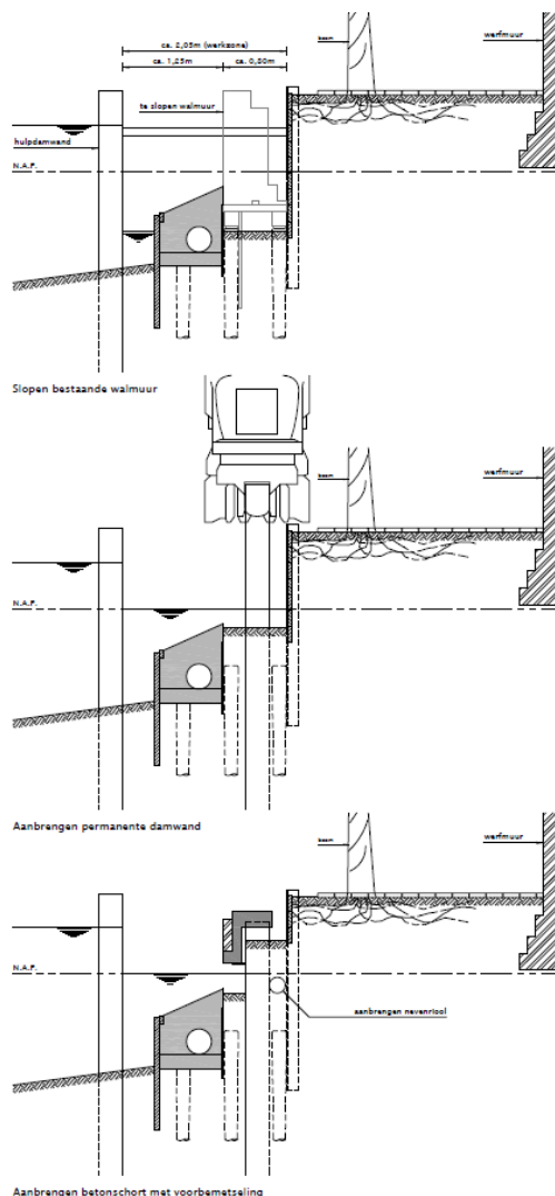
Figuur 8 – ontwerp-bouwfasering vervangen walmuren Oudegracht
