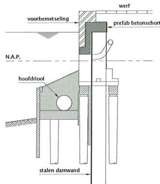
Nieuwe situatie met stalen damwand
