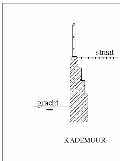
Afb. 2 overzicht kademuur
