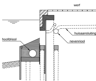
Afb. 8 Oplossing tpv rioolkoffer
