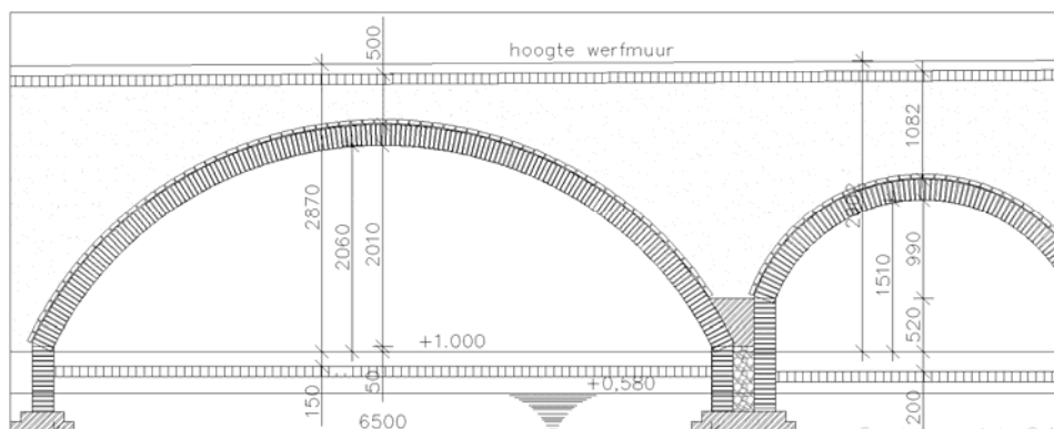
Figuur 7 - een brede kelder met een groot pijl (OG #3#).
