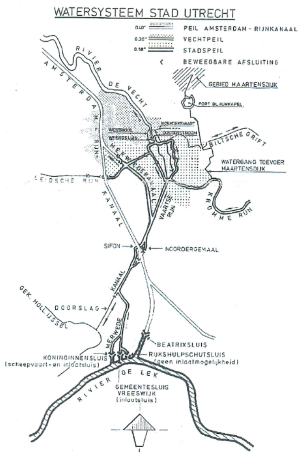
Figuur 4 – hoofdstructuur watersysteem stad Utrecht
