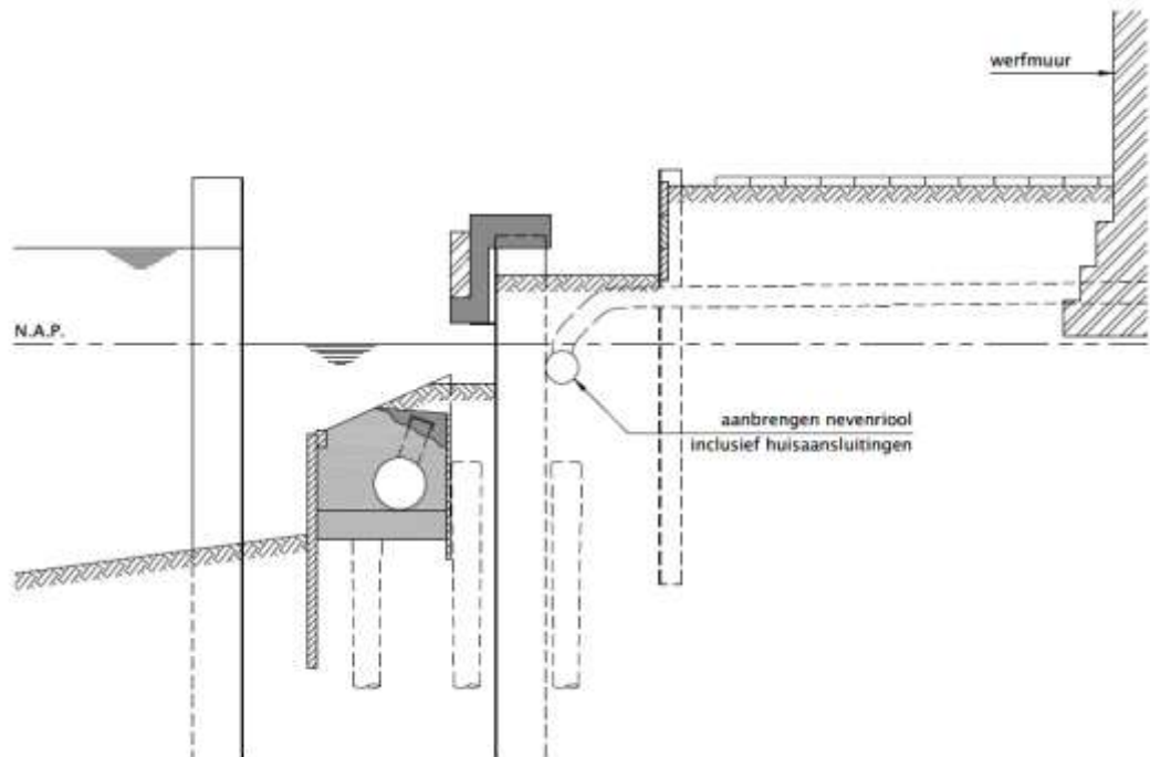
Figuur 8: Damwandmethode (afbeelding uit Ontwerpnootie herstel lage walmuren)
