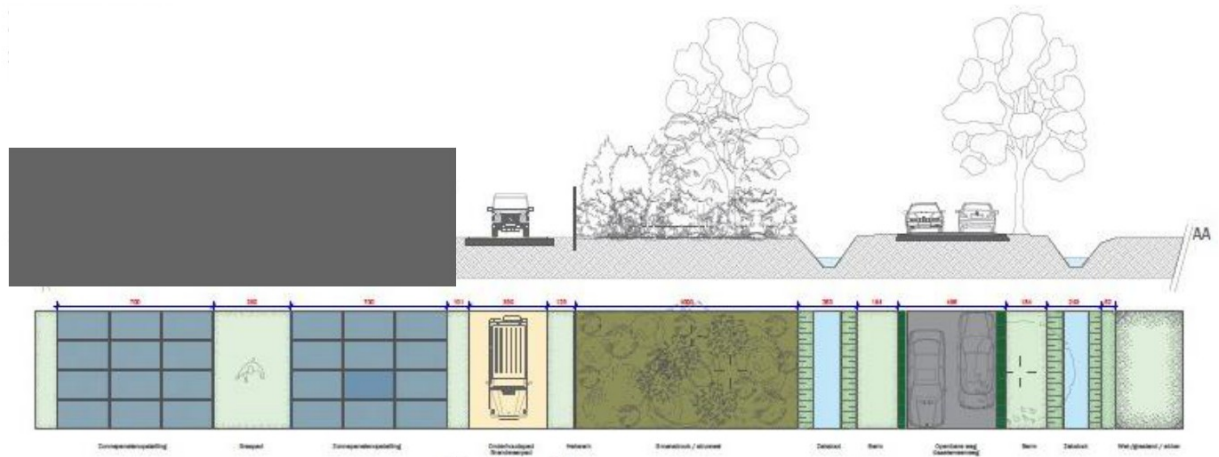
Afbeelding 39; Doorsnede A - AA (ruimtelijkheid langs openbare weg, Usselerveenweg) (dd. 28-11-2024)
