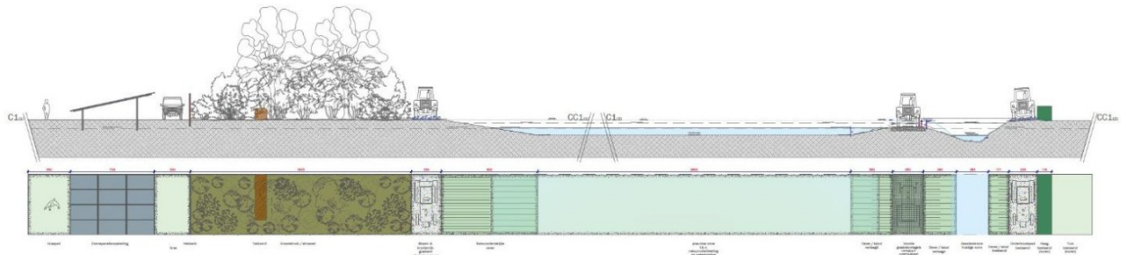
Afbeelding 54; Doorsnede C1(1) – CC1(1) + C1(2) – CC1(2) (ruimtelijkheid tussenzone / rond Usselerstroom) (dd. 28-11-2024)
