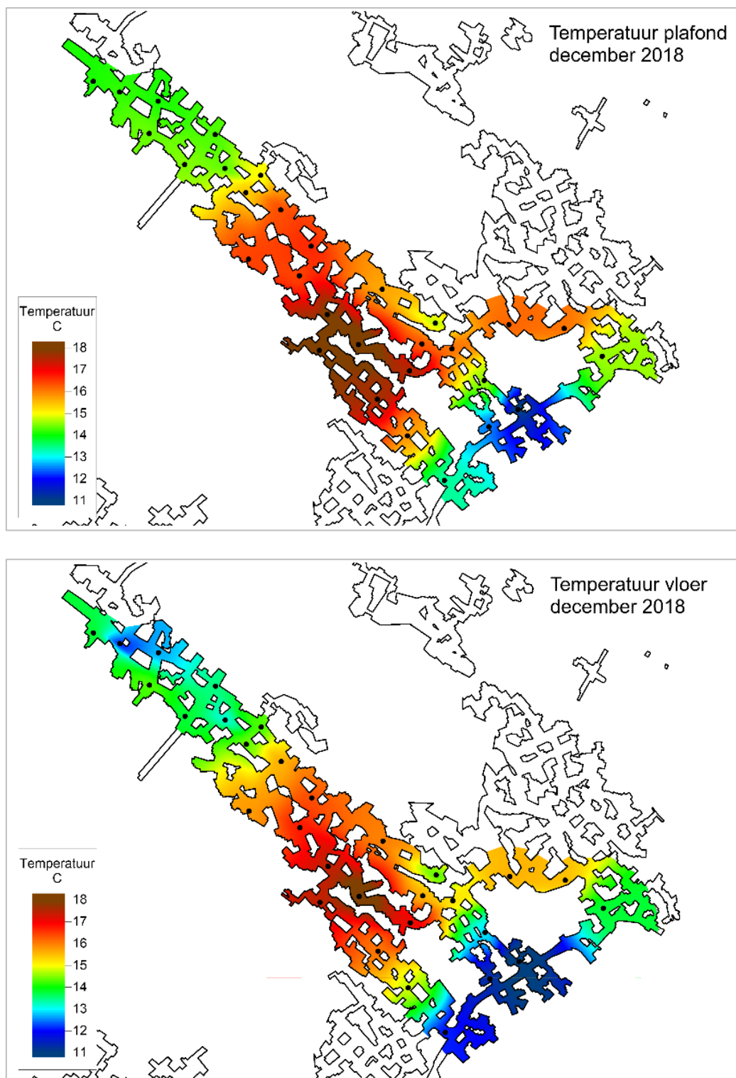
Figuur 32 IR-temperatuurmetingen in Kerstmarkt in december 2018.
