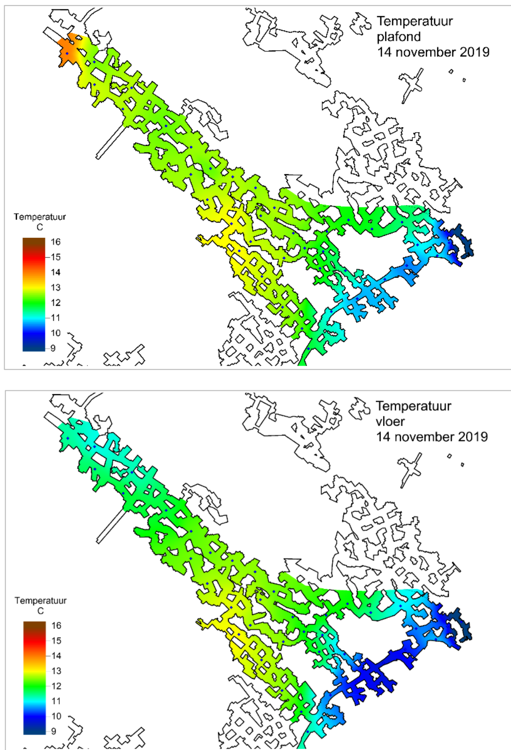
Figuur 33 IR-temperatuurmetingen in Kerstmarkt begin november 2019.
