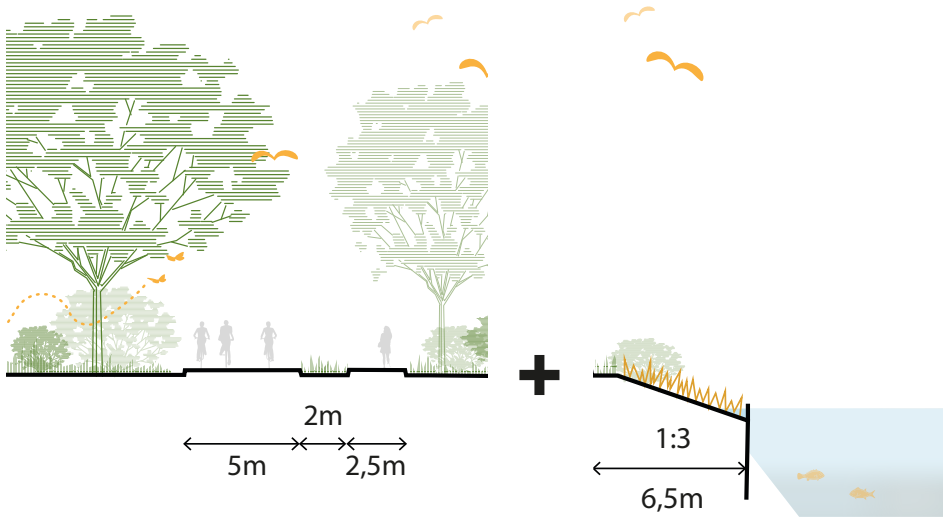
Principeprofiel basis: vrij liggende paden met smalle middenberm + plasdrasberm
