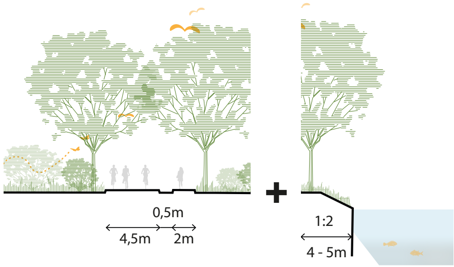
Principeprofiel smal: gecombineerde paden + smalle oever
