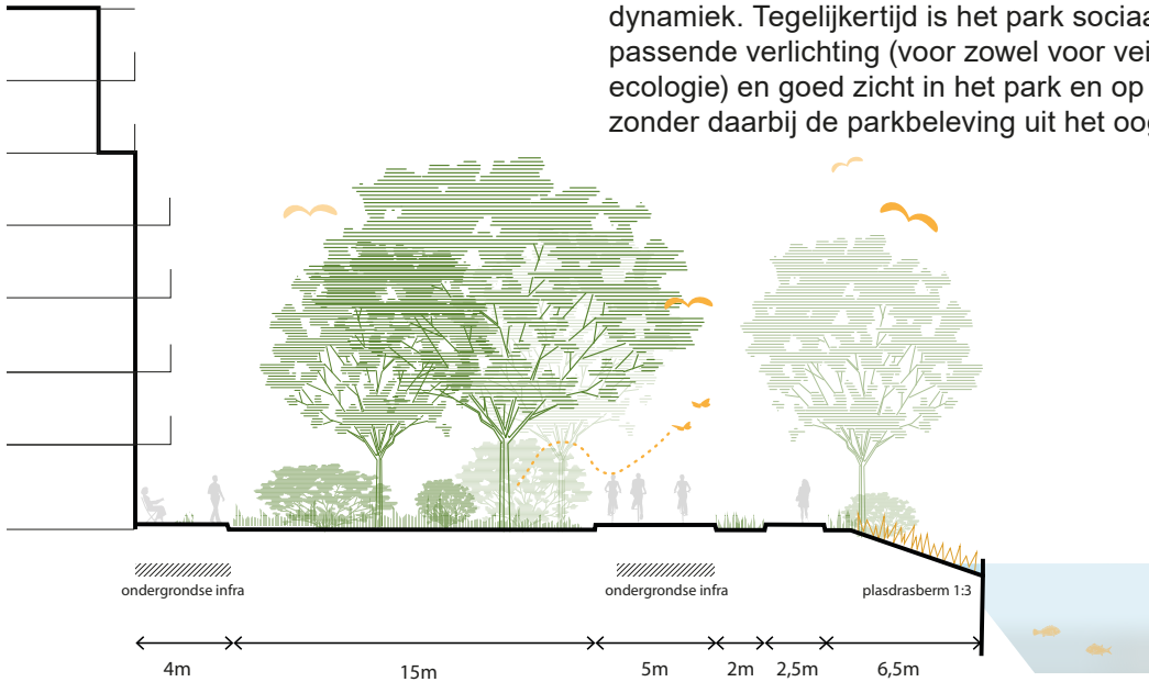
Vrij liggend fiets- en wandelpad gescheiden door een groenstrook met een plasdrasberm
