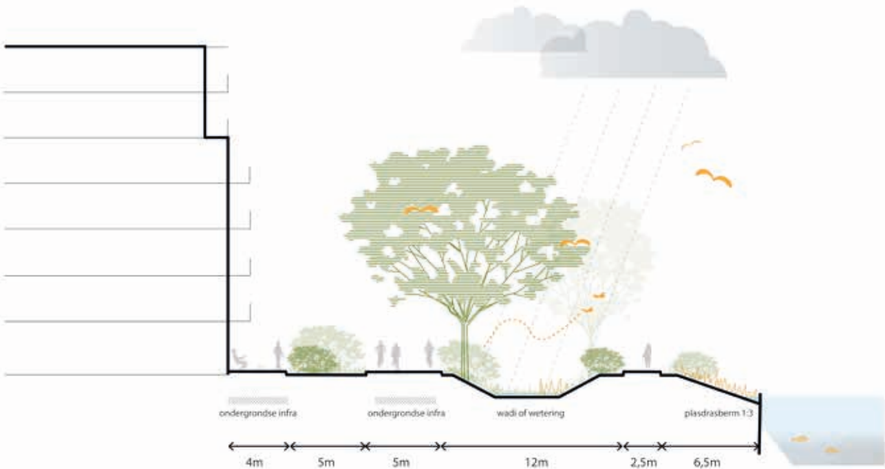
Vrij liggend fiets- en wandelpad gescheiden door een groenstrook met een plasdrasberm
