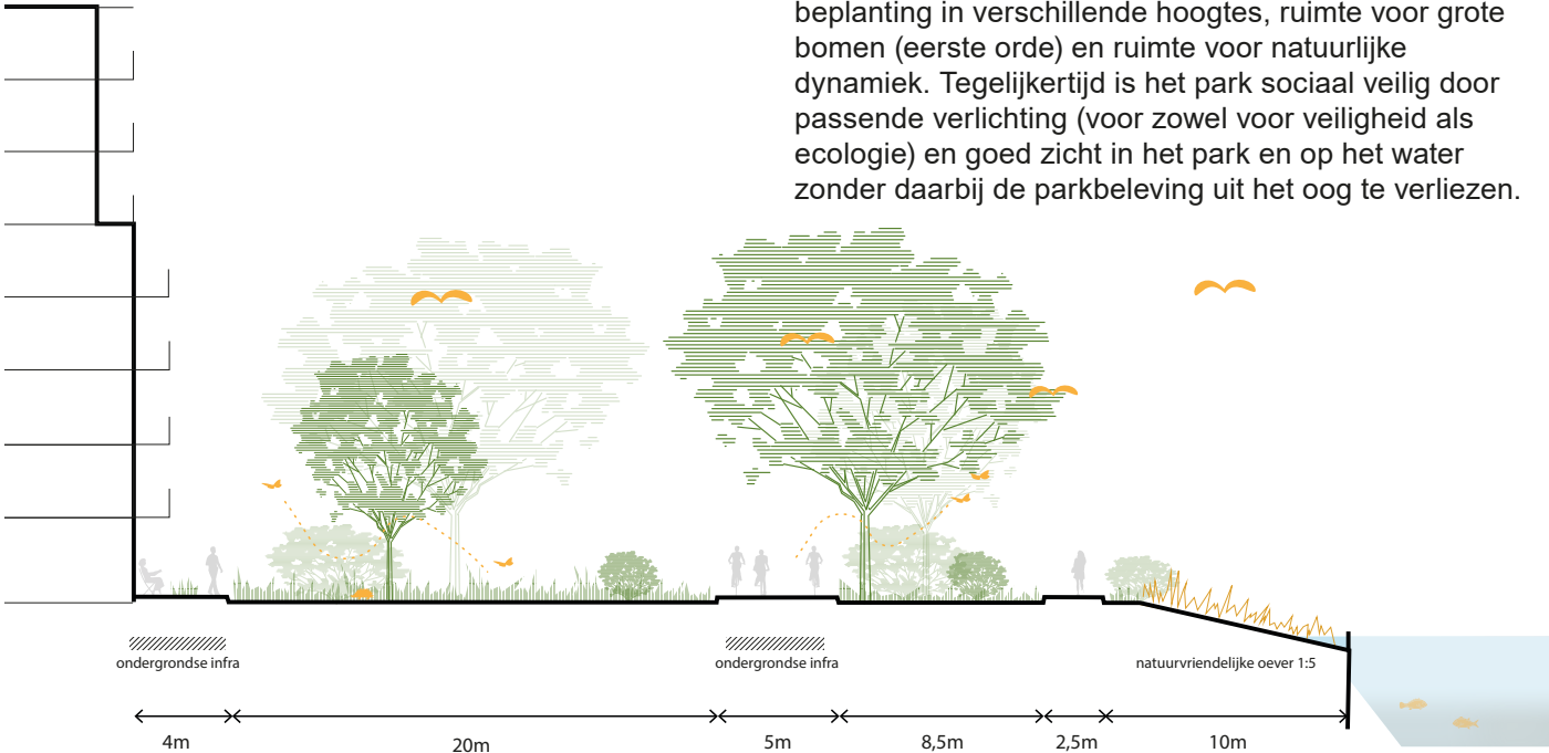
Vrij liggend fiets- en wandelpad gescheiden door een brede groenstrook met een ecologische oever
