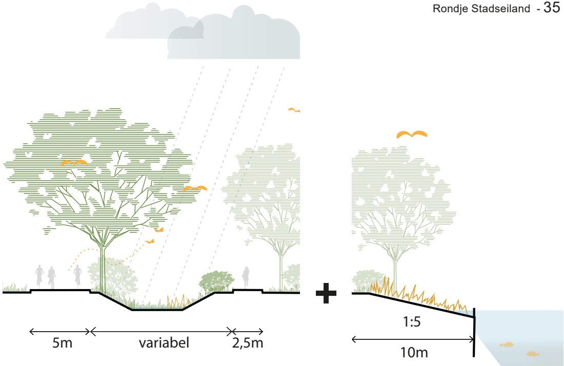
Principeprofiel pocket park: vrij liggende paden met brede middenberm + ecologische oever
