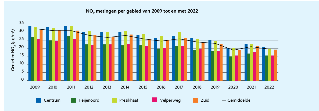
Figuur 3 NO 2 metingen per gebied van 2009 tot 2022
