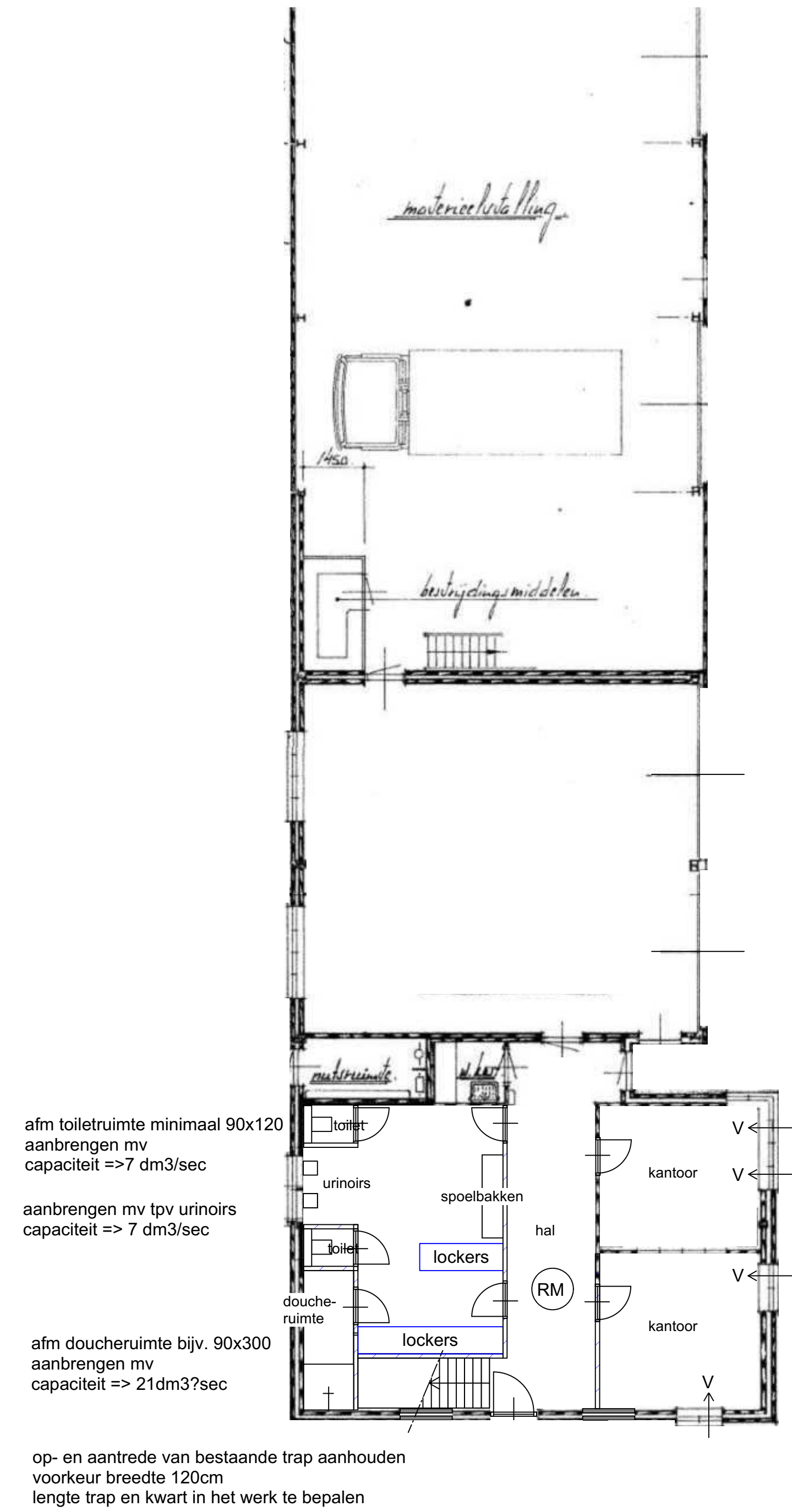
GEWIJZIGDE SITUATIE BEGANE GROND
