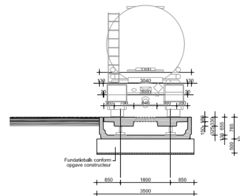
Dwarsdoorsnede
