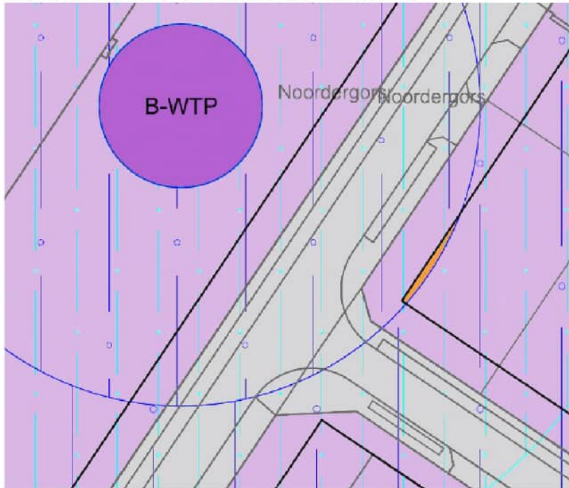
Figuur 5.7 Illustratie overlap PR10^{-05} contour van 55 meter met het bouwvlak (in oranje de overlap)
