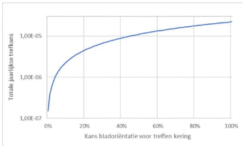
Figuur 5.16 Kans van kritieke bladoriëntatie waarbij de Maeslantkering kan worden getroffen bij mastfalen uitgezet tegenover de jaarlijkse resulterende totale trefkans van de Maeslantkering
