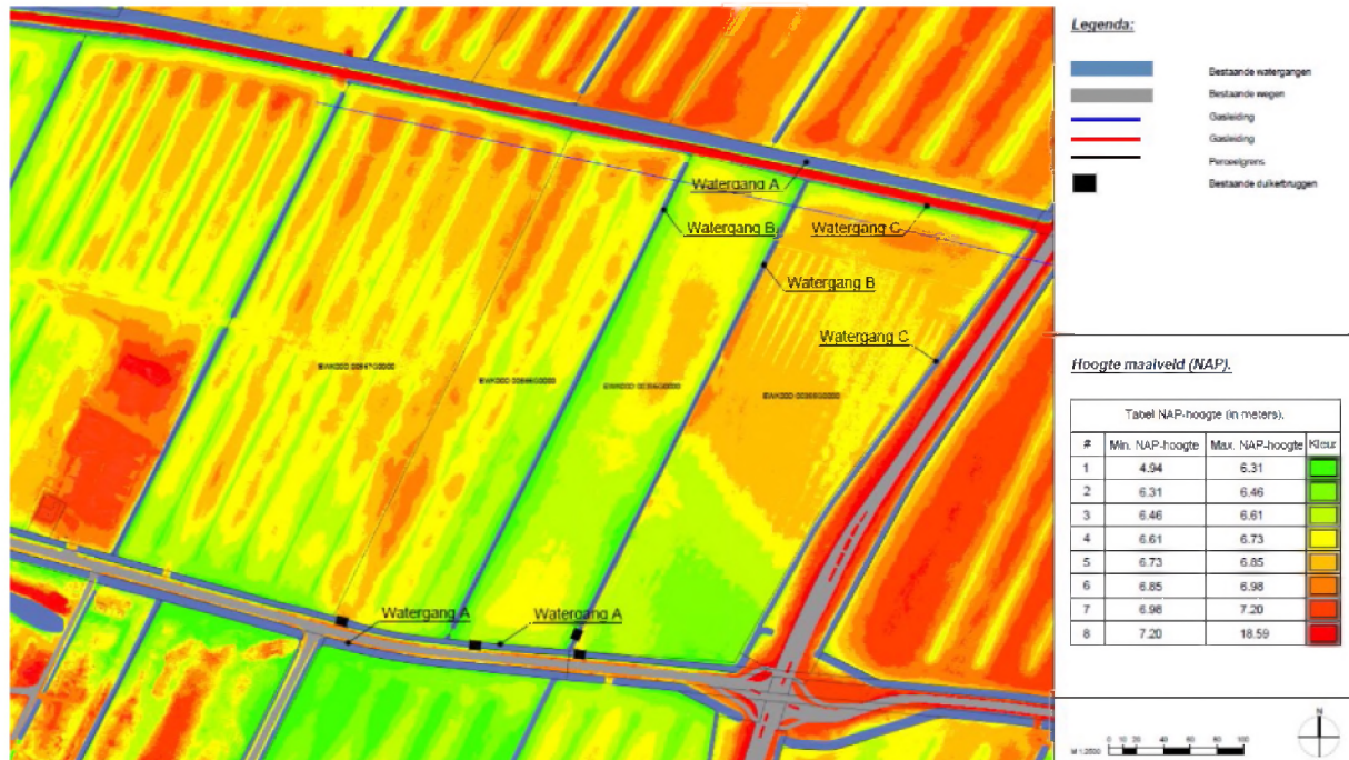
FIGUUR 6: TECHNISCHE TEKENING HUIDIGE PERCELEN MET DE MAAIVELHOOGTE (NAP HOOGTE), BESTAANDE DUIKERS, WATERGANGEN, PERCEELGRENZEN EN PERCEELNUMMERS. VOOR EEN GEDETAILLEERDE WEERGAVE ZIE BIJLAGE XI: TECHNISCHE TEKENING HUIDIGE PERCELEN.
