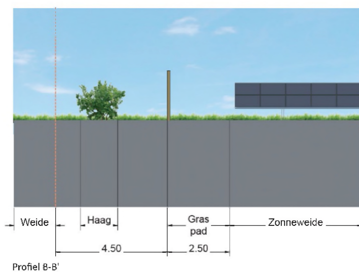
FIGUUR 10: DOORSNEDE B-B' BEOOGD ZONNEPARK SCHOENAKER, VANAF WESTZIJDE, VOOR LOCATIE ZIE FIGUUR 8. BRON: LABELTIEN
