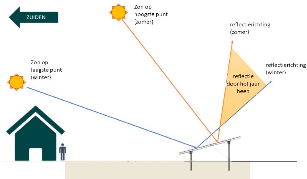
FIGUUR 30: LICHTWEERKAATSING OP ZONNEPANELEN
