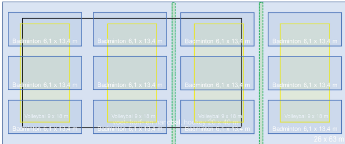
Figuur 3 Principe indeling velden in sporthal 63 x 26 x 7 (groen zijn scheidingswanden)
