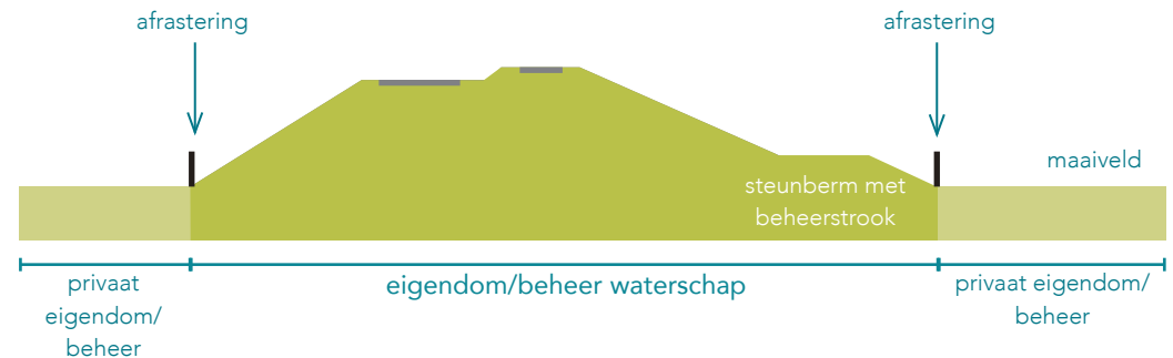
dijk met tuimelkade
