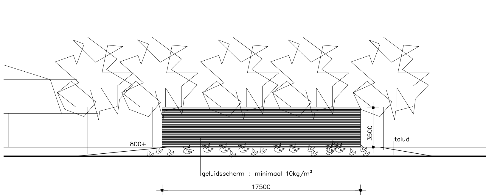
Principe aanzicht
