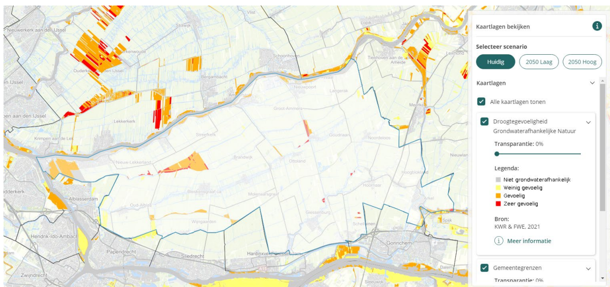
Risicogebieden ten tijde van extreme droogte. KWR & PWE, 2021. Klimaateffectenatlas
