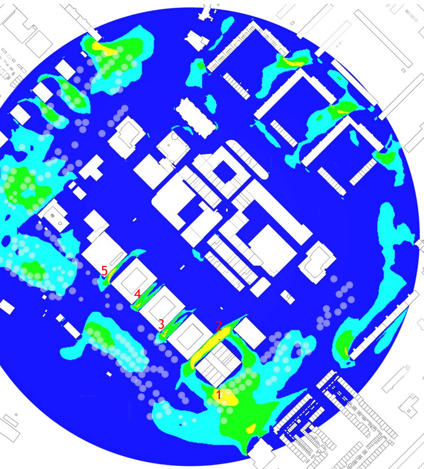
figuur 6: beoordeling windgevaar op maaiveld
