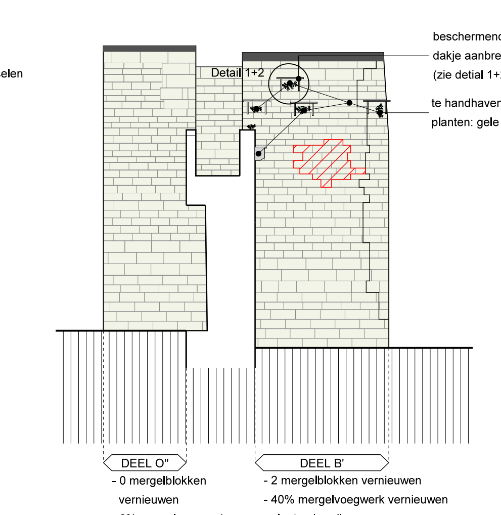
DOORSNEDE D-D (zijgevel vierkante toren)
