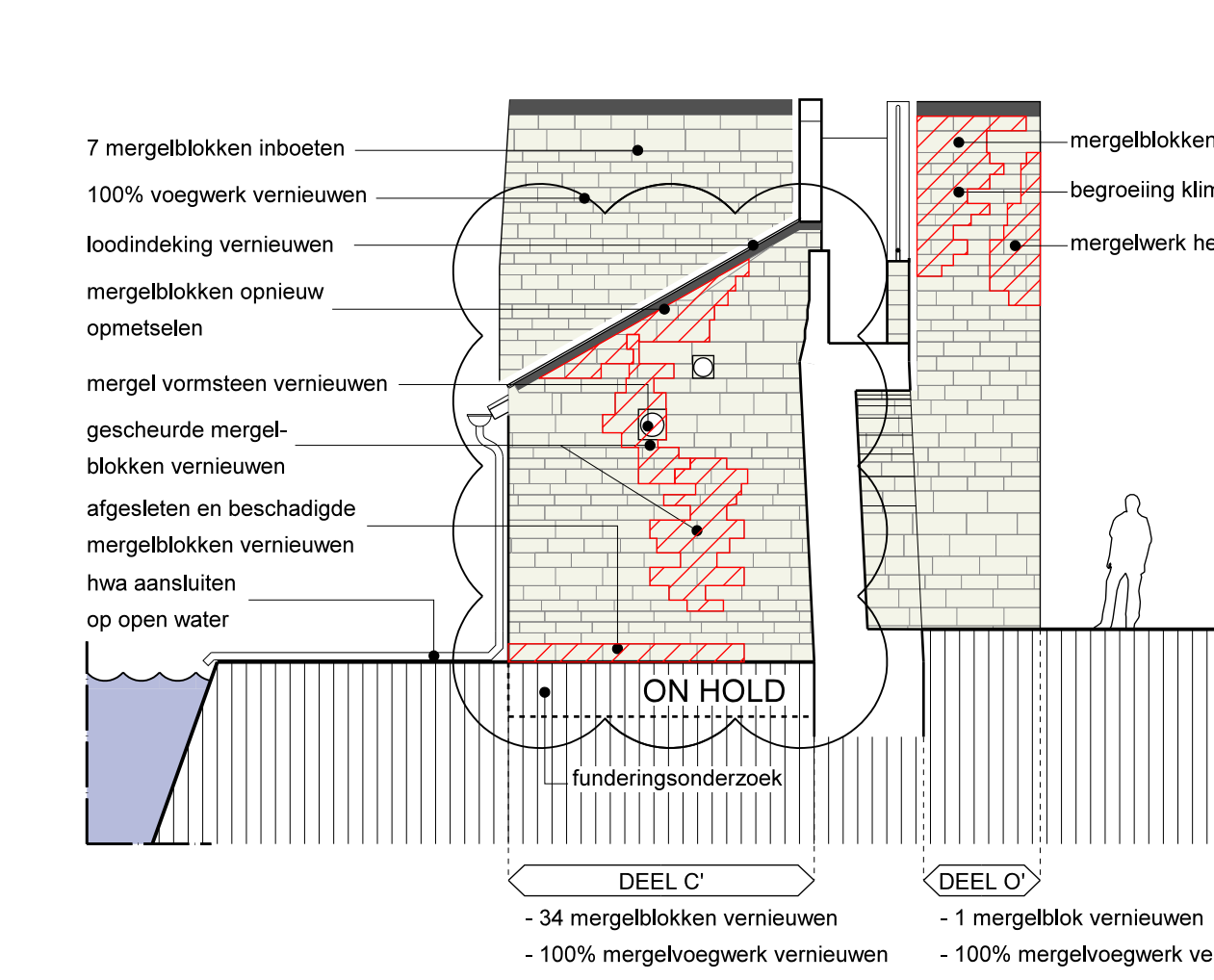
DOORSNEDE C-C (zijgevel kruithuis)
