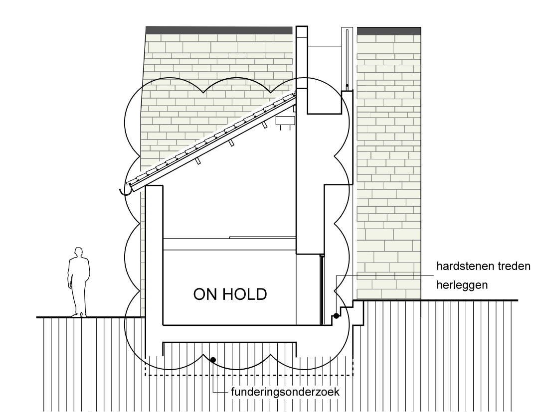
DOORSNEDE B-B
