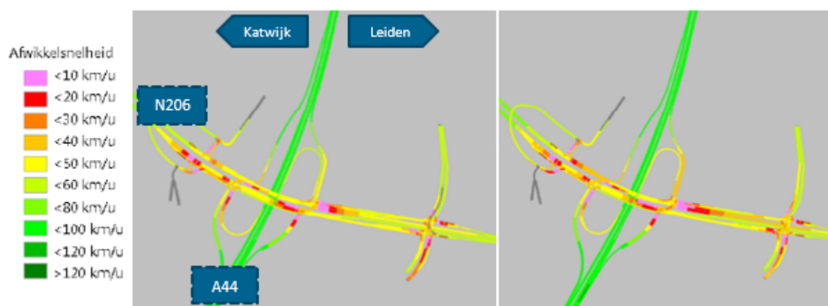
Figuur 5.2.13.4 Afwikkelingsnelheden op de knoop Leiden-West in de ochtendspits (links) en de avondspits (rechts) met de ontwikkeling van het 'Herstelbesluit Woongebied Valkenhorst'
