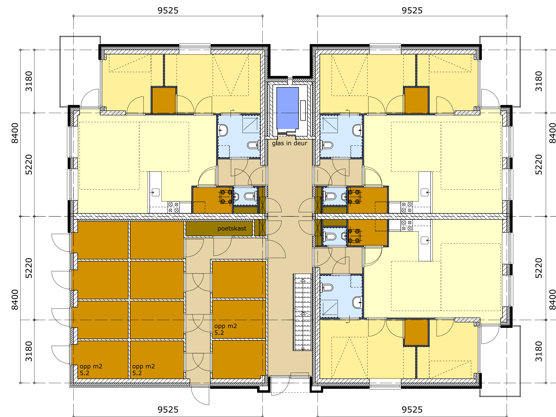
begane grond 3 appartementen/ 11 bergingen/ portiekontsluiting
