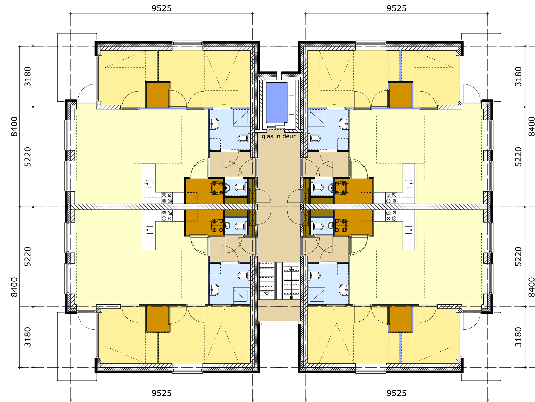
1e verdieping/ 4 appartementen 70m2 gbo.
