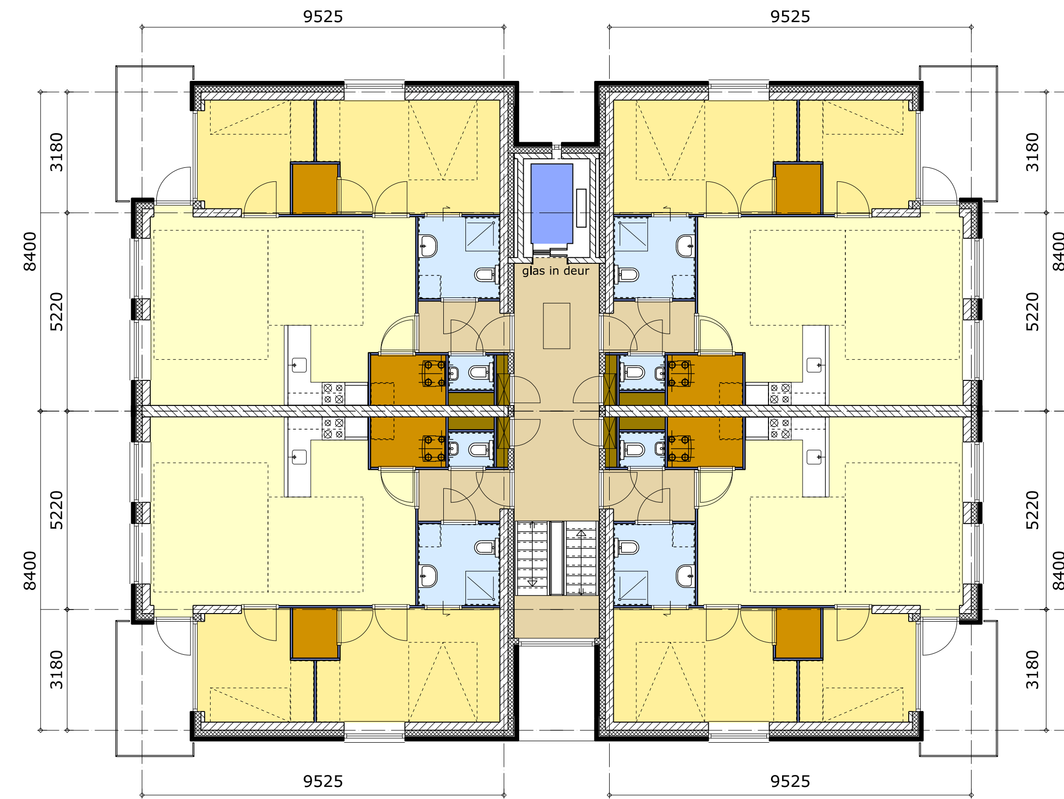
2e verdieping/ 4 appartementen 70m2 gbo.
