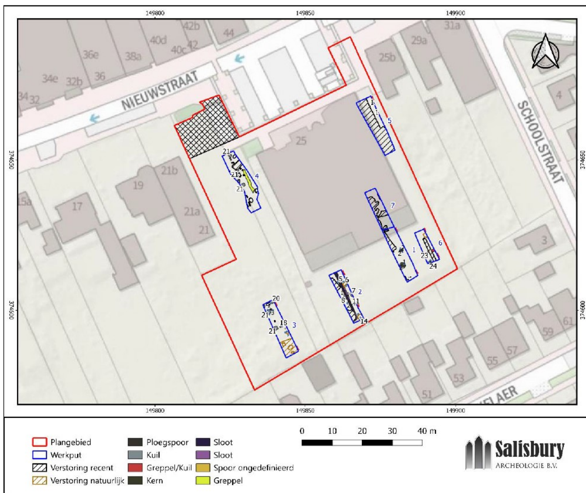
Overzichtskartaal van de aangelegde proefsleuven met sporen bij de Nieuwstraat 25 in Eersel (uit rapport Salisbury).
