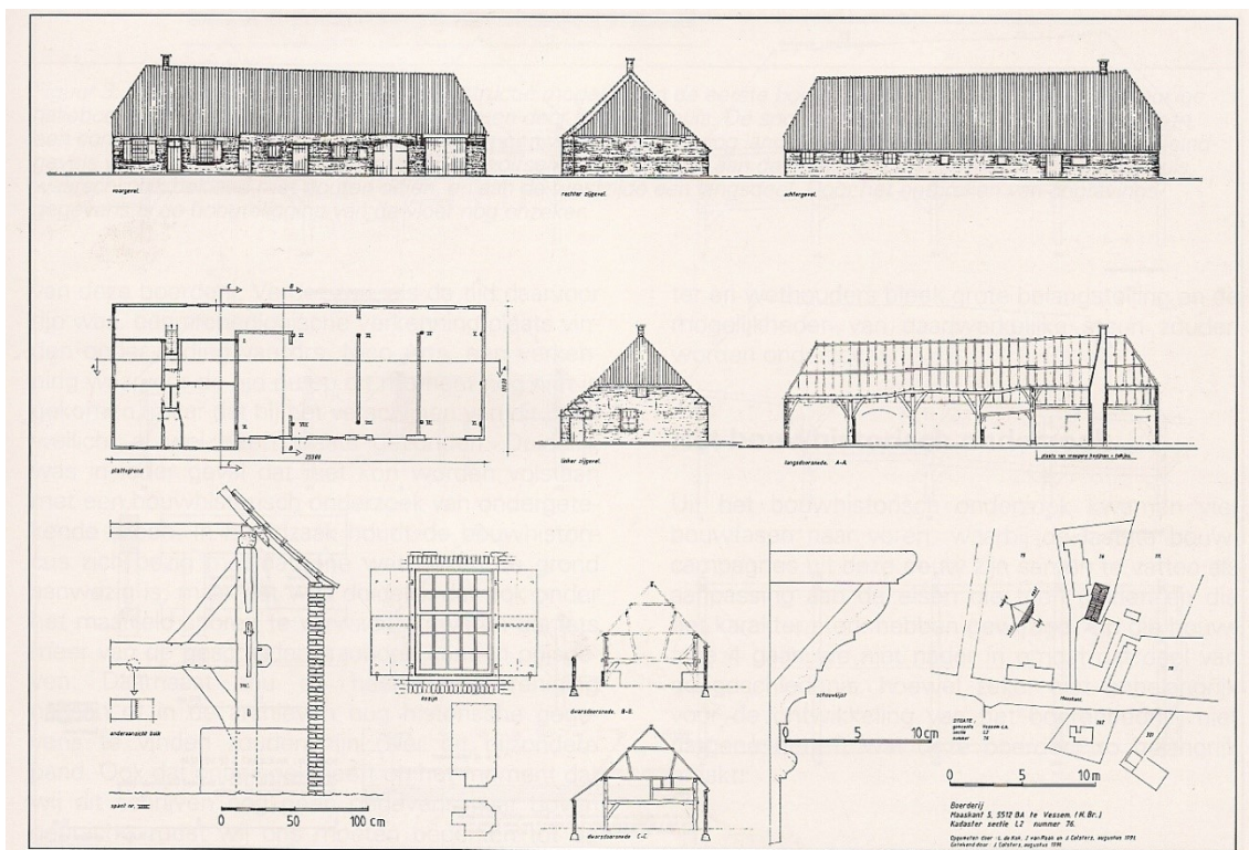
Opmetingen van de boerderij Maaskant 5 in 1991. BIGGELAAR 1993.
