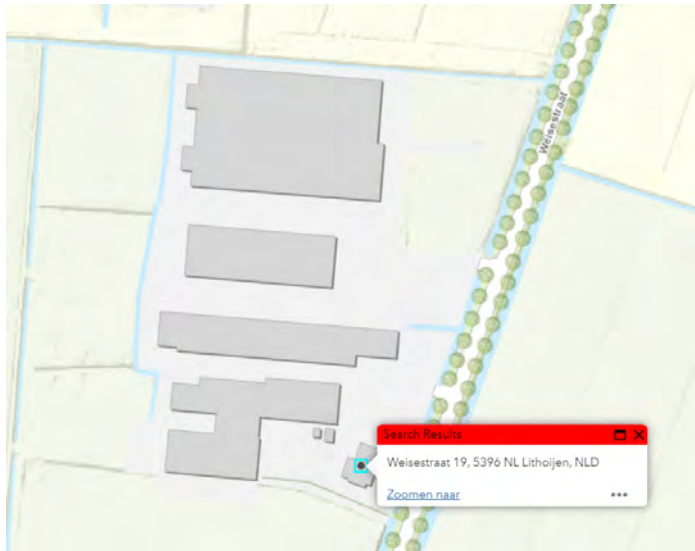
Uitsnede kaart aardkundig waardevolle gebieden.
