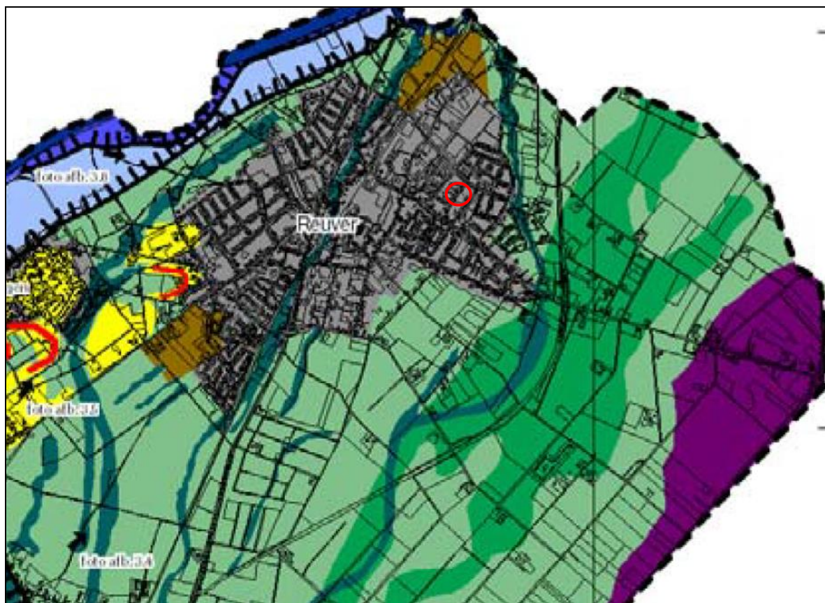
Figuur 3: Detail van de terrassenkaart binnen de gemeente Beesel. Het plangebied is aangegeven met de rode cirkel. Het Pleniglaciaal terras is in lichtgroen aangegeven met de restgeulen in een blauwgroene kleur. In geel de rivierduinen en in bruin de aanwezige enkeerdgronden (Bron: ADC Heritage 2010, 21).
